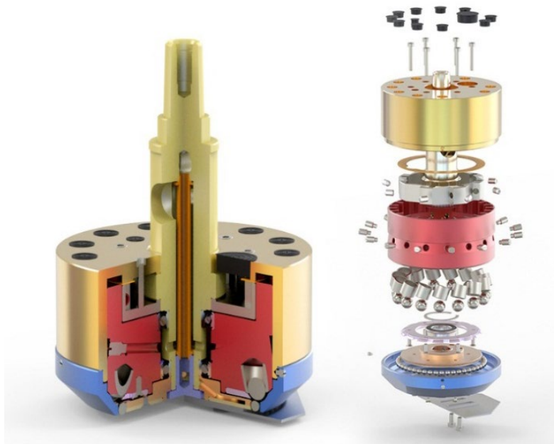
Рисунок 3 – Визуализация процесса сборки инструмента
