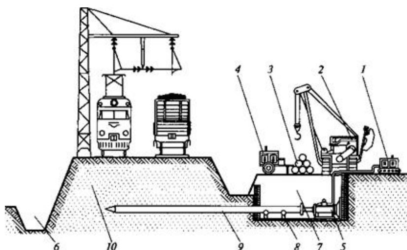
1 – гидронасос домкрата; 2 – автокран; 3 – трубы; 4 – сварочный агрегат; 5 – гидродомкрат; 6 – приемный котлован; 7 – рабочий котлован; 8 – направляющие; 9 – прокалывающая труба; 10 – железнодорожная насыпь
