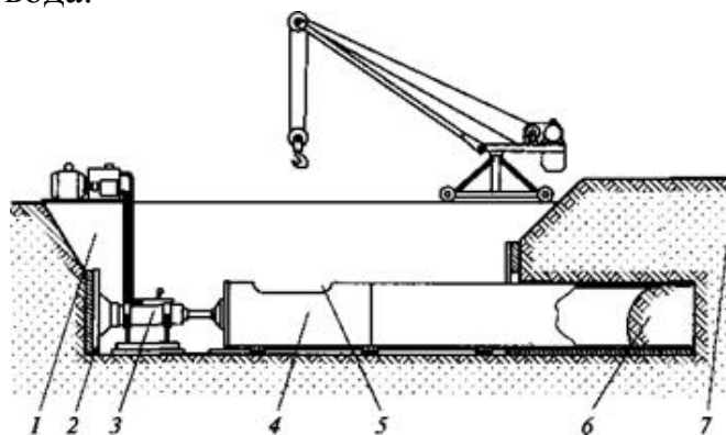
1 – рабочий котлован; 2 – упорная стенка; 3 – гидродомкрат; 4 – продавливающая труба; 5 – окно для выемки керна; 6 – керн; 7 – насыпь Рисунок 2 - Схема прокладки труб способом статического продавливания
