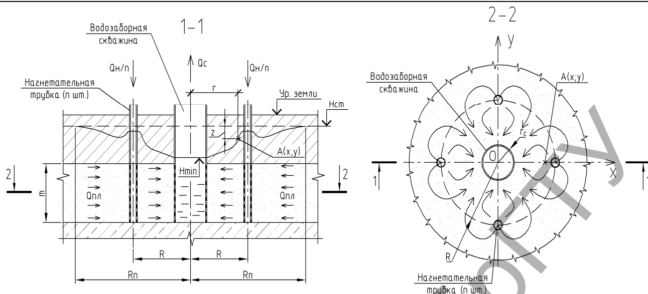
Рисунок 1 – Расчетная схема зафильтровой промывки водозаборной скважины в напорном пласте
