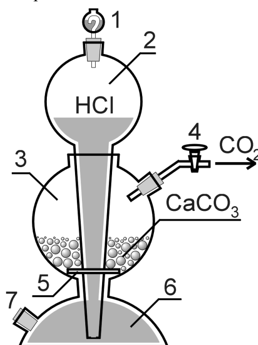
Рисунок 2 – Аппарат Киппа
