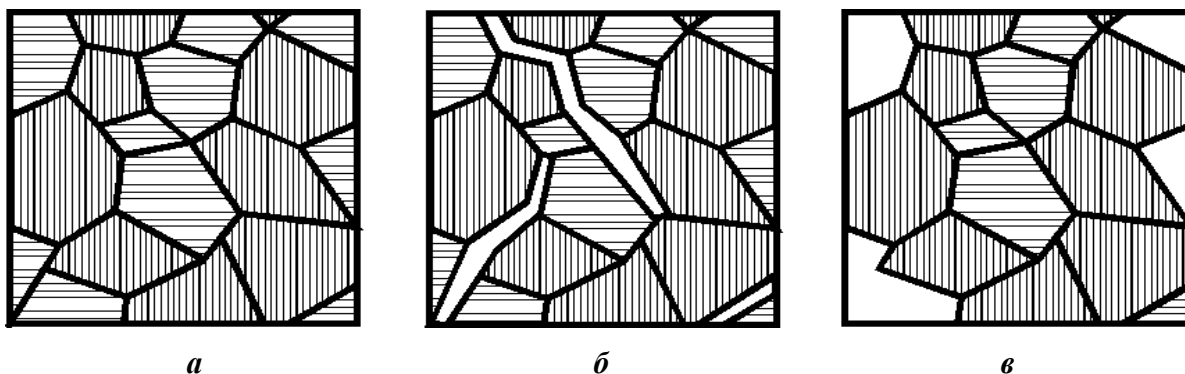
Рисунок 10.1 – Виды коррозионных разрушений металлов:
