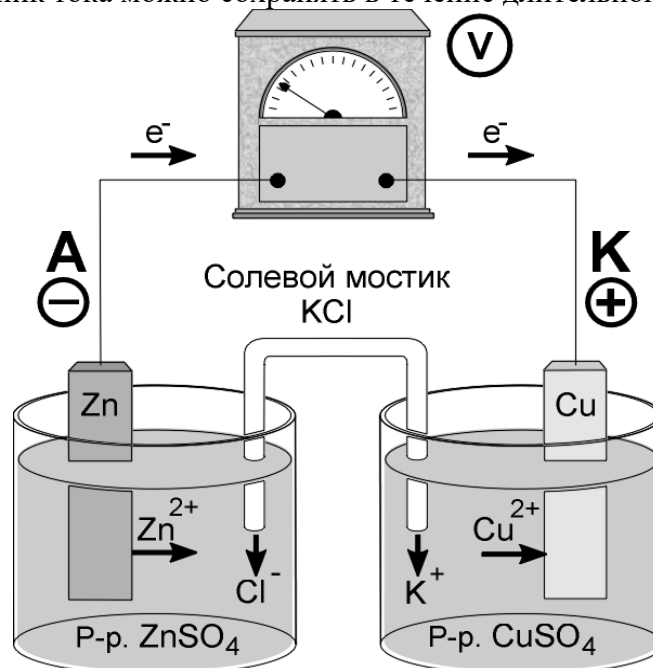
Рисунок 2.3 – Элемент Даниэля
