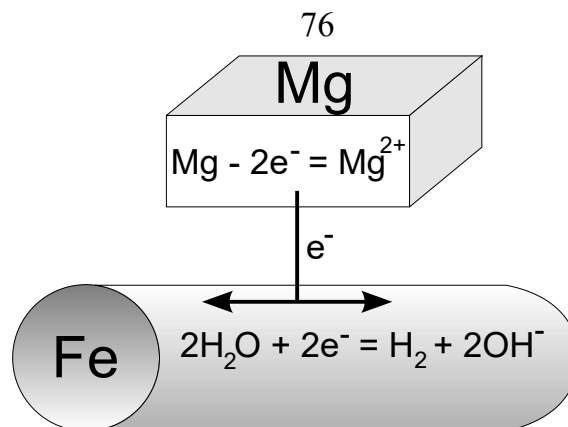
Рисунок 2.5 – Схема процессов, протекающих при катодной защите железного трубопровода в морской воде с помощью магния.
