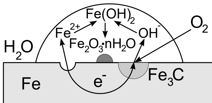
Рисунок 10.3 – Схема коррозии стали с кислородной деполяризацией на микрогальванопаре железо-цементит
