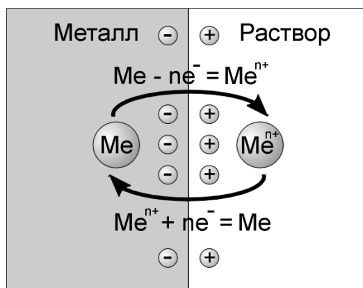
Рисунок 1.1 – Схема, иллюстрирующая механизм образования двойного электрического слоя на границе металл-раствор
