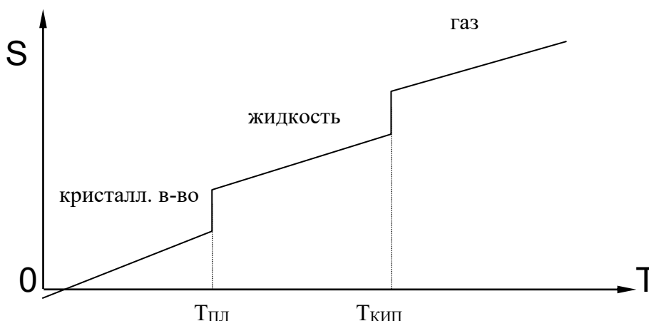
Рисунок 1.1 – Изменение энтропии от температуры
