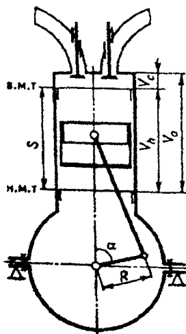
Рисунок 7.1 – Схема для определения основных параметров двигателя поршня S, который равен удвоенному радиусу R кривошипа: S = 2R . При перемещении поршня от одной мертвой точки до другой коленчатый вал поворачивается на угол 180^\circ , т.е. совершает половину оборота
