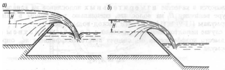
Рисунок 11.7– Водосливы с наклонной тонкой стенкой
