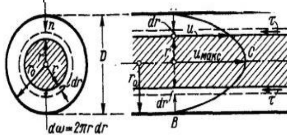
Рисунок 5.4 – Ламинарное равномерное движение в круглой трубе Из формулы (14)
