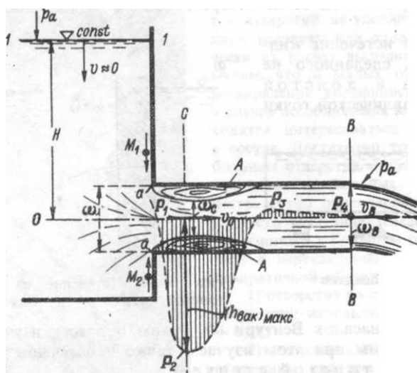
Рисунок 7.9 – Насадок
