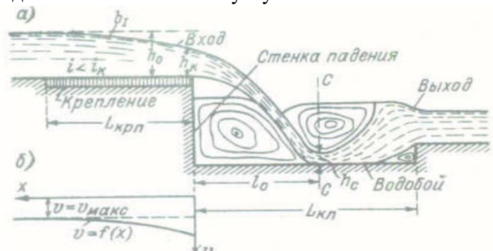
Рисунок 13.1 – Одноступенчатый перепад
