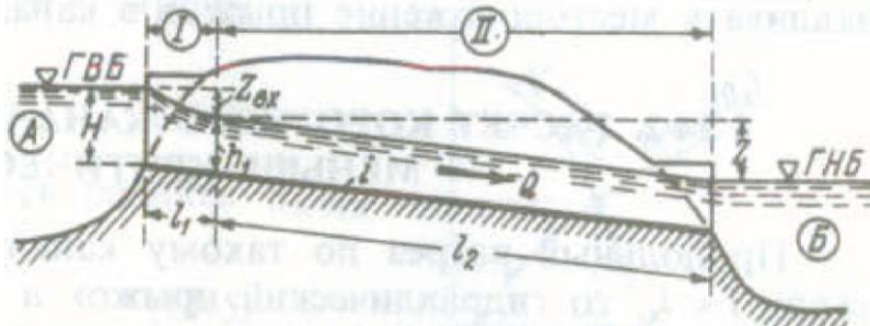
Рисунок 13.5 – Канал, соединяющий два бьефа
