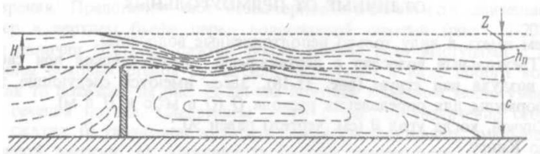
Рисунок 11.14 – Донный и поверхностный режим истечения
