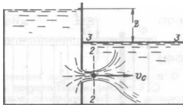
Рисунок 7.6 – Истечение жидкости через затопленное отверстие под уровень
