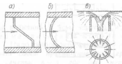
Рисунок 11.6 – Водосливы с непрямолинейным в плане гребнем
