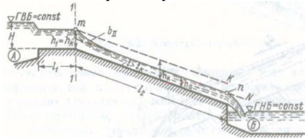
Рисунок 13.9 – Короткий канал (быстроток). i > i_k Истечение в атмосферу.
