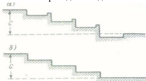
Рисунок 13.2 – Многоступенчатый перепад а) колодезный, б - безколодезный
