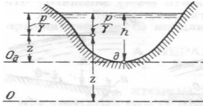
Рисунок 9.3 – К обоснованию формулы критической глубины
