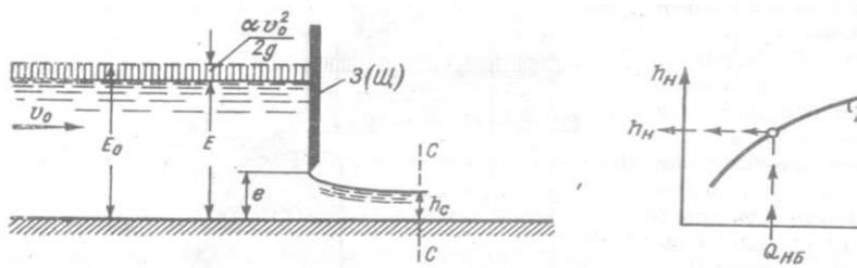
Рисунок 12.3 – Истечение через донное отверстие, например поднимающимся затвором
