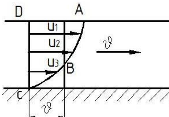
Рисунок 4.15 – Эпюра скорости действительного потока.
