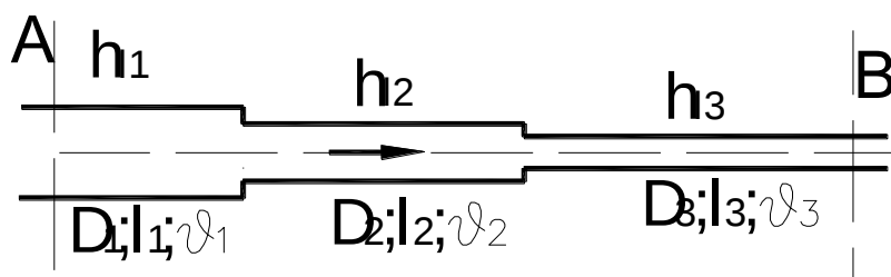
Рисунок 6.8 – Последовательное соединение трубопроводов
