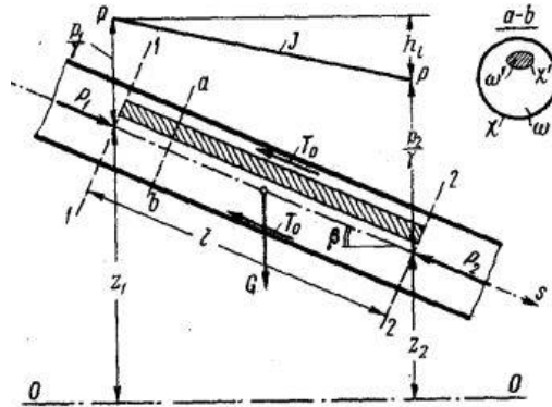
Рисунок 5.2 – К выводу основного уравнения равномерного движения
