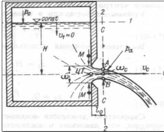
Рисунок 7.1 – Истечение жидкости из малого отверстия в атмосферу
