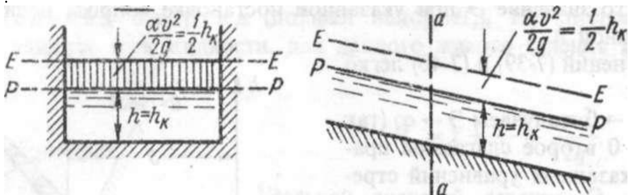
Рисунок 9.6 – Зависимость критической глубины от скоростного напора
