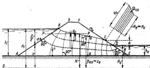
Рисунок 14.14 Фильтрация воды через однородную плотину на водонепроницаемом основании
