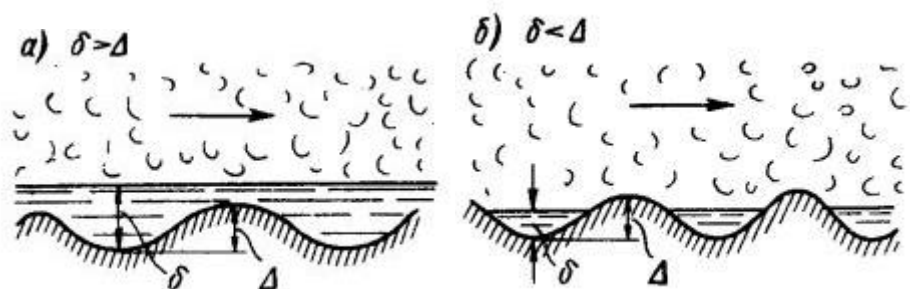
Рисунок 5.8 – Гладкие а) , шероховатые б) русла.
