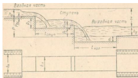
Рисунок 13.3 – План и разрез одноступенчатого перепада
