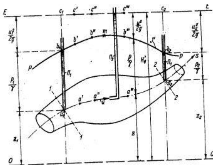
Рисунок 4.14 – Геометрическая интерпретация уравнения Бернулли.
