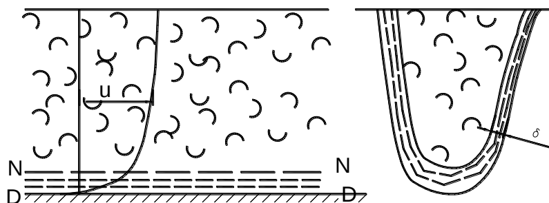
Рисунок 5.7 – Эпюра скоростей при турбулентном движении, вязкий подслой.
