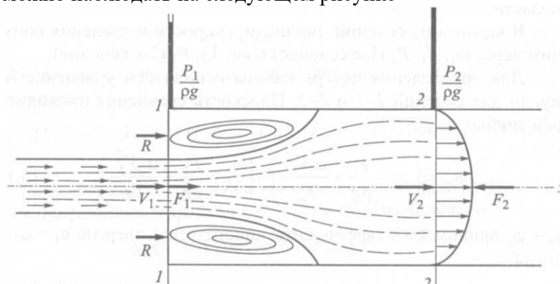
Рисунок 5.12 – Характерные признаки местных сопротивлений
