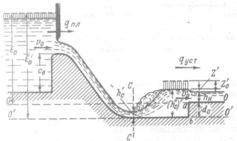
Рисунок 12.14 – К расчету теоретической глубины d_d водобойного колодца
