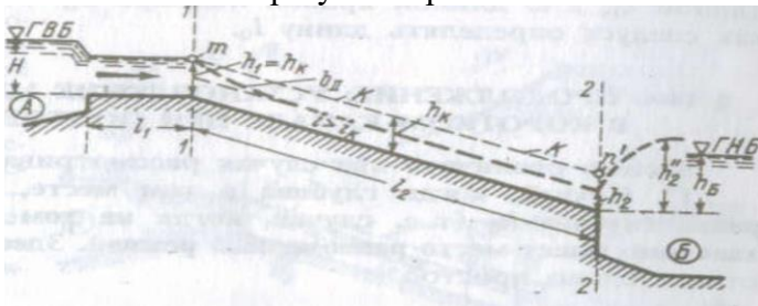
Рисунок 13.10 – Короткий канал, i > i_k ; к расчету подтопления канала нижним бьефом
