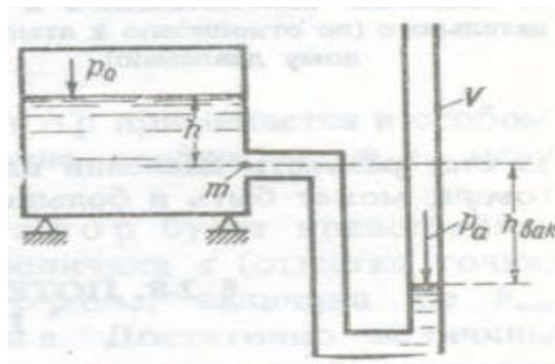
Рисунок 2.8 – Вакуум
