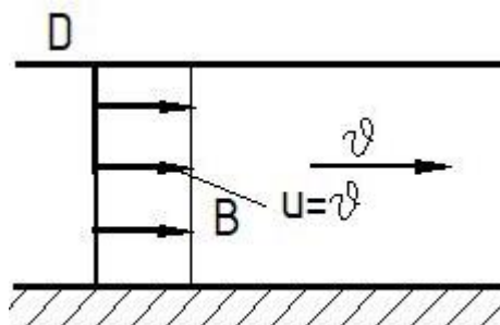
Рисунок 4.16 – Эпюра скорости условного потока
