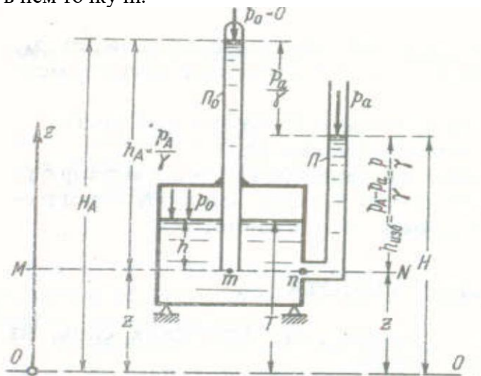
Рисунок 2.7 – Пьезометрическая высота и потенциальный напор
