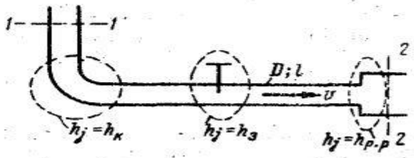
Рисунок 6.1 – Фрагмент трубопровода с различными видами потерь
