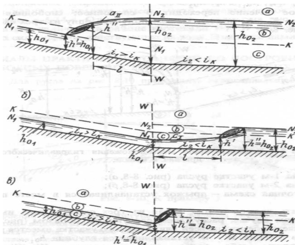
Рисунок 10.4 – К определению местоположения гидравлического прыжка
