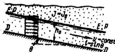
Рисунок 14.7 – Равномерное движение грунтовой воды
