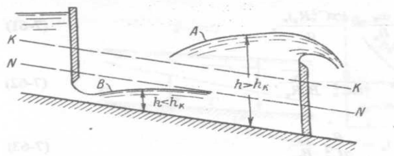
Рисунок 9.10 – Спокойный А и бурный В потоки.
