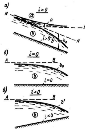
Рисунок 14.11 – Возможные формы свободной поверхности в цилиндрическом русле
