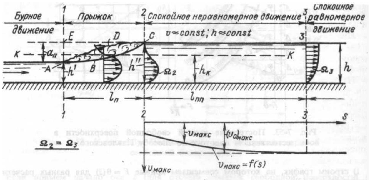
Рисунок 10.1– Гидравлический прыжок и послепрыжковый участок
