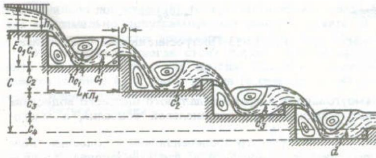
Рисунок 13.4 – К расчету многоступенчатого колодезного перепада
