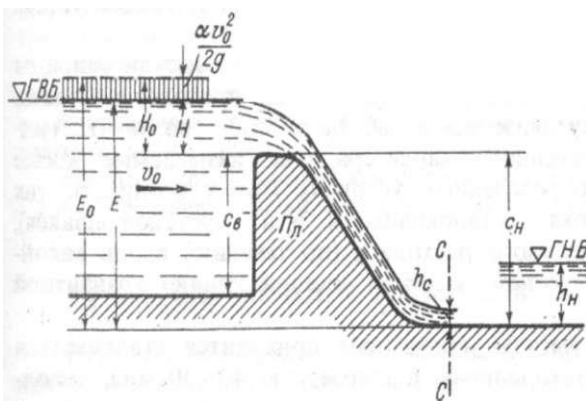
Рисунок.12.1 – Перелив через плотину
