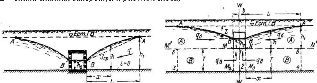
Рисунок 14.12 – Приток воды к галерее расположенной на водоупоре
