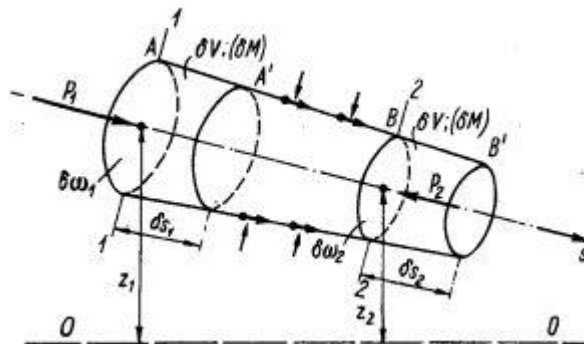
Рисунок 4.13 – К выводу уравнения Бернулли
