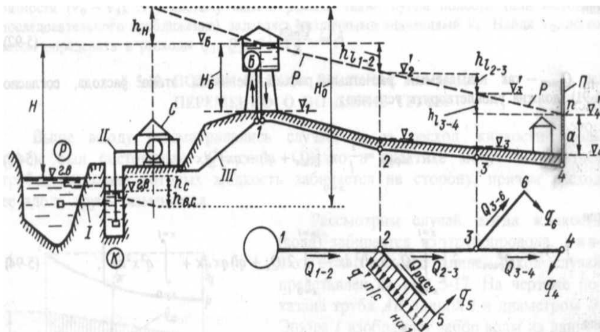
Рисунок 6.12 — Тупиковая (незамкнутая) водопроводная сеть Р — река (источник водоснабжения), К — береговой колодец, С — насосная станция, Б — водонапорная башня, / — самотечная труба, // — всасывающая труба, /// — напорная труба, 1 — 2 — 3 — 4 — магистраль, 2 — 5 и 3 — 6 — ответвления.
