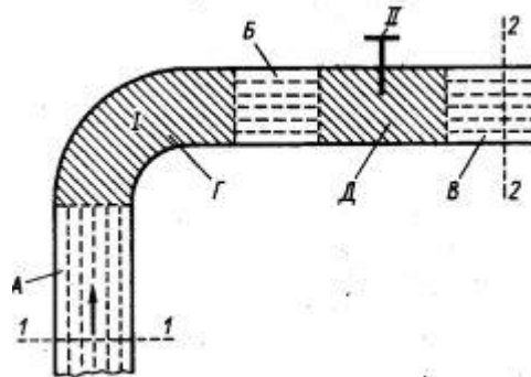
Рисунок 5.1 – Области, в которых имеются сопротивления: А – по длине, В – местные
