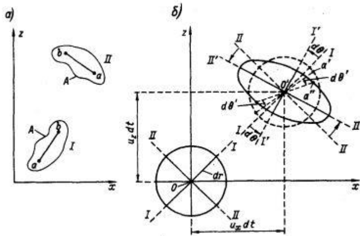
Рисунок 4.3 – Виды движения жидкости
