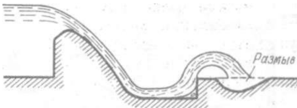
Рисунок 12.19 – Размыв грунта при недостаточной длине колодца
