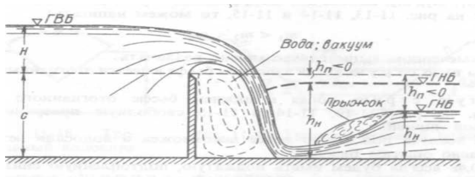
Рисунок 11.12 – Струя поджатая подтопленная снизу
