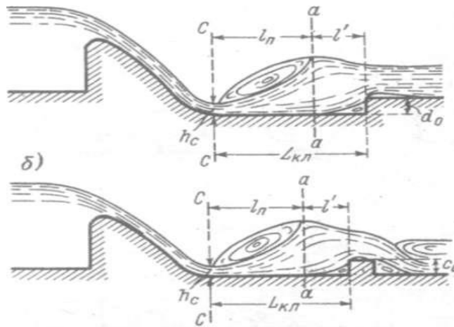
Рисунок 12.18 – Расчетная схема течения воды в пределах колодца
