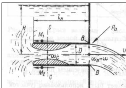
Рисунок 7.10 – Внутренний цилиндрический насадок (насадок Борда)
