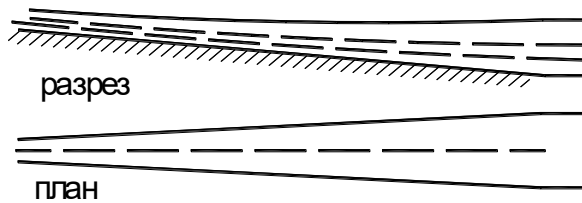
Рисунок 4.11 – Пример неравномерного движения воды на быстротоке
