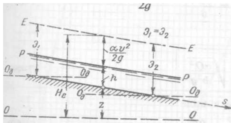
Рисунок 9.5 – Изменение вдоль потока величины H_e (при \mathcal{E} = \text{const} )
