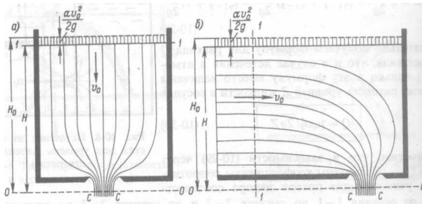
Рисунок 7.7 – Движение жидкости в сосуде
