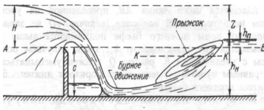
Рисунок 11.10 – Неподтопленный водослив с тонкой стенкой
