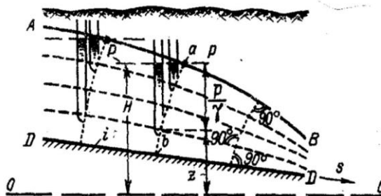
Рисунок 14.8 – Схема действительного фильтрационного потока
