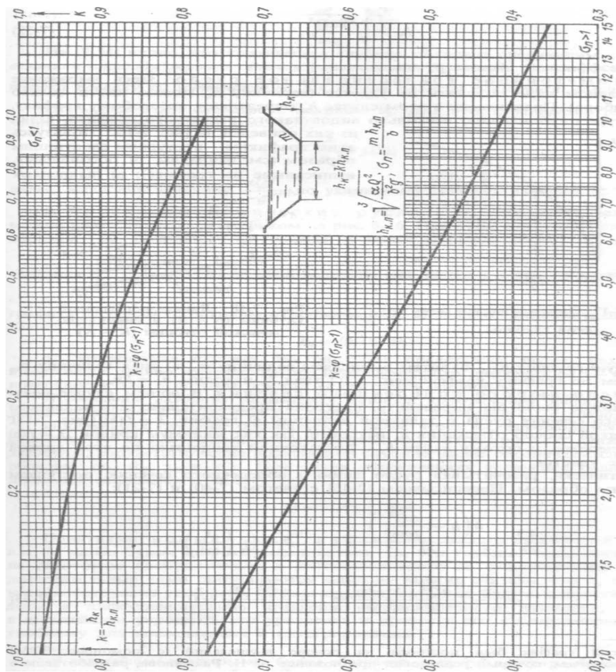
Рисунок 9.7 – График для определения критической глубины для канала трапецидального сечения
