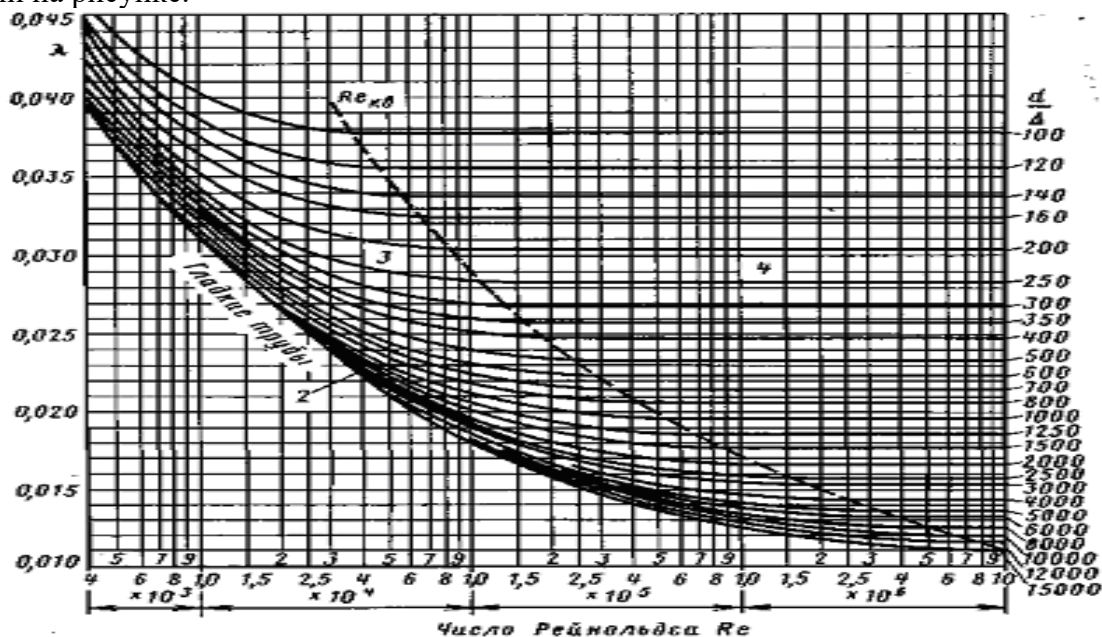
Рисунок 5.10 – График Кольбука для определения коэффициента гидравлического трения
