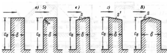
Рисунок 11.21 – Прямоугольные водосливные стенки
