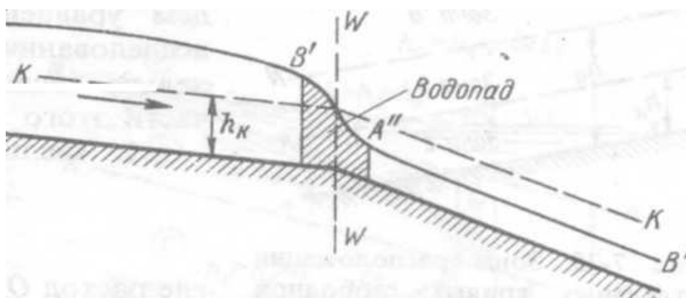
Рисунок 9.12– Водопад (переход спокойного состояния в бурное)
