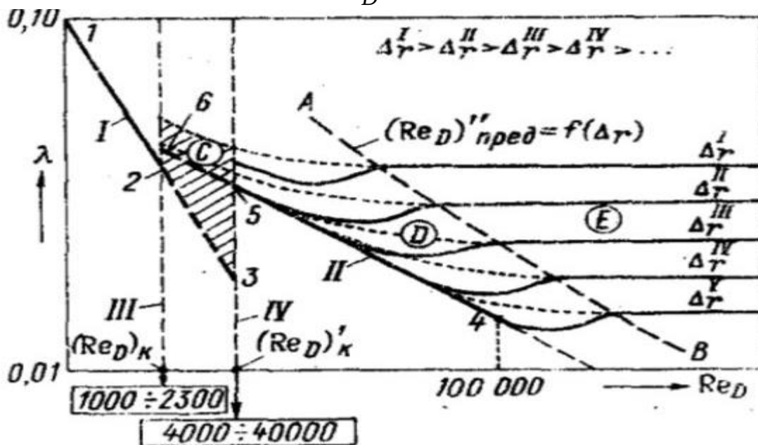
Рисунок 5.9 – Схема графика Никурадзе
