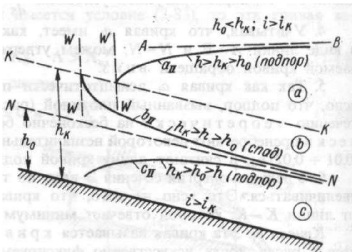
Рисунок 9.18 – Формы отдельных кривых при i > i_{кр}
