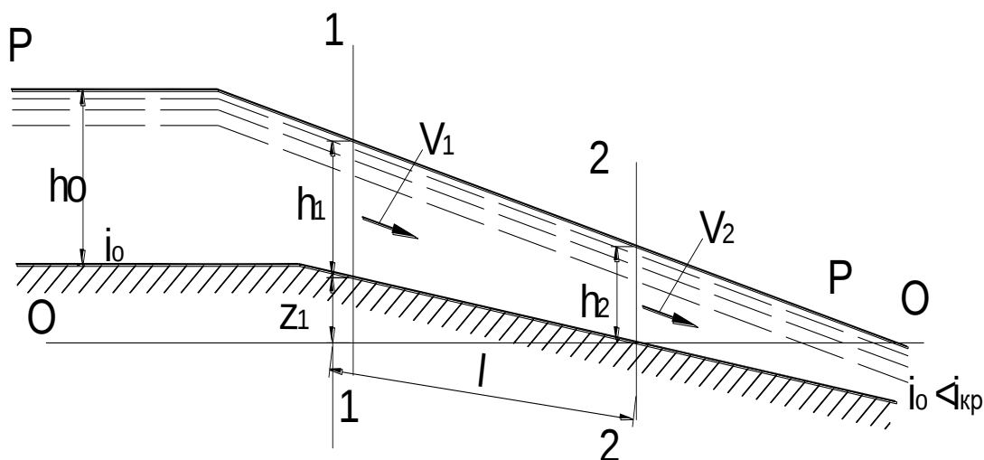
Рисунок 9.21 – К выводу уравнения В. Чарномского
