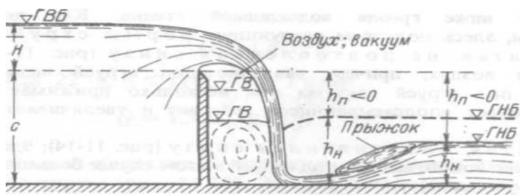
Рисунок 11.11 – Струя поджатая неподтопленная снизу
