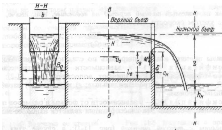
Рисунок 11.1 – Истечение через водослив с тонкой стенкой
