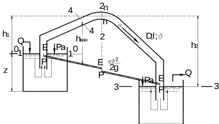
Рисунок 6.4 – Сифон
