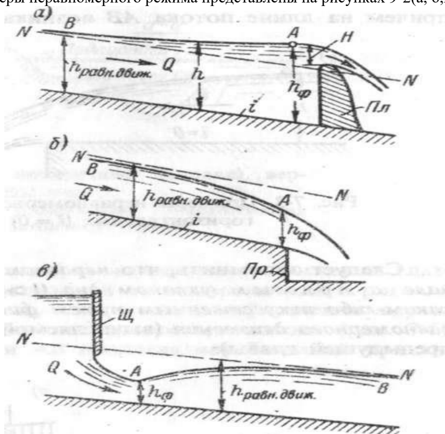
Рисунок 9.2 – Примеры неравномерного движения в цилиндрическом канале с прямым уклоном ( i > 0 )
