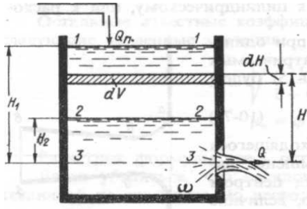
Рисунок 7.11 – Истечение жидкости в атмосферу при переменном напоре
