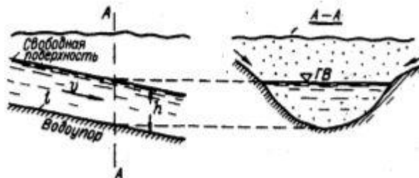
Рисунок 14.1 – Равномерное движение грунтовой воды
