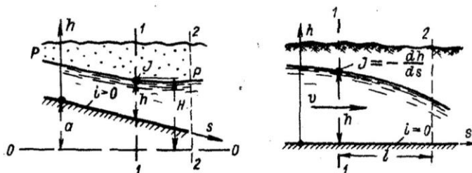
Рисунок 14.10 – К выводу дифференциального уравнения неравномерного движения
