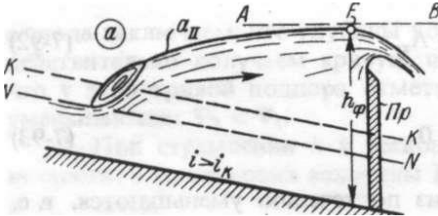
Рисунок 9.19 – Кривая свободной поверхности типа a_{II} .
