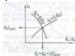
Рисунок 13.7 – К расчету быстротока при i < i_k
