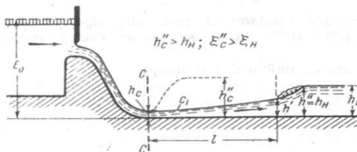
Рисунок 12.5 – Сопряжение бьефов при помощи отогнанного прыжка
