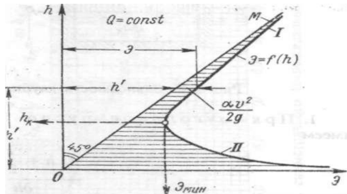
Рисунок 9.4 – График удельной энергии сечения \mathcal{E}
