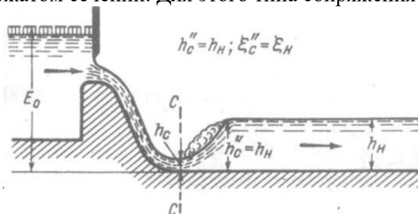
Рисунок 12.7 – Прыжок в сжатом сечении
