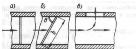
Рисунок 11.5 – Водосливы с прямолинейным гребнем в плане
