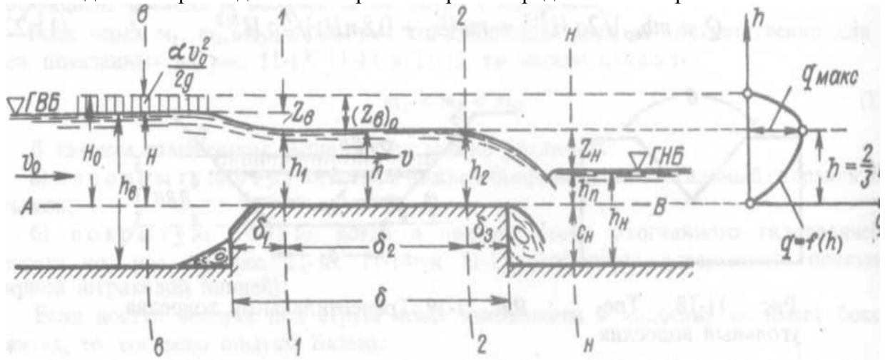
Рисунок 11.15 – Неподтопленный водослив с широким порогом
