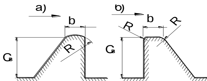
Рисунок 11.24 – Водосливы со стенкой трапецидального очертания со скругленными углами;
