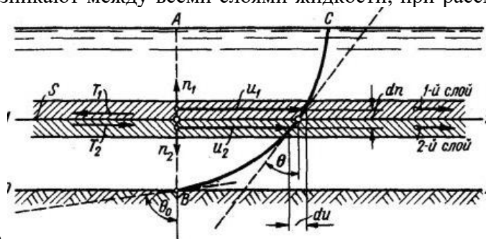
Рисунок 5.3 – К пояснению законов продольного внутреннего трения
