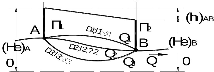
Рисунок 6.10 – К расчету параллельного соединения трубопроводов Потеря напора от узла А к узлу В будет равна:
