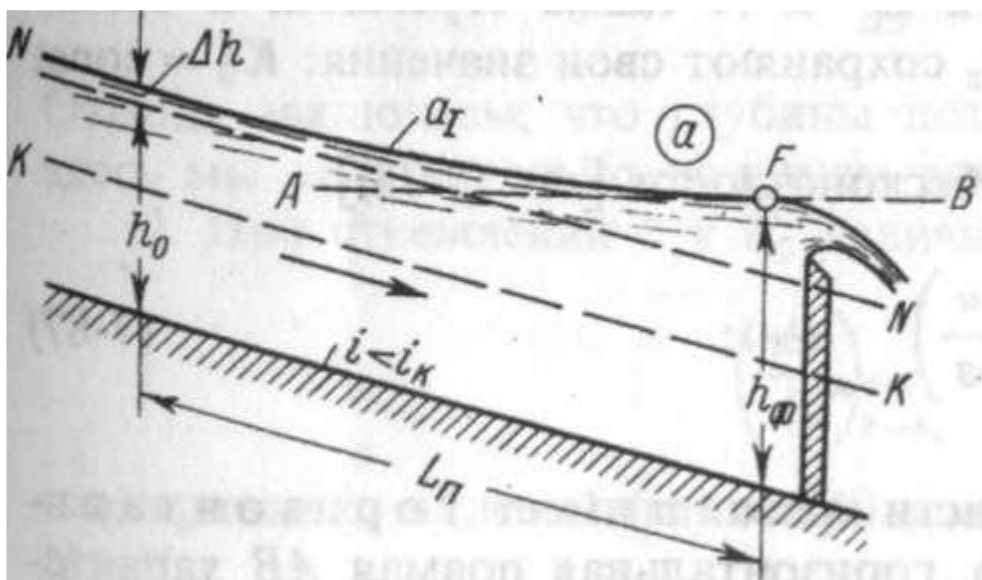
Рисунок 9.15 – Кривая свободной поверхности типа a_1
