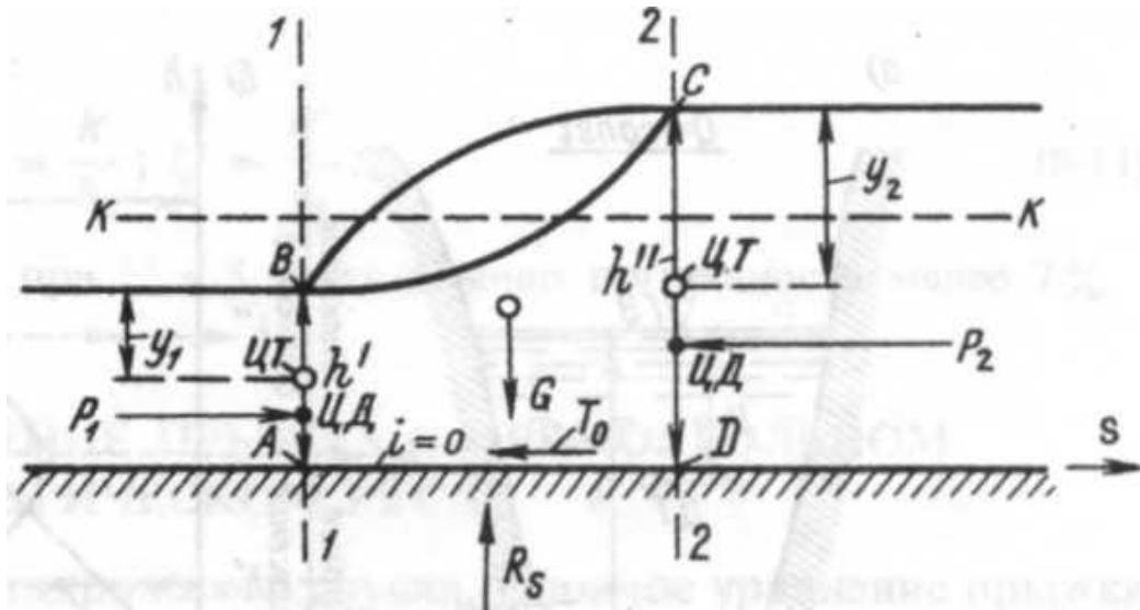
Рисунок 10.2 – Схема гидравлического прыжка
