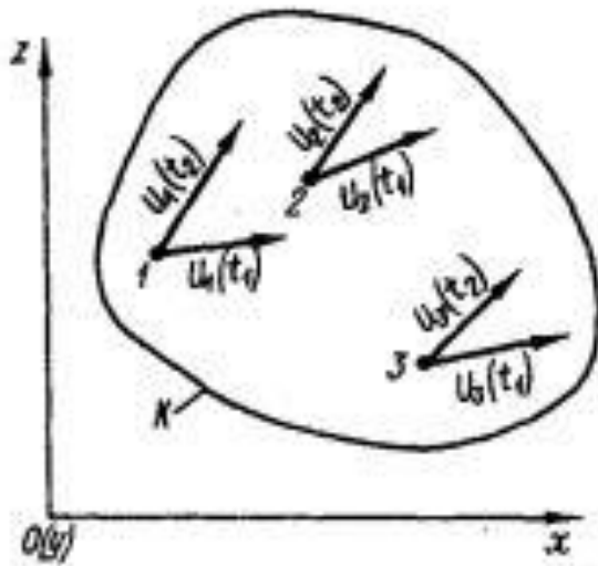
Рисунок 4.2 – К методу Эйлера.
