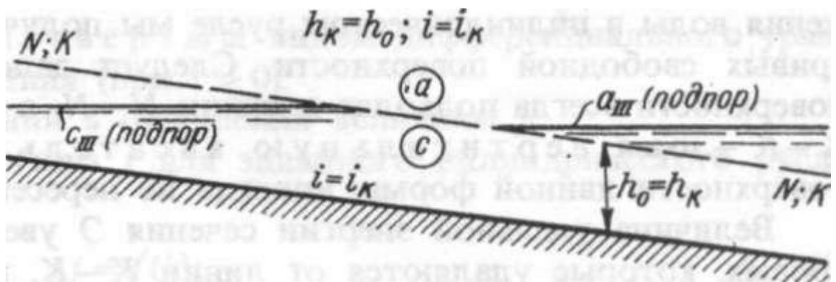
Рисунок 9.20 – Формы кривых свободной поверхности при i=i_K
