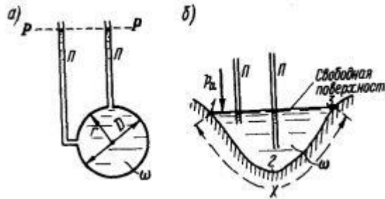
Рисунок 4.12 – Пример напорного а), безнапорного б) движения жидкости
