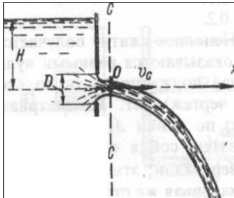
Рисунок 7.5 – Траектория струи
