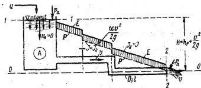
Рисунок 6.3 – Короткий трубопровод, истечение в атмосферу
