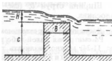
Рисунок 11.3 – Водослив с широким порогом
