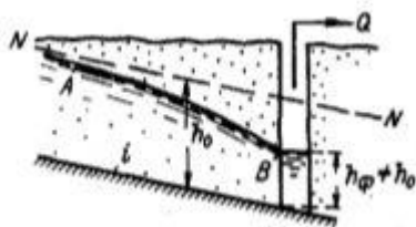
Рисунок 14.2 – Неравномерное движение грунтовой воды
