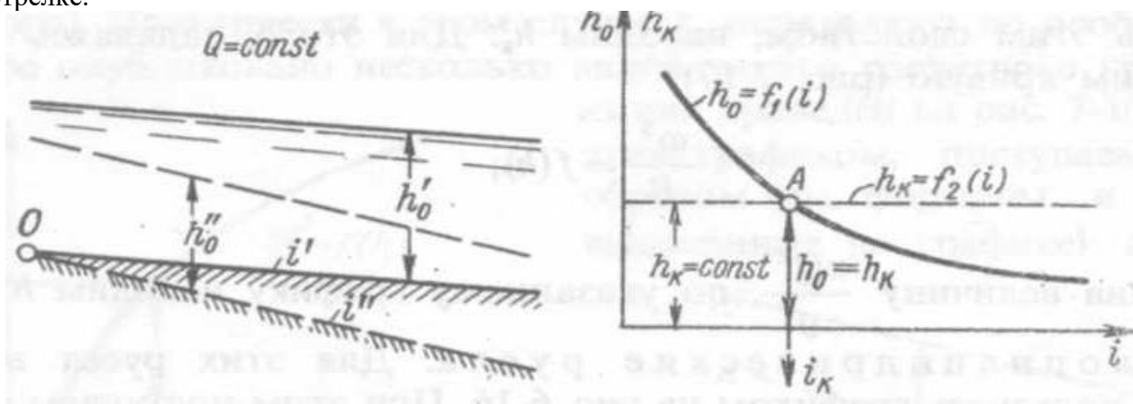
Рисунок 9.8 – К определению критического уклона
