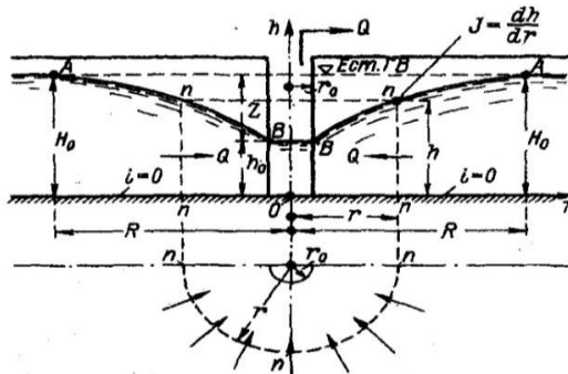
Рисунок 14.13 – Приток воды к галерее расположенной на водоупоре
