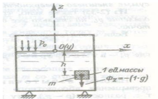
Рисунок 2.6 – Давление p для жидкости, находящейся под действием силы тяжести
