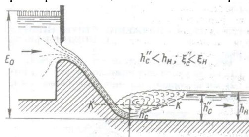
Рисунок 12.6 – Сопряжение бьефов при помощи затопленного прыжка
