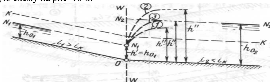
Рисунок 10.3 – К определению местоположения гидравлического прыжка в русле
