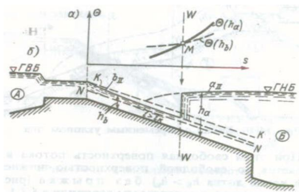
Рисунок 13.12 – Определение местоположения прыжка в канале (не прямоугольное русло)
