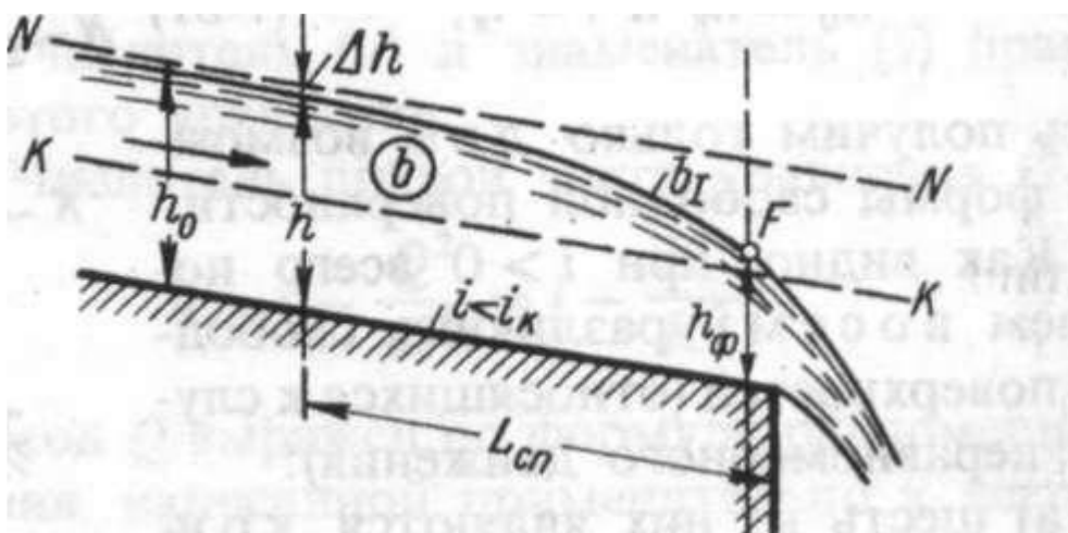
Рисунок 9.16 – Кривая свободной поверхности типа b_1
