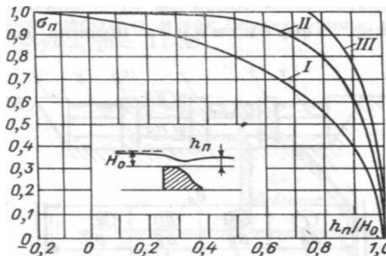
Рисунок 11.19 – График для определения коэффициента подтопления водослива: I- вакуумного, II – безвакуумного, III - безвакуумного с уширенным гребнем.
