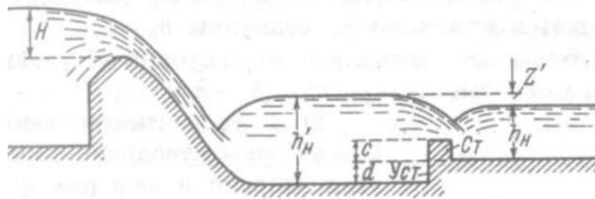
Рисунок 12.13 – Водобойный колодец комбинированного типа
