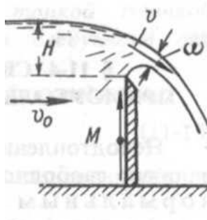
Рисунок 11.8 – Принципиальная схема нормального водослива
