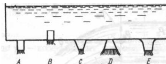
Рисунок 7.8 – Типы насадков
