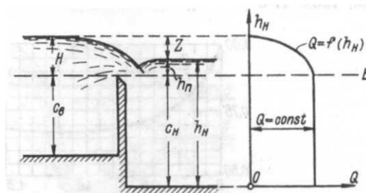
Рисунок 11.9 – Подтопленный водослив с тонкой стенкой
