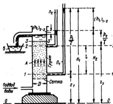
Рисунок 14. 6 – Установка Дарси
