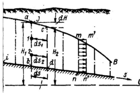
Рисунок 14.9 – Расчетная модель фильтрационного потока по Дюпюи
