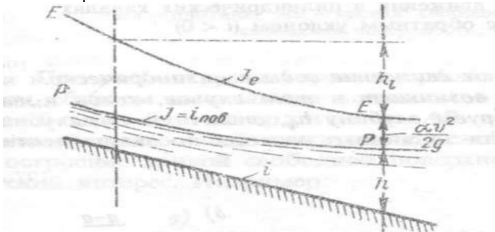
Рисунок 9.1 – Неравномерное движение
