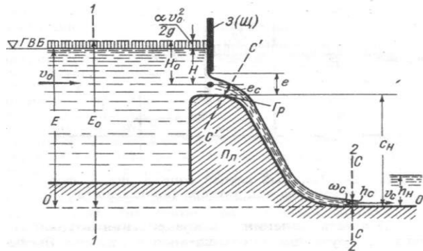
Рисунок 12. 8 – Общий случай сопряжения бьефов. Плотина с затвором
