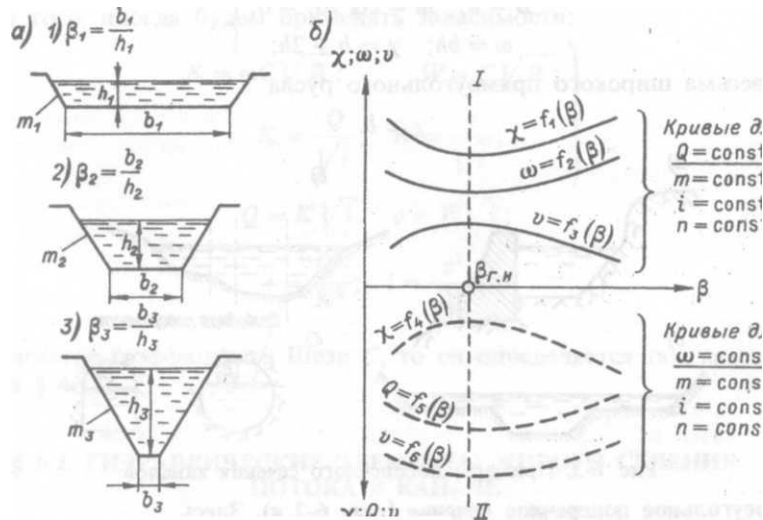
Рисунок 8.4 – Изменение элементов живого сечения \chi, \omega, v, Q с изменением относительной ширины \beta трапецеидального канала
