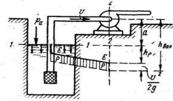
Рисунок 6.6 – К расчету вакуума во всасывающей трубе насоса
