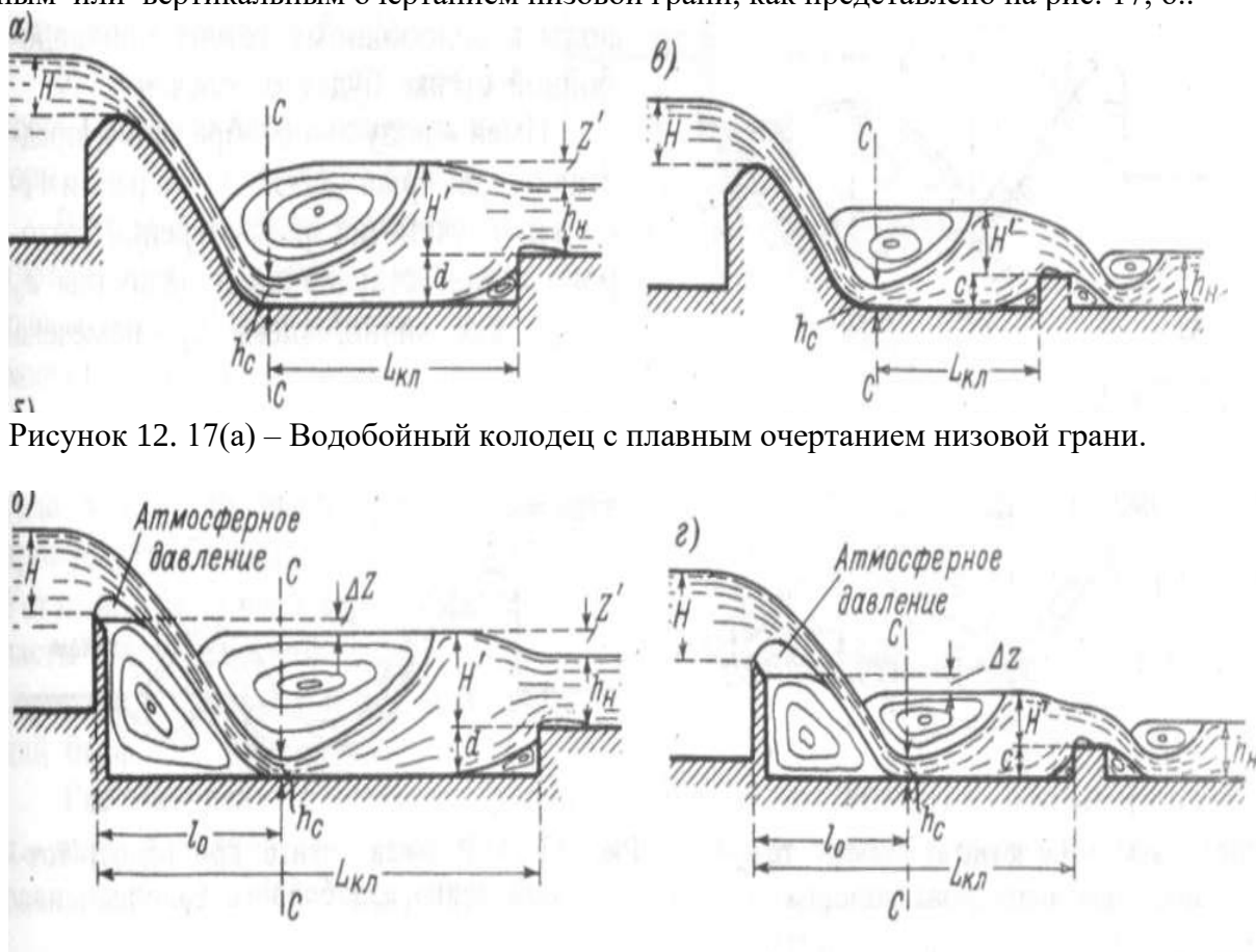
Рисунок 12.17 (б) – Водобойный колодец, образованный уступом.
