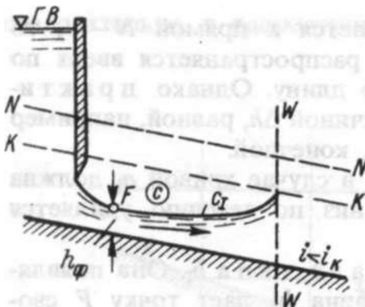
Рисунок 9.17 – Кривая свободной поверхности типа C_1 Второй случай характеризуется условиями (9.18).
