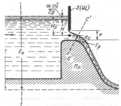
Рисунок 12.2– Истечение из-под затвора
