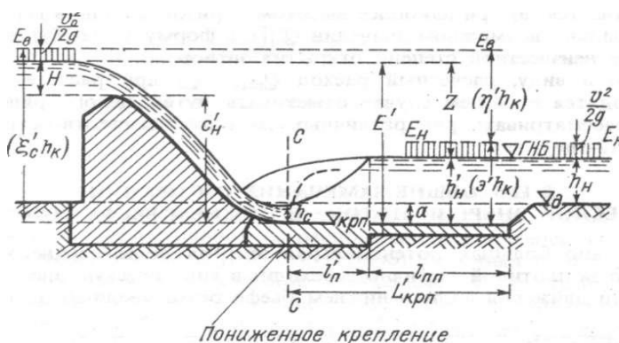
Рисунок 12.10 - К расчету отметки пониженного крепления НБ
