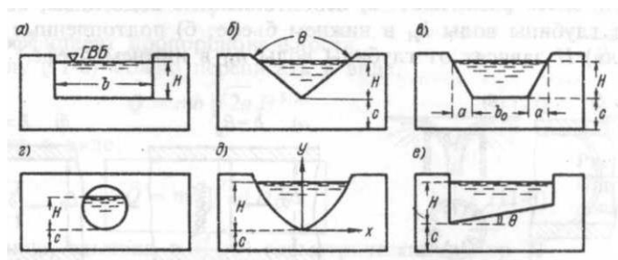
Рисунок 11.2 – Формы водосливных отверстий
