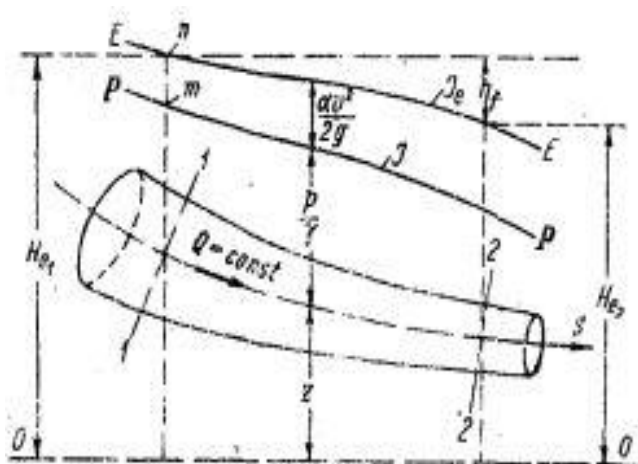
Рисунок 4.17 – Геометрическая интерпретация уравнения Бернулли для реальной жидкости
