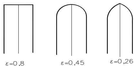
Рисунок 11.20 – Зависимость коэффициента уменьшения от очертания входной грани быка
