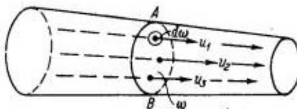
Рисунок 4.9– Живое сечение А-В.
