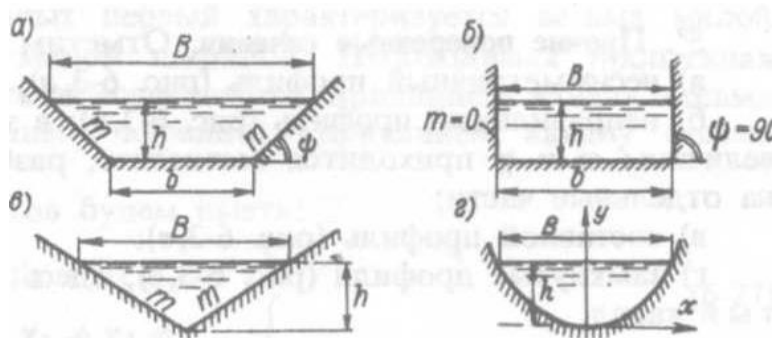
Рисунок 8.2 – Примеры поперечного сечения каналов
