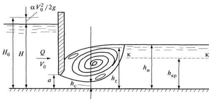
Рисунок 11.27 – Истечение жидкости из-под затвора в форме надвинутого прыжка
