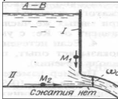
Рисунок 7.3 – Пример неполного сжатия
