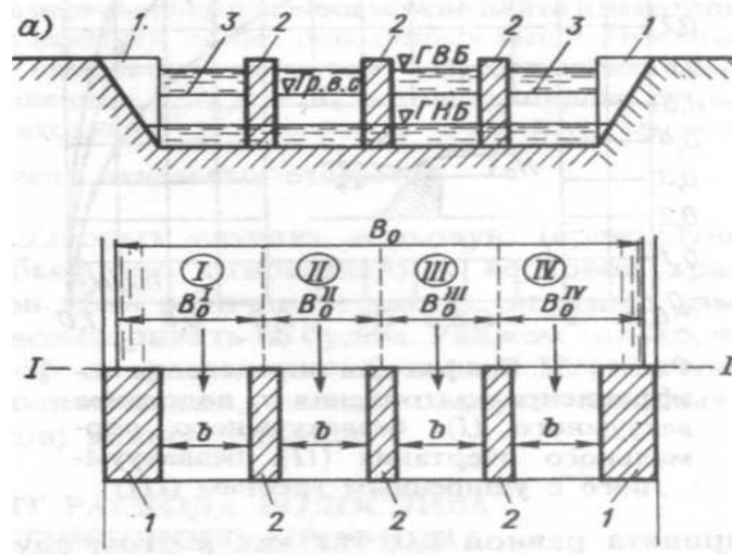
Рисунок 11.18 – Разрез и план плотины: а) разрез, б) план.
