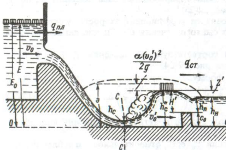
Рисунок 12.15 – К расчету теоретической высоты c_o водобойной стенки Удельный расход водобойной стенки в общем случае определяют по формуле
