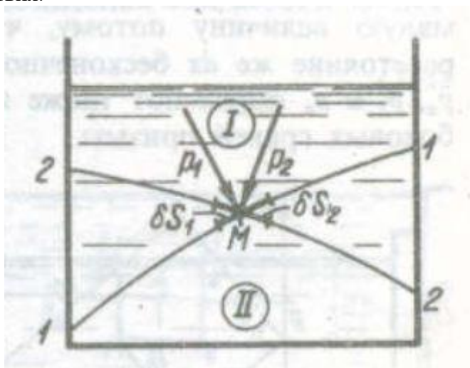
Рисунок 2.2 – Направление гидростатического давления в точке
