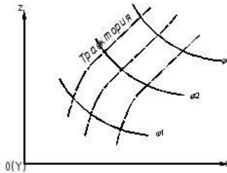
Рисунок 4.5 – Скалярное поле потенциальной функции
