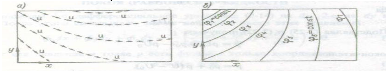
Рисунок 2.5 – Векторное поле скоростей и скалярное поле потенциальной функции поля скоростей.
