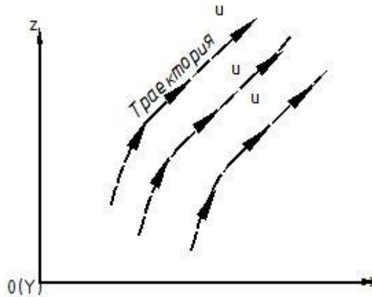
Рисунок 4.4 – Векторное поле скоростей.
