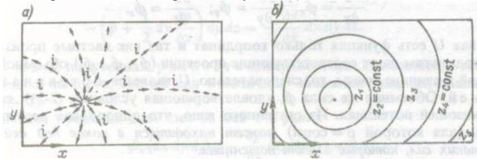
Рисунок 2.4 – Замена векторного поля (а) уклонов земной поверхности скалярным полем отметок земной поверхности.
