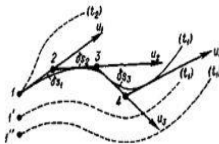
Рисунок 4.7 – Схема траектории частицы 1 жидкости при неустановившемся движении.
