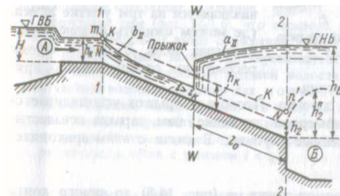
Рисунок 13.11 – Короткий канал, i > i_k , прыжок в канале
