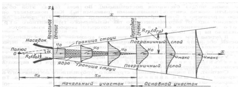
Рисунок 7.12 – Схема свободной турбулентной струи
