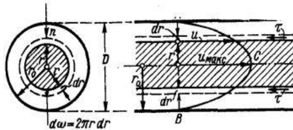
Рисунок 5.5 – К выводу формулы потерь напора при ламинарном равномерном установившемся движении
