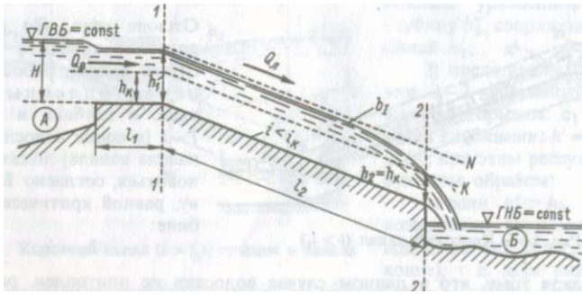
Рисунок 13.8 – Короткий канал (быстроток). i < i_k Истечение в атмосферу.
