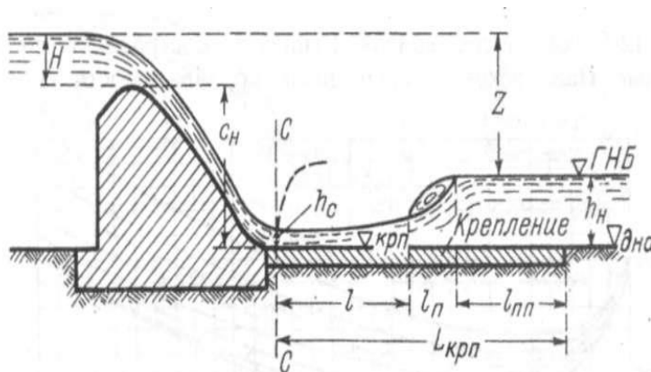
Рисунок 12.9 – К расчету длины крепления нижнего бьефа
