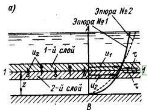
Рисунок 5.6 – К вопросу о турбулентных касательных напряжениях
