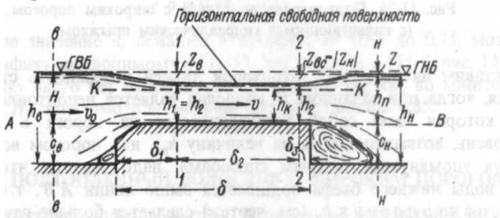
Рисунок 11.16 – Подтопленный водослив с широким порогом Z_{вс} – перепад восстановления.
