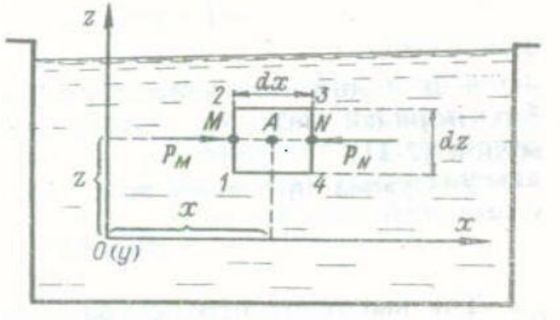
Рисунок 2.3 – К выводу дифференциального уравнения покоя жидкости
