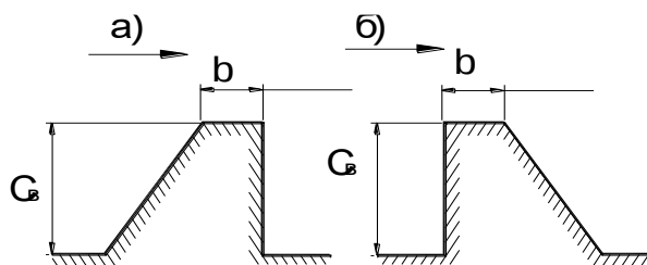
Рисунок 11.22 – Трапецидальные водосливные стенки
