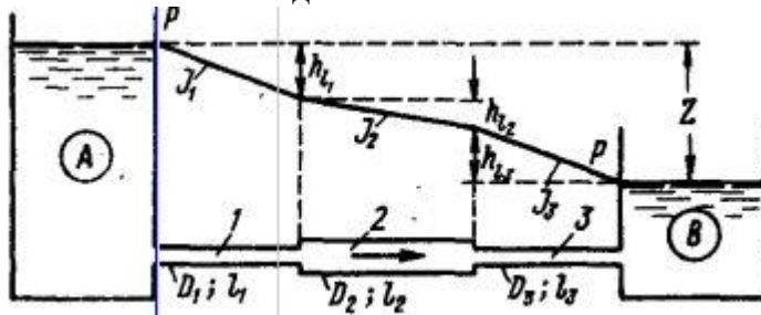
Рисунок 6.7 – Простой длинный трубопровод переменного сечения
