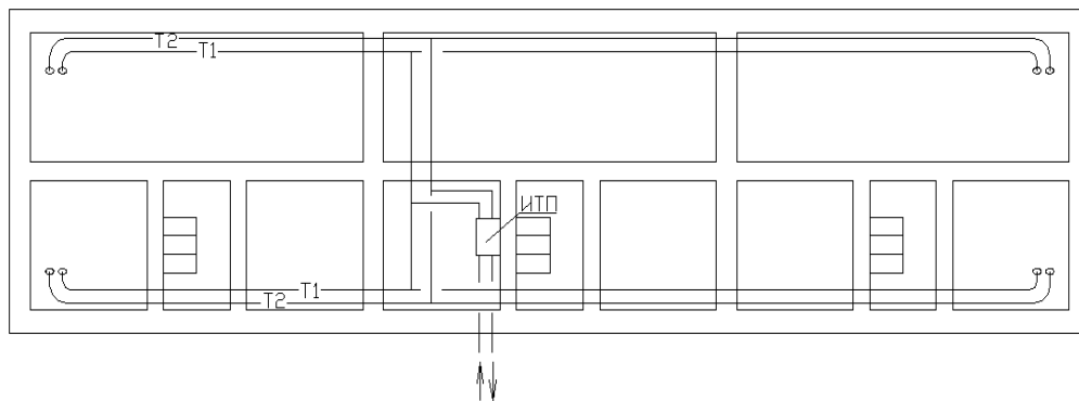
рис. 4.6 — Расположение магистралей системы водяного отопления с нижней разводкой
