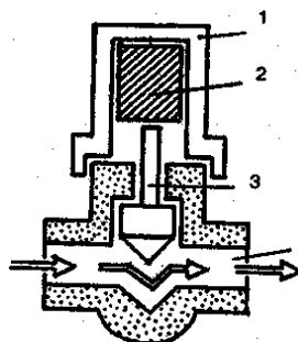
рис.1.3 — Термостатический клапан: 1 – термоголовка; 2 – рабочее вещество; 3 – клапан.
