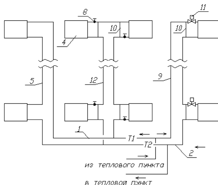
рис.4.2 — Схема вертикальной однетрубной системы водяного отопления с нижней разводкой подающих магистралей и тупиковым движением воды 12 – П-образный стояк со смещенными замыкающими участками 10
