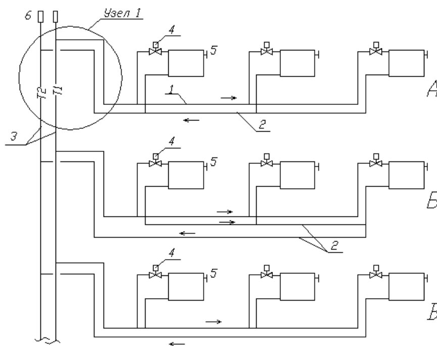
рис.5.1 — Схемы систем отопления с горизонтальной разводкой труб 1 – подающий трубопровод Т1, 2 – обратный трубопровод Т2, 3 – магистральные стояки, устанавливаемые на лестничной клетке, 4 – термостатический клапан с термоголовкой, 5 – ручной воздухоотводчик, 6 – автоматический воздухоотводчик.
