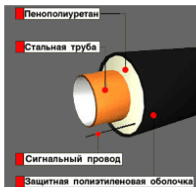
рис.8.1 — Устройство ПИ-труб
