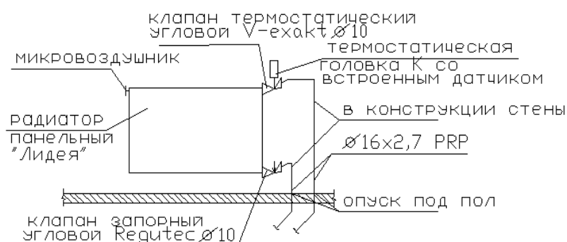
рис.6.2 — Узел подключения радиатора
