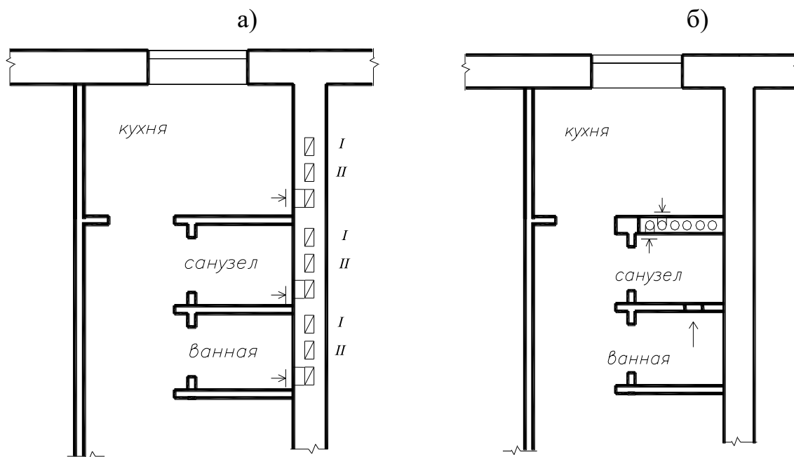
рис.6.1 — Устройство вентиляционных каналов:
