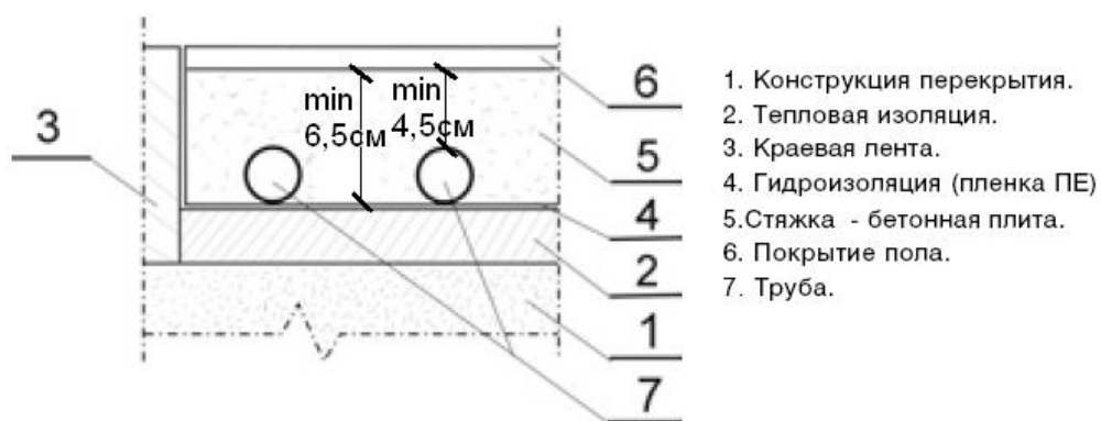
рис.9.1 — Схема конструкции подпольного нагрева с укладкой мокрым методом
