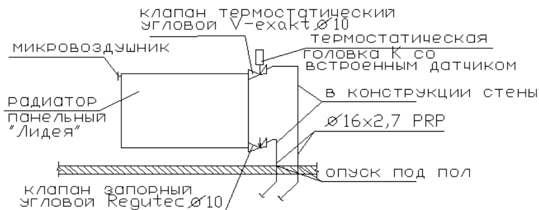
рис.4.2 — Узел подключения радиатора (узел 2)
