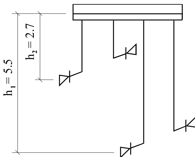
рис.6.4 — Схема вытяжной системы вентиляции с обособленными каналами
