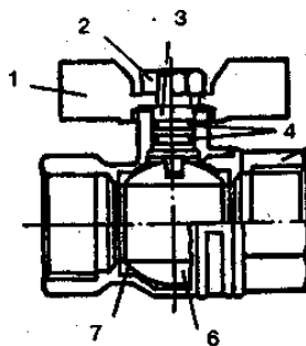
рис.1.2 — Шаровой кран:
