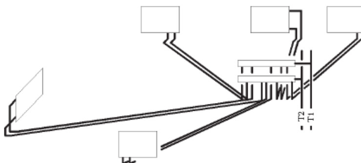
рис.5.4 — Схема поквартирной системы водяного отопления с лучевой веткой
