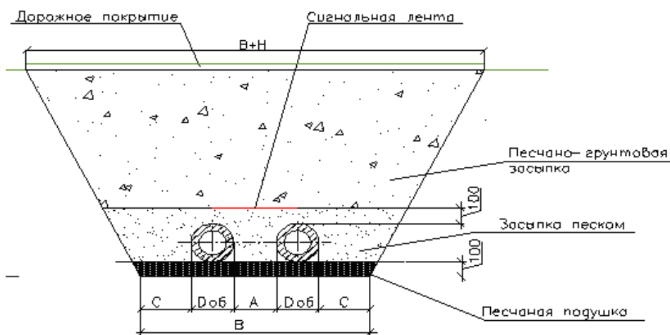
рис.8.4 — Бесканальная прокладка ПИ-трубопроводов
