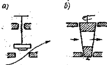
рис.1.1 — Принципиальные схемы действия арматуры: вентиль (а), пробкового (шарового) крана (б).
