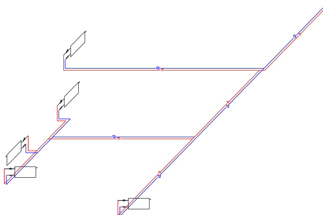
рис.5.3 — Схема квартирной петлевой смешанной двухтрубной системы водяного отопления.
