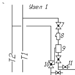
рис.5.5 — Узел 1 — Ввод в квартирные системы отопления
