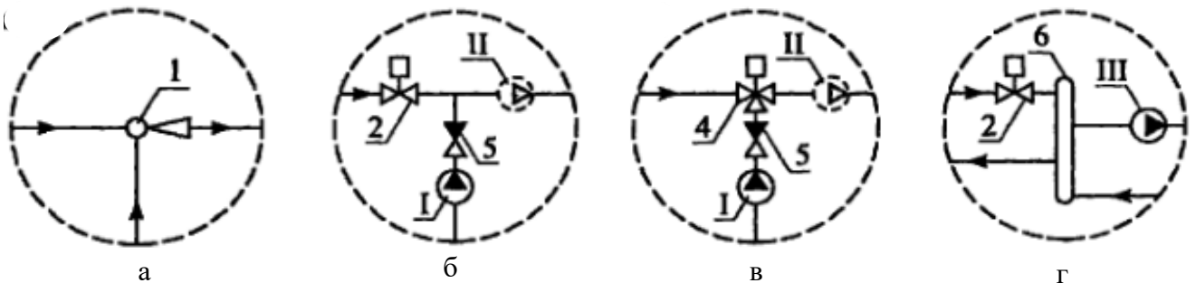
рис.2.1 — Схемы узлов смешения
