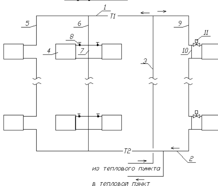
Устройство вертикальной систем водяного отопления с искусственной циркуляцией
