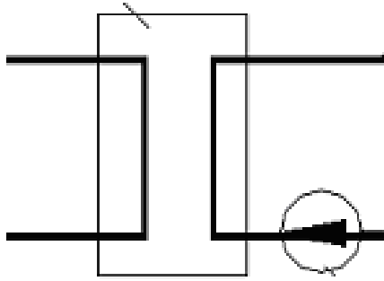
рис.2.2 — Независимая схема подключения: 1 – теплообменник, 2 – циркуляционный насос
