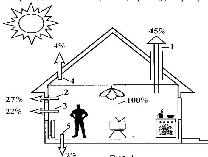
Рис. 2.1 — Примерная структура теплового баланса жилого дома в холодный период года
