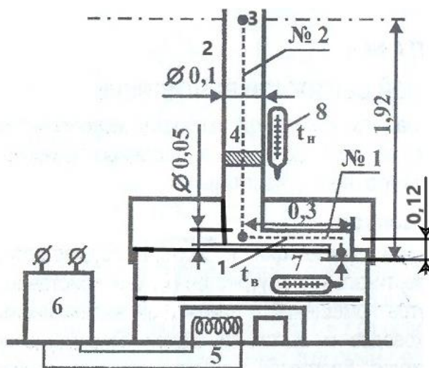
рис.7.1 — Опытная установка
