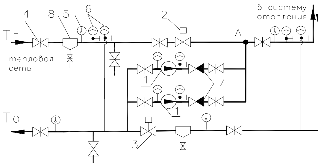
рис.5.2 — Принципиальная схема местного теплового пункта при зависимом присоединении системы водяного отопления к наружным тепловым сетям со смесительным насосом, включенным в перемычку.
