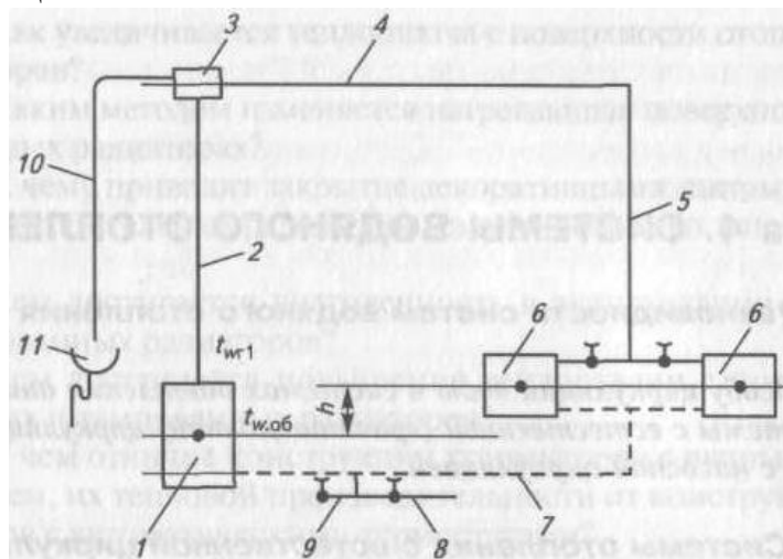
рис.4.4 – Схема системы водяного отопления с естественной циркуляцией
