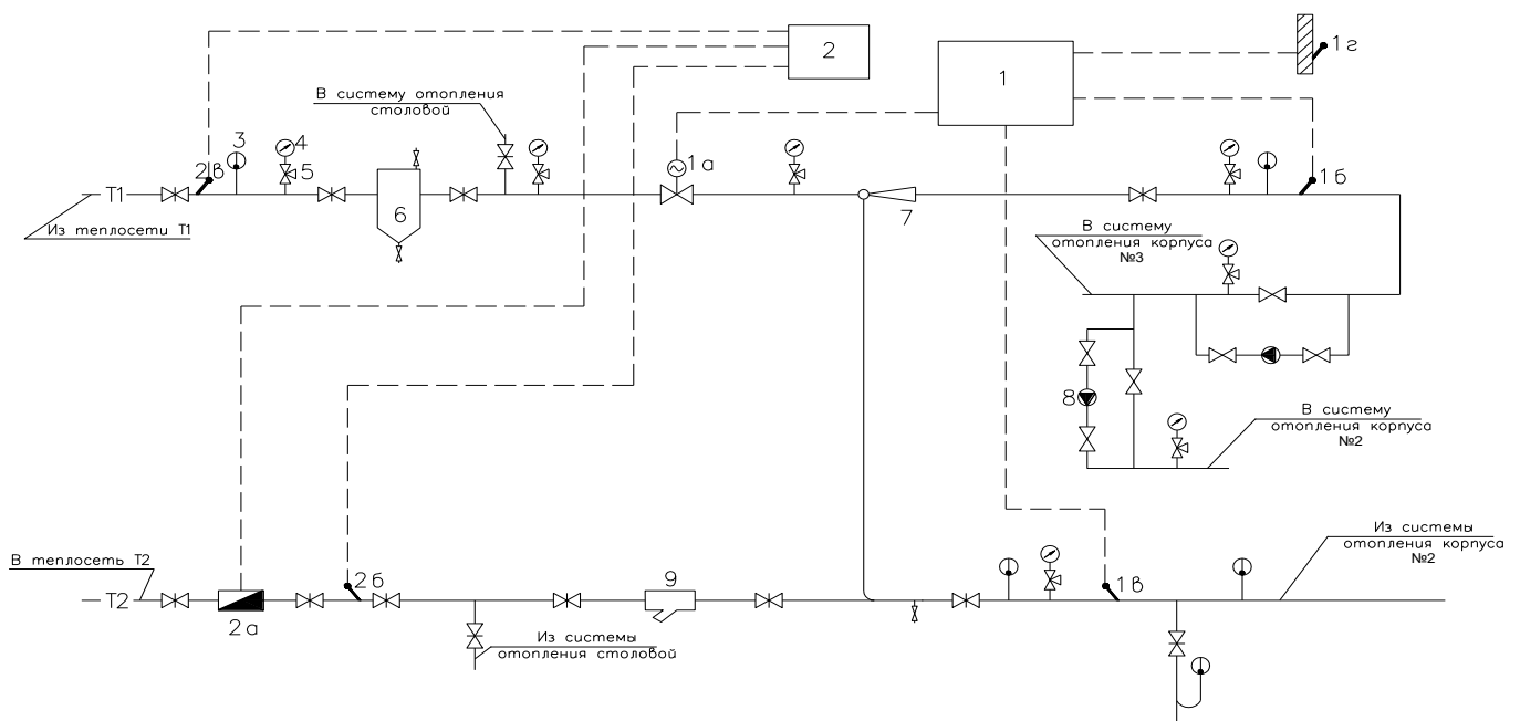
рис.2.3 — Зависимая схема теплового пункта со смесительным элеваторным узлом
