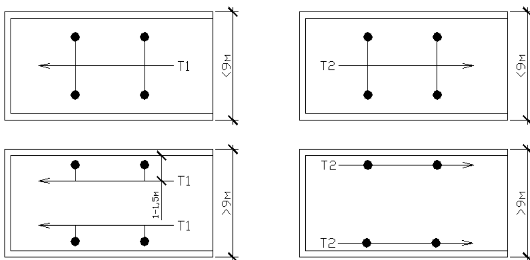
рис. 4.5 – Расположение магистралей системы водяного отопления
