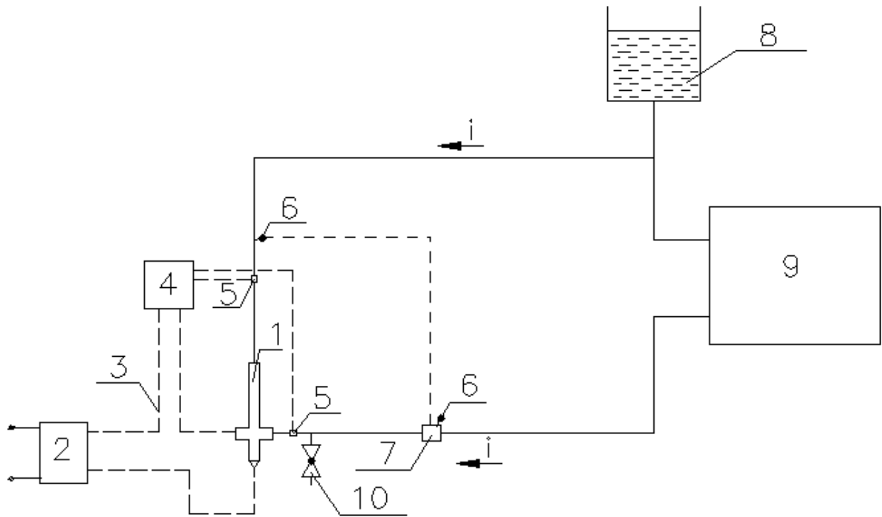
рис.5.1 — Схема экспериментального стенда
