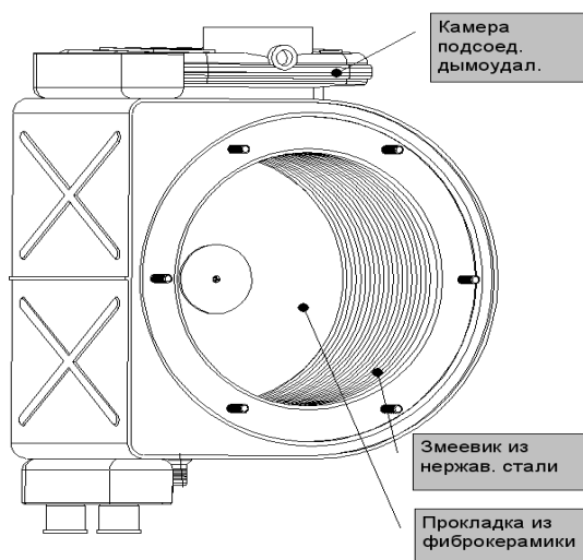
рис.6.1 — Схема теплообменника АОГВ-50-ЗП
