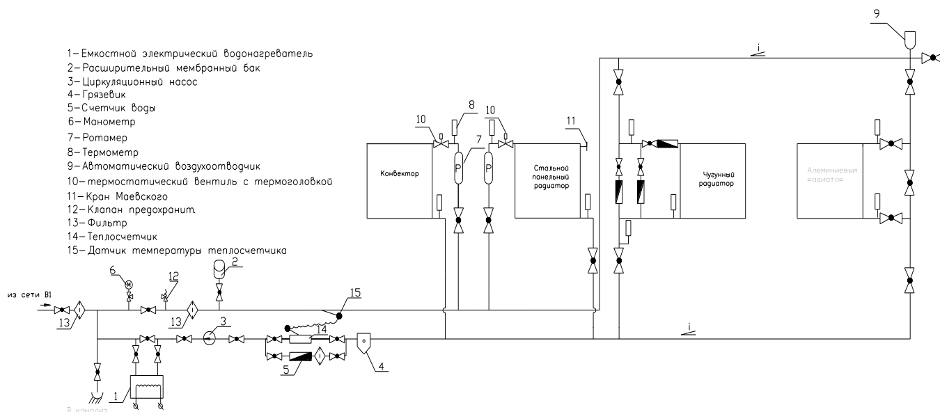
рис.3.1 — Схема измерительного стенда
