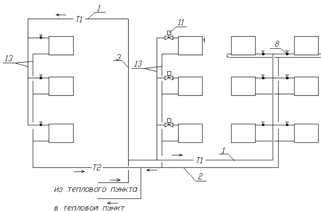
рис.4.3 — Схема вертикальной двухтрубной системы водяного отопления с верхней и нижней разводкой подающих магистралей и тупиковым движением воды 13 – подающая и обратная части стояка
