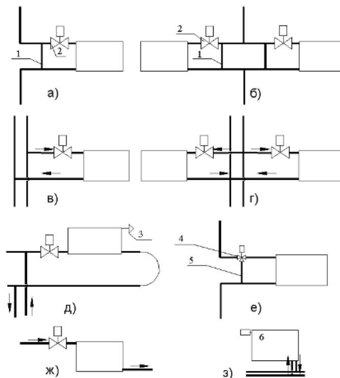
рис.6.1 — Присоединение отопительных приборов к стоякам вертикальных систем отопления:
