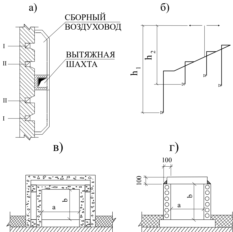
рис.6.2 — Вентшахта с объединенными вентканалами:
