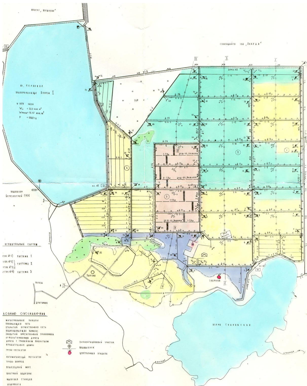
Рисунок 4.19 – Схема запроектированных мероприятий на объекте «Спорово»
