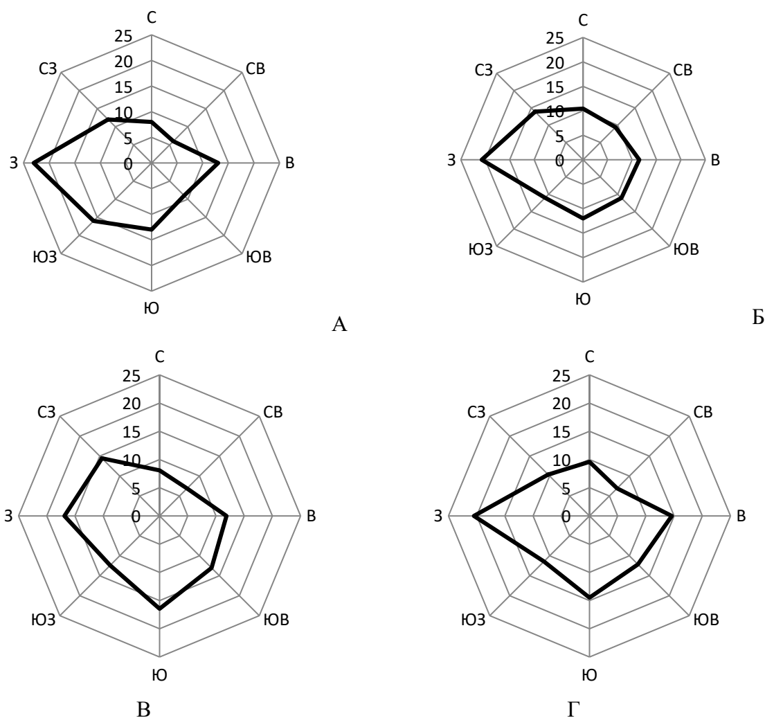
Рисунок 2.11 – Повторяемость различных направлений ветра по метеорологическим станциям: А – Брест, Б – Пинск, В – Василевичи, Г – Брагин
