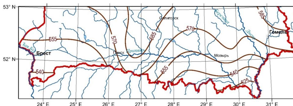
Рисунок 2.8 – Годовые нормы суммарного испарения на территории Белорусского Полесья, мм
