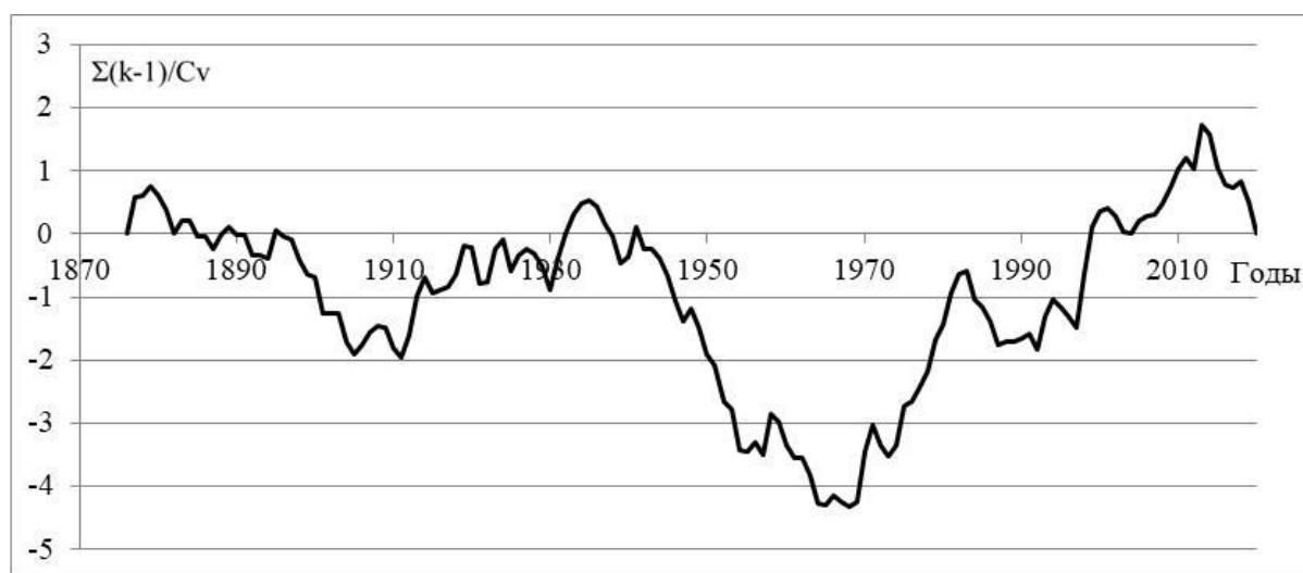
Рисунок 3.6 – Нормированная разностная интегральная кривая среднегодовых расходов воды р. Припять в створе г. Мозыря
