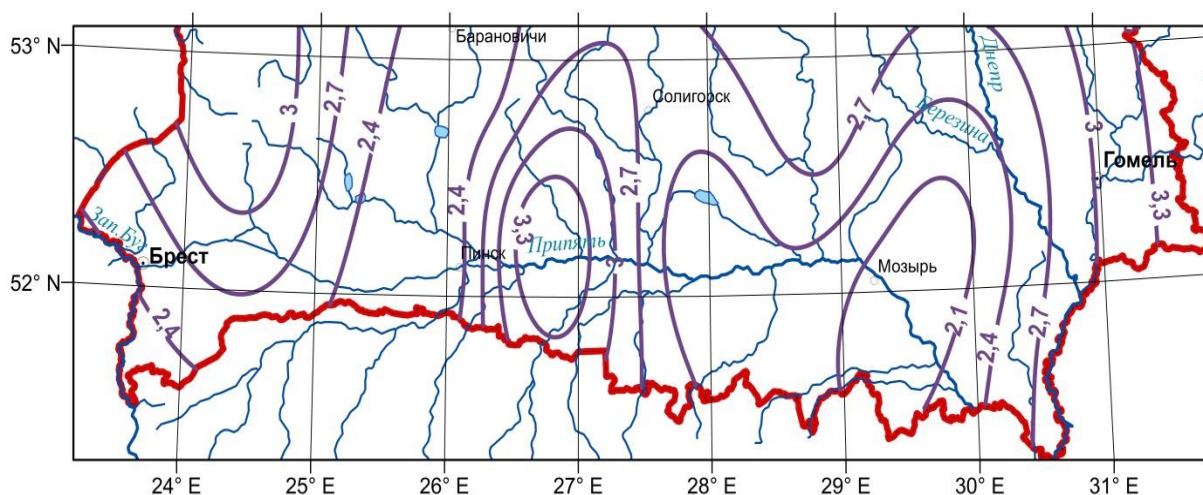
Рисунок 2.10 – Средняя скорость ветра Белорусского Полесья
