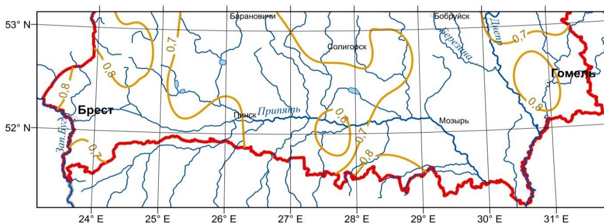
Рисунок 3.10 – Карта коэффициентов вариации максимального стока воды весеннего половодья рек Белорусского Полесья за период 1969–2020 гг.
