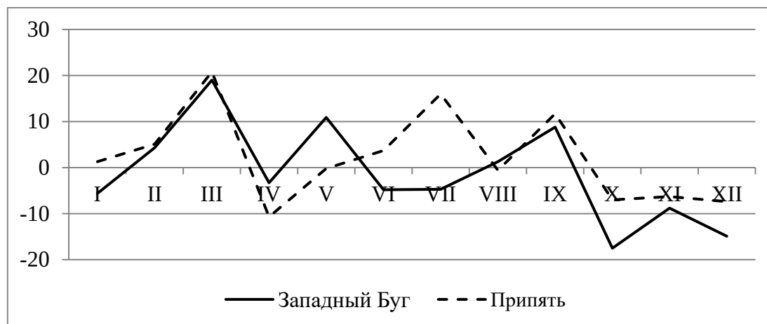
Рисунок 2.15 – Прогноз изменения месячного количества осадков (%) для Белорусского Полесья до 2035 г. (средняя величина за период 2021–2050 гг.)
