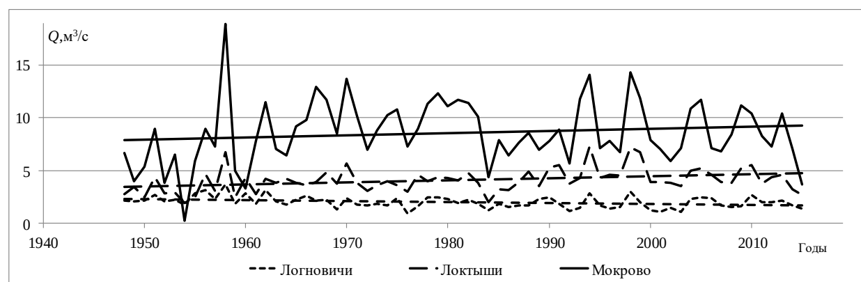
Рисунок 3.22 – Многолетний ход среднегодовых расходов воды р. Лань
