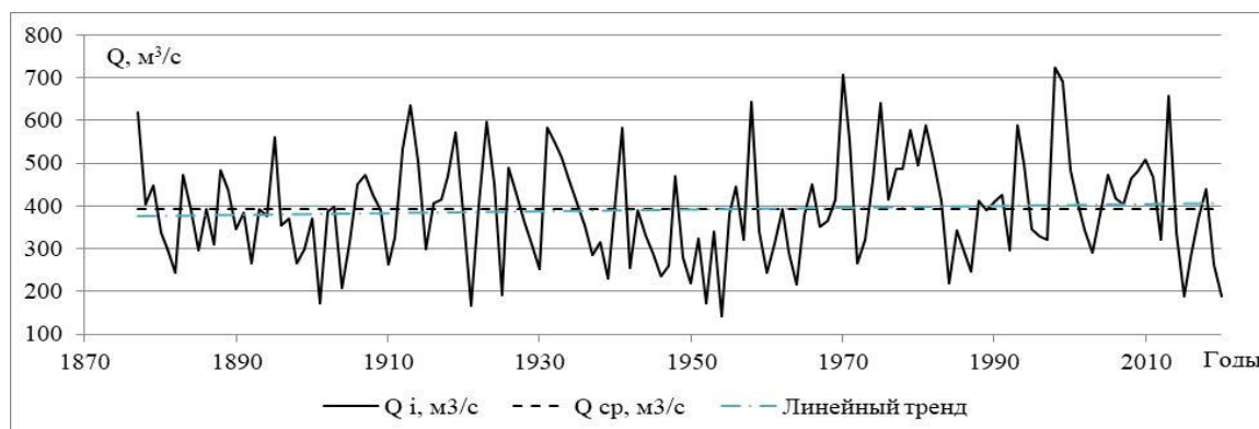
Рисунок 3.2 – Многолетний ход среднегодовых расходов воды р. Припять в створе г. Мозыря
