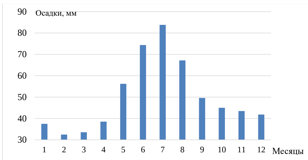
Рисунок 2.6 – Годовой ход осадков в пределах Белорусского Полесья
