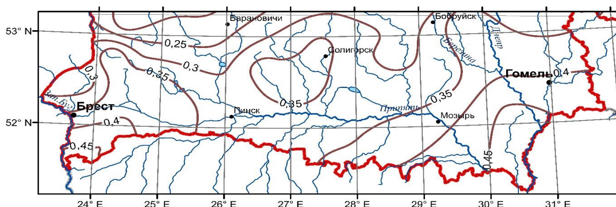
Рисунок 3.3 – Карта коэффициентов вариации среднего годового стока рек Полесья за период 1969–2020 гг.
