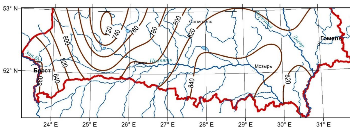
Рисунок 2.7 – Годовые нормы максимально возможного испарения на территории Белорусского Полесья, мм
