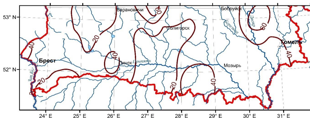
Рисунок 3.9 – Карта среднего максимального стока воды весеннего половодья рек Белорусского Полесья за период 1969–2020 гг., л/(с·км 2 )
