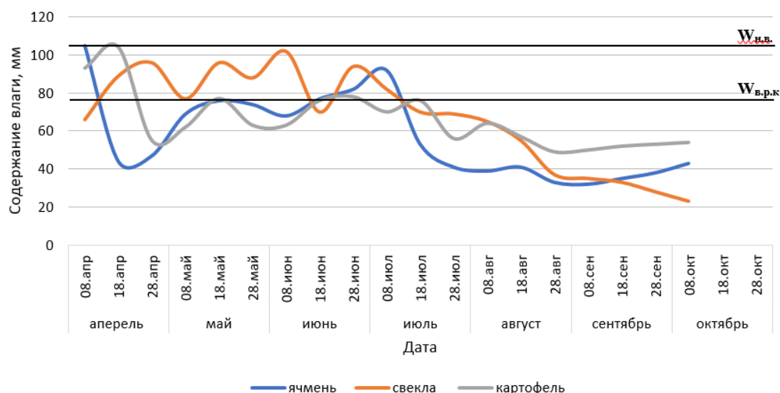
Рисунок 4.23 – Содержание продуктивных влагозапасов в почве
