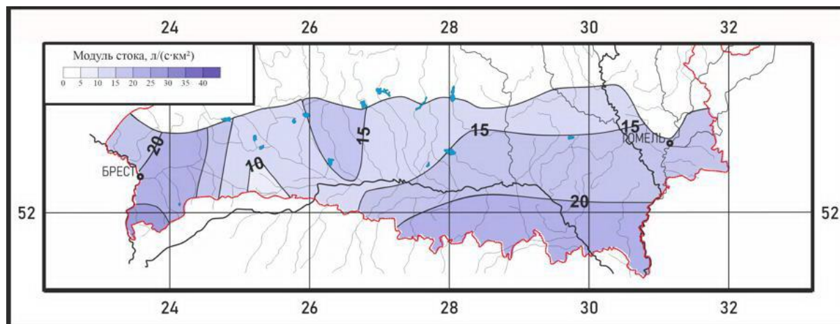
Рисунок 3.11 – Модули максимальных расходов воды дождевых паводков 10 %-ной обеспеченности
