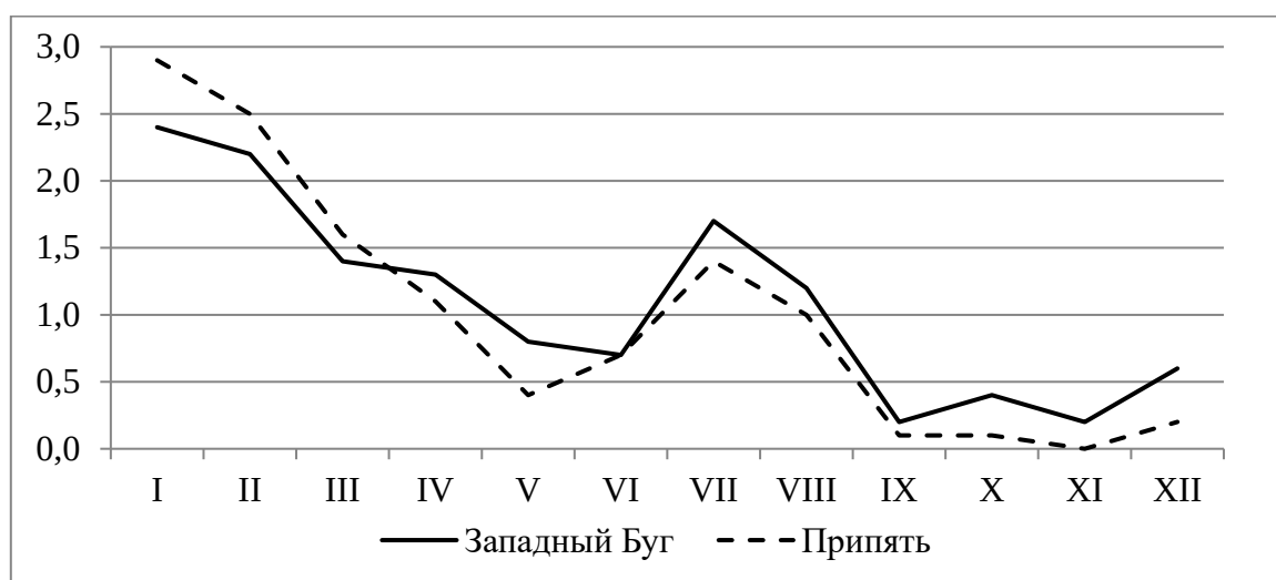
Рисунок 2.12 – Общая оценка изменения среднемесячной температуры воздуха (°C) в бассейнах рек Белорусского Полесья (1986–2010 гг.) – (1961–1985 гг.)
