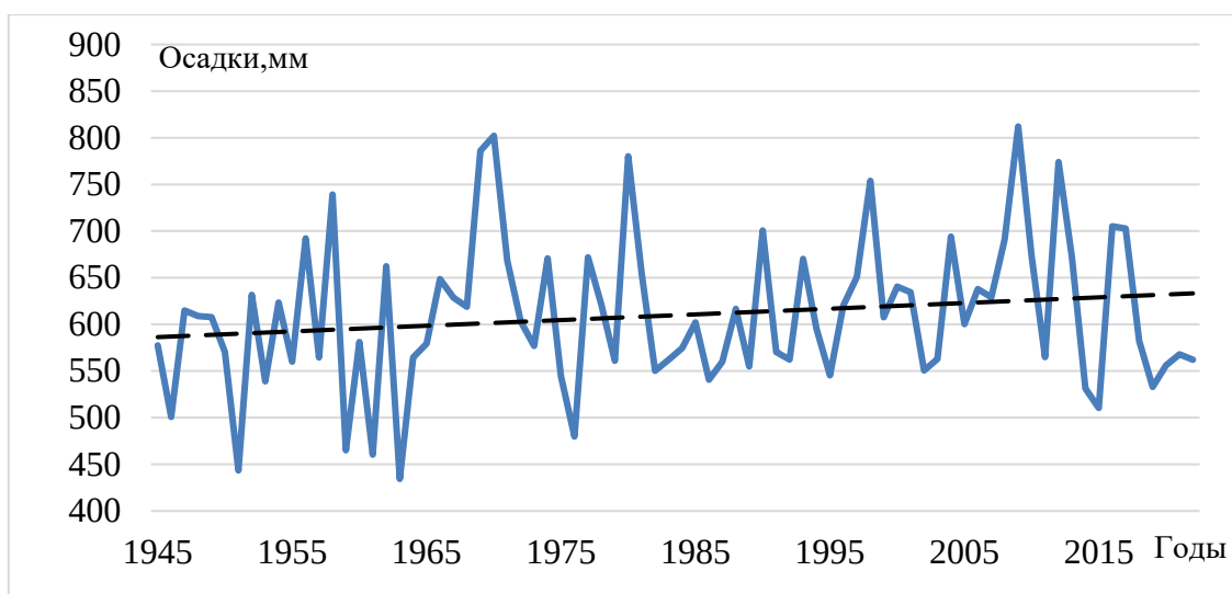
Рисунок 2.5 – Многолетние колебания годового количества осадков в пределах Белорусского Полесья за период 1945–2022 гг.
