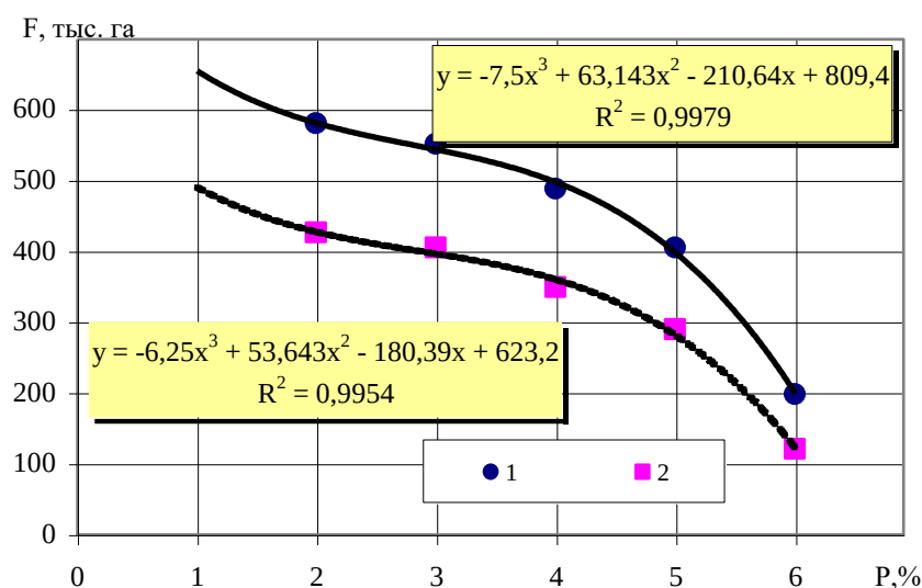
Рисунок 3.15 – Площади затопления поймы р. Припять в зависимости от обеспеченности уровня воды: 1 – всего по пойме; 2 – в пределах Беларуси
