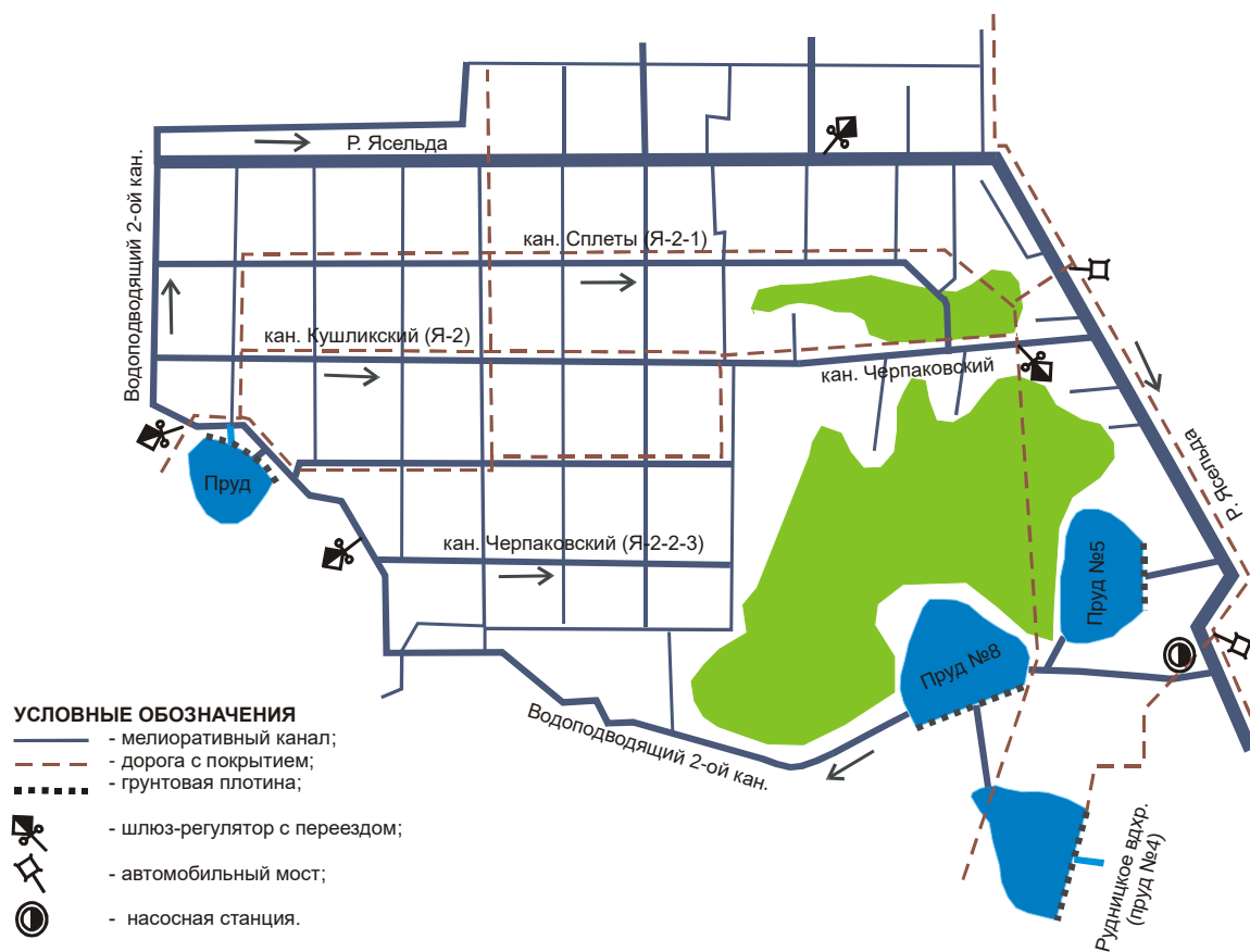
Рисунок 4.15 – Схема мелиорации земель на объекте «Верховье Ясельды»
