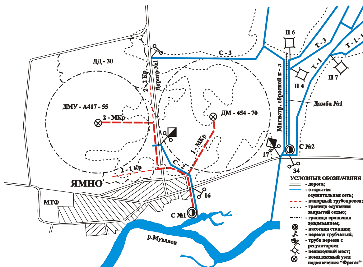
Рисунок 4.20 – Схема мелиоративной системы «Ямно» в совхозе «Брестский» Брестского района
