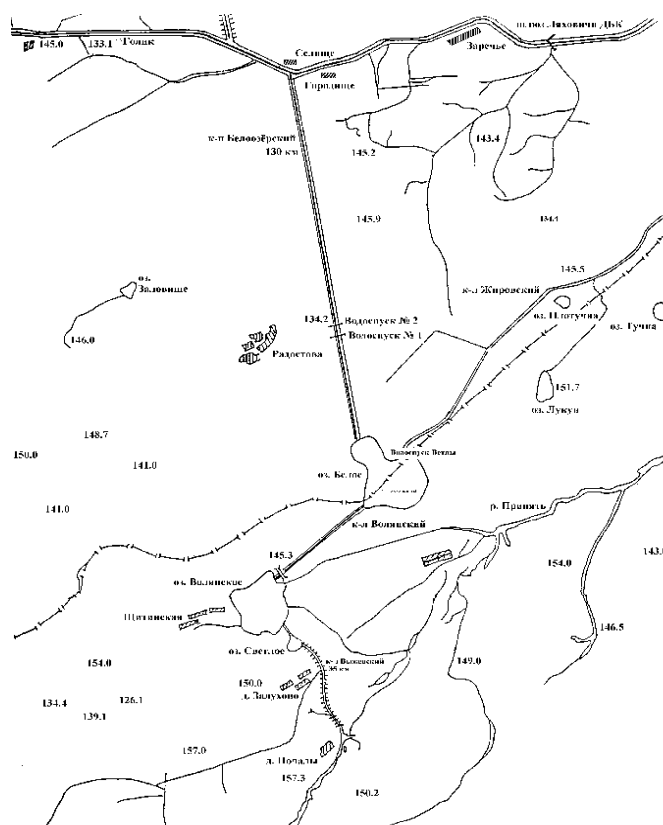
Рисунок 4.5 – Схема водного питания Днепровско-Бугского канала
