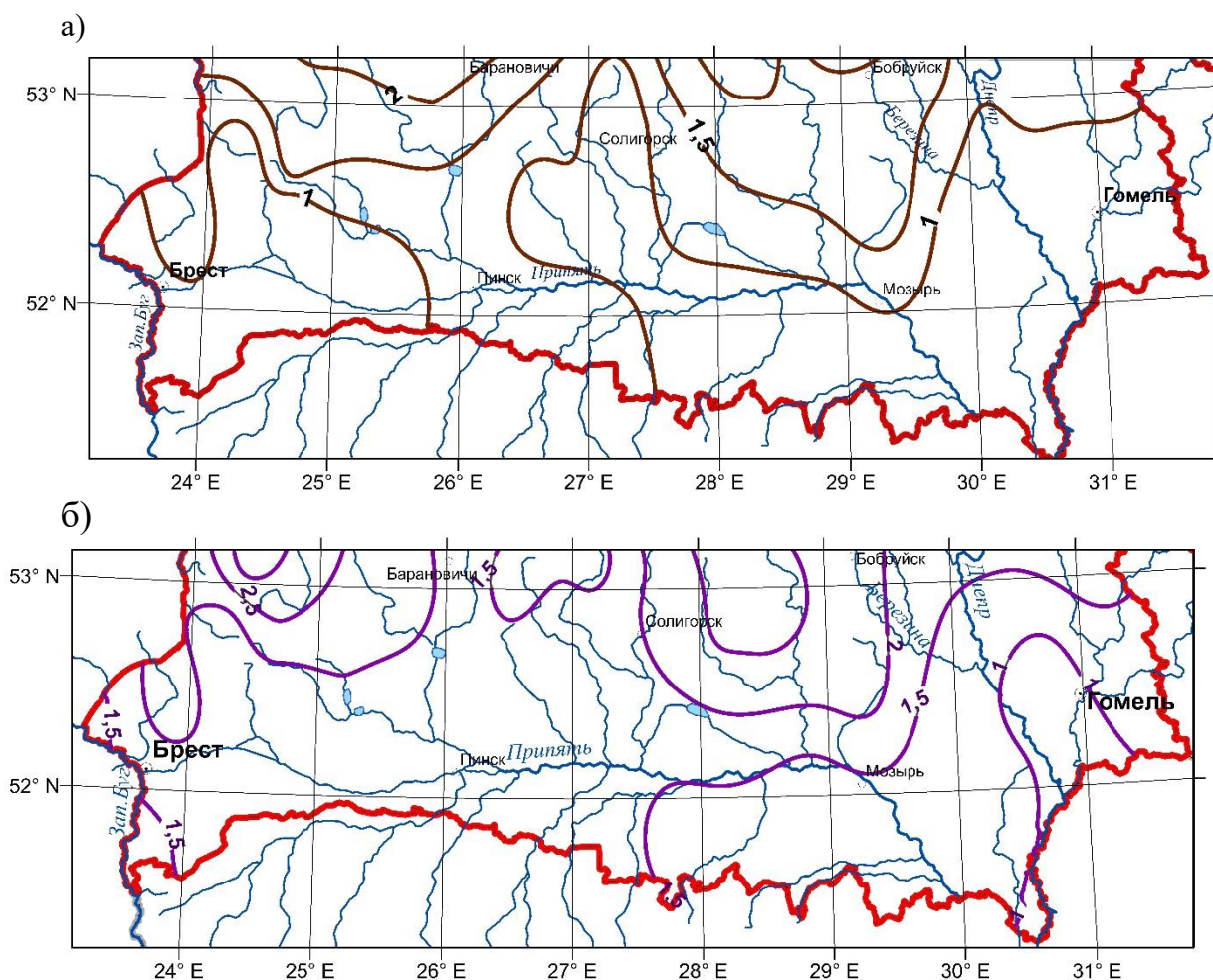
Рисунок 3.14 – Модуль минимального стока воды рек Беларуси: а) летне-осенняя межень; б) зимняя межень
