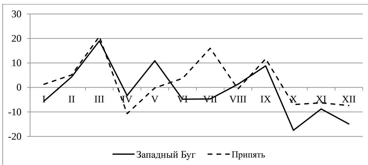
Рисунок 2.13 – Общая оценка изменения месячного количества осадков (%) в бассейнах рек Белорусского Полесья (1986–2010 гг.) – (1961–1985 гг.)
