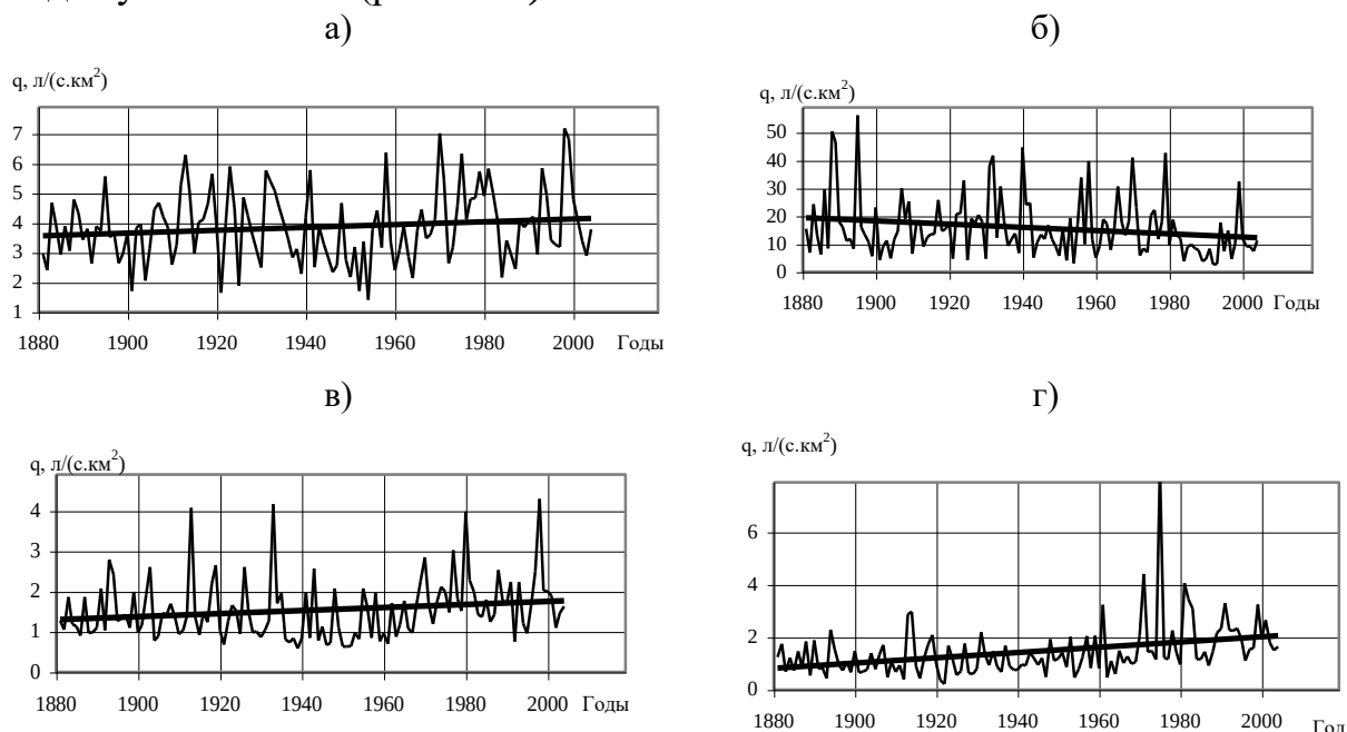
Рисунок 3.21 – Динамика модулей стока воды рек Полесья: а) годовых; б) максимальных весеннего половодья; в) минимальных летне-осенних; г) минимальных зимних
