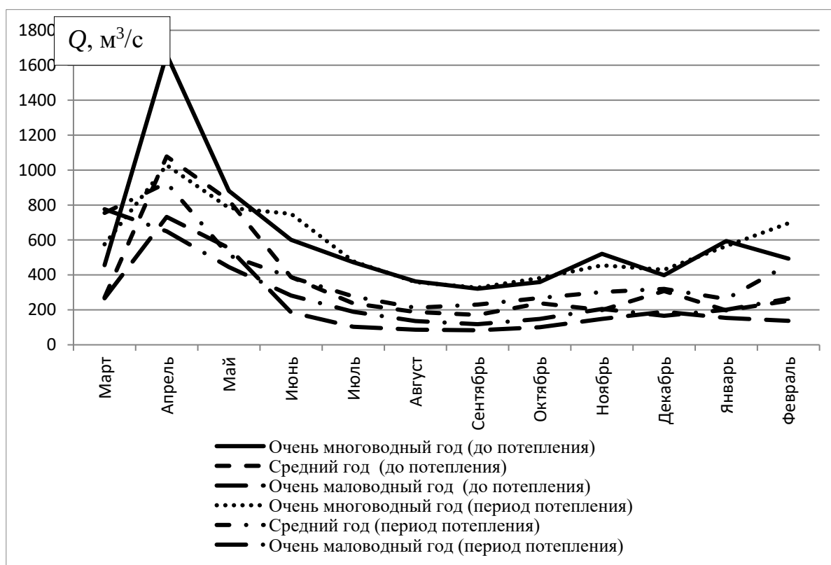
Рисунок 3.7 – Гидрографы стока воды р. Припять – г. Мозырь
