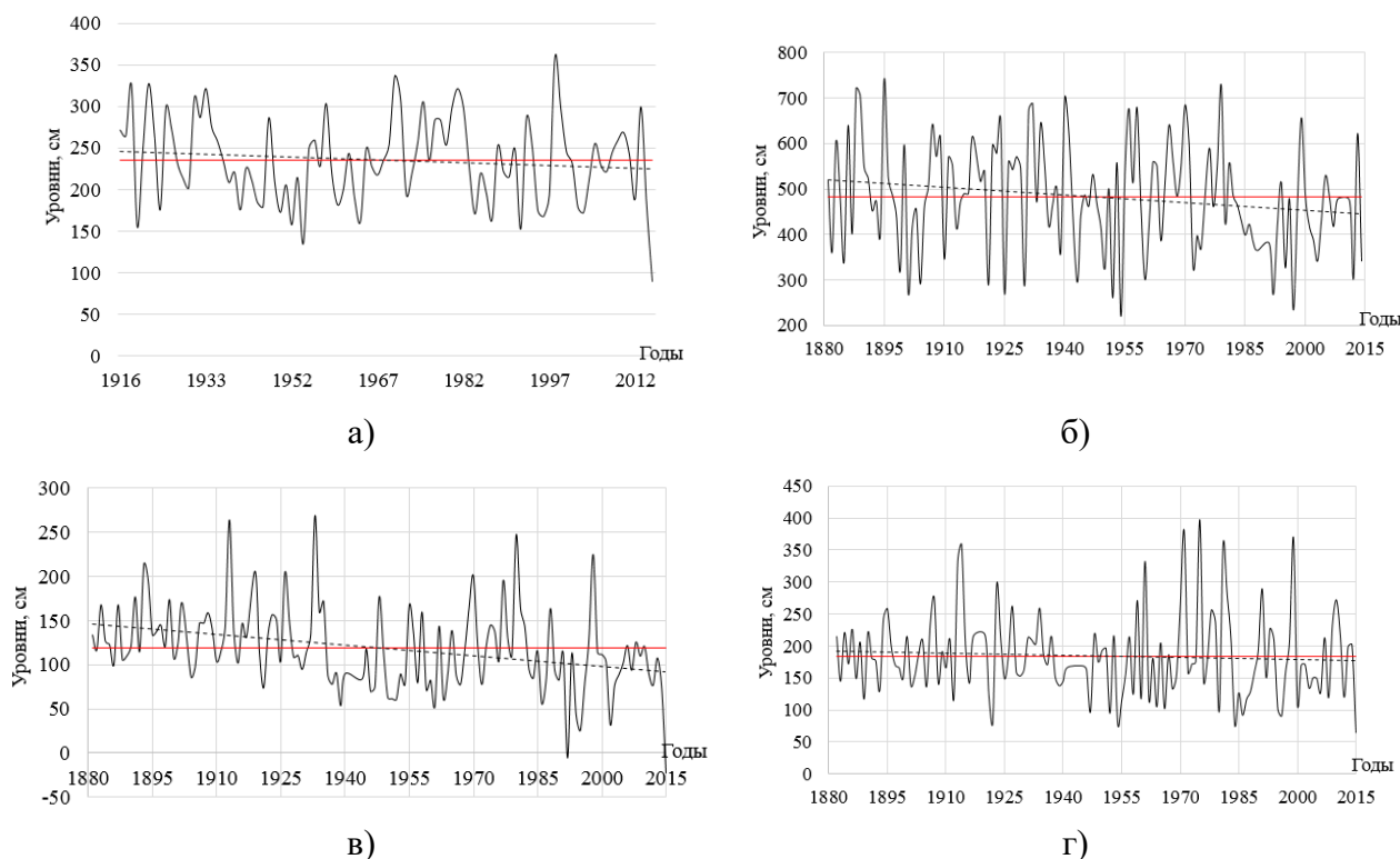
Рисунок 3.17 – Хронологический многолетний ход уровней воды р. Припять – г. Мозырь за период инструментальных наблюдений до 2015 г.: а) средних годовых; б) максимальных весеннего половодья; ----- в) минимальных периода открытого русла; г) минимальных зимнего периода черная линия – линия тренда; красная горизонтальная линия – средние значения уровней воды
