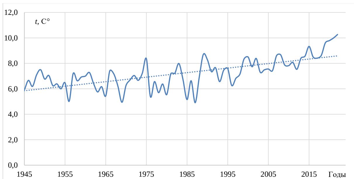
Рисунок 2.3 – Многолетние колебания средней годовой температуры воздуха в пределах Белорусского Полесья
