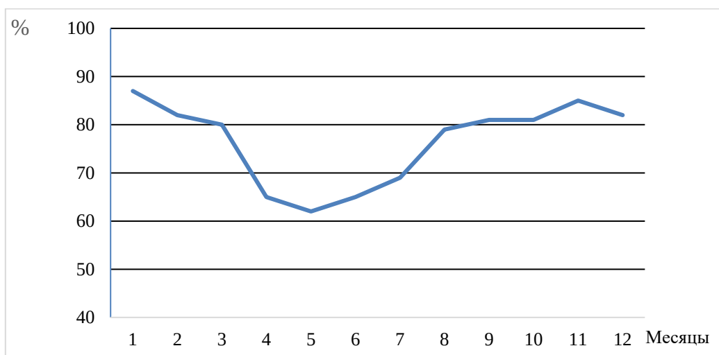
Рисунок 2.1 – Годовой ход относительной влажности воздуха Белорусского Полесья
