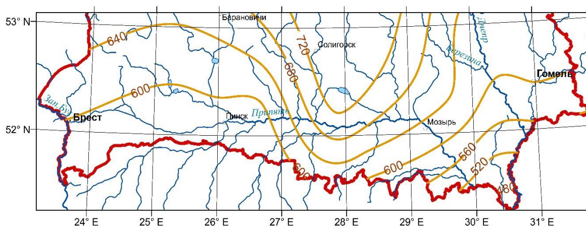
Рисунок 2.4 – Распределение годовых атмосферных осадков по территории Белорусского Полесья, мм
