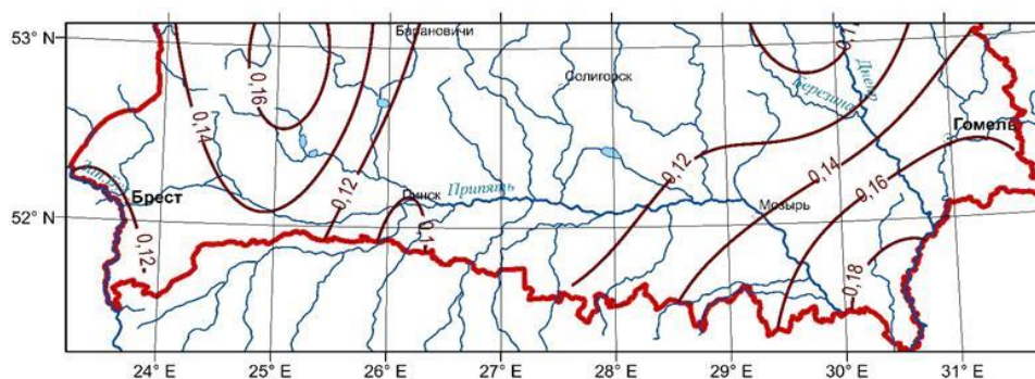
Рисунок 2.9 – Пространственная структура коэффициентов суммарного испарения на территории Белорусского Полесья
