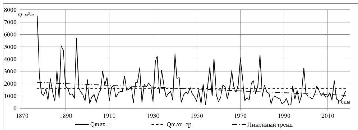
Рисунок 3.8 – Хронологический ход максимальных расходов воды весеннего половодья р. Припяти в створе г. Мозыря
