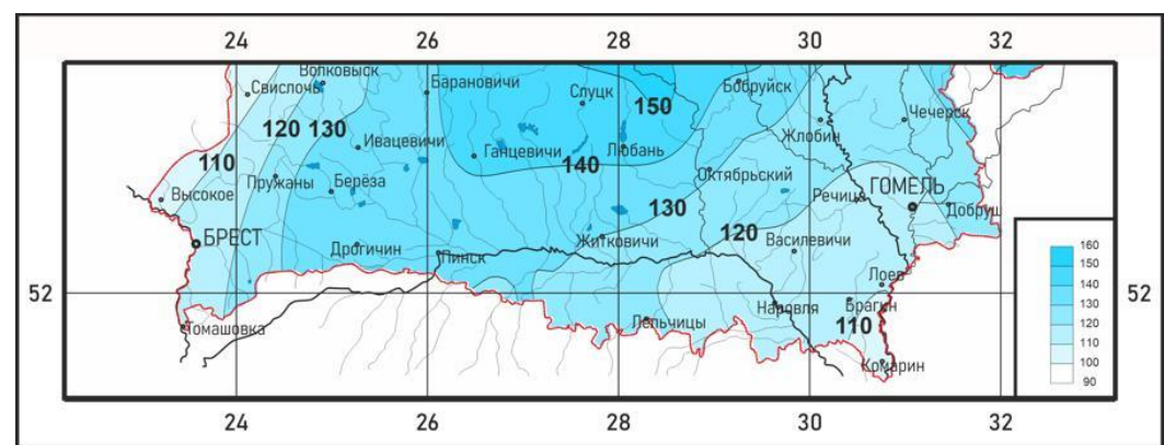
Рисунок 3.16 – Пространственная структура средних значений уровней воды за период инструментальных наблюдений в абсолютных отметках: а) средних годовых; б) максимальных весеннего половодья; в) минимальных периода открытого русла; г) минимальных зимнего периода
