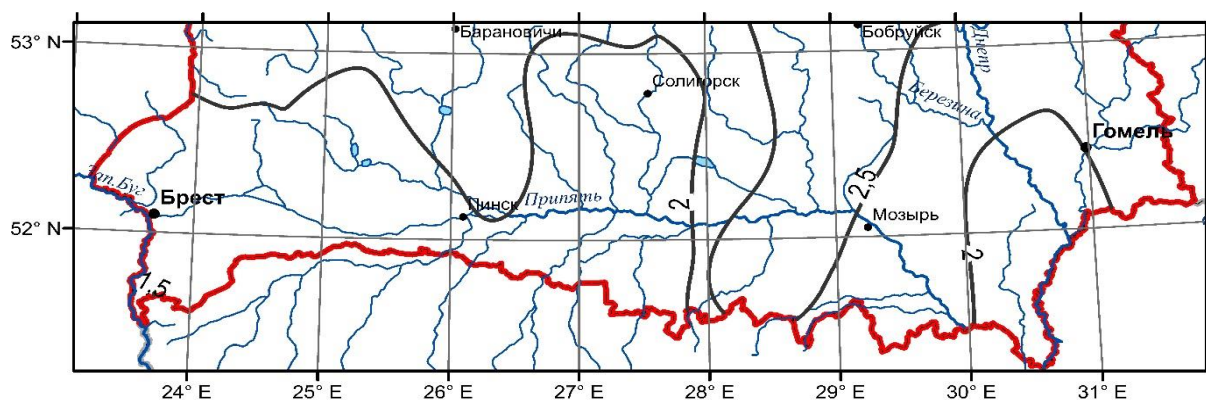
Рисунок 3.4 – Карта среднего годового поверхностного стока рек Полесья за период 1969–2020 гг., л/(с·км 2 )
