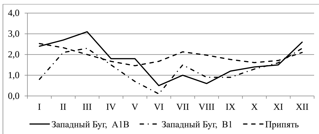
Рисунок 2.14 – Прогноз изменения среднемесячной температуры воздуха (°C) для рек Белорусского Полесья до 2035 г. (средняя величина за период 2021–2050 гг.)
