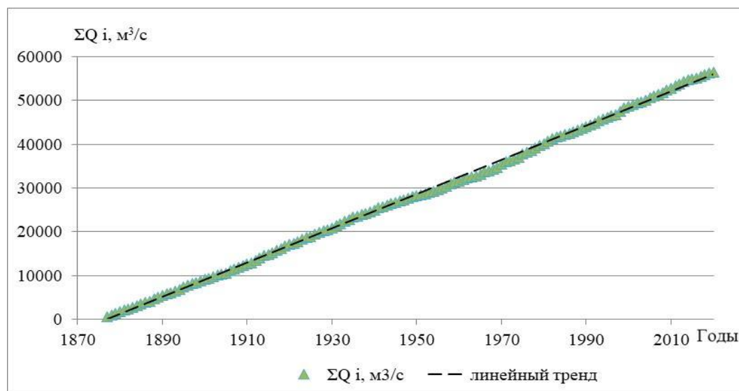
Рисунок 3.5 – Суммарная интегральная кривая среднегодовых расходов воды р. Припять в створе г. Мозыря
