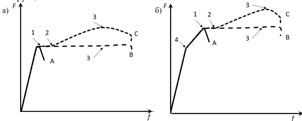
Рисунок 1 – Обобщенные идеализированные кривые деформирования стального элемента
