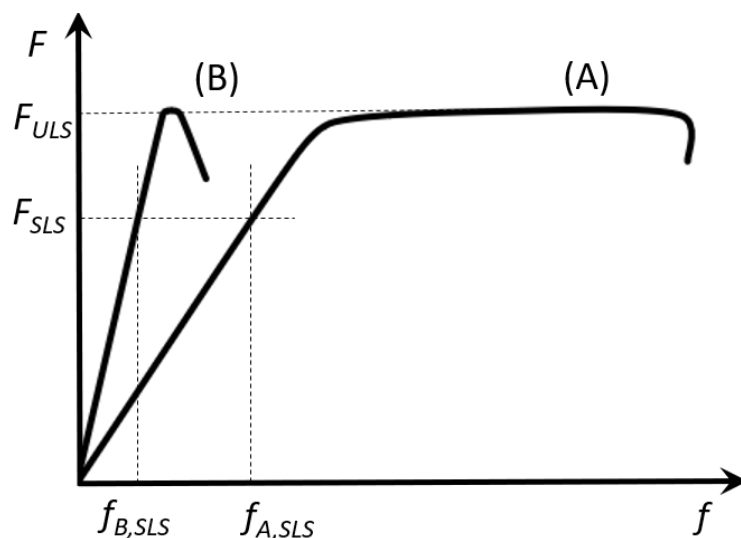
Рисунок 2 – Кривые деформирования в зависимости от класса сечения
