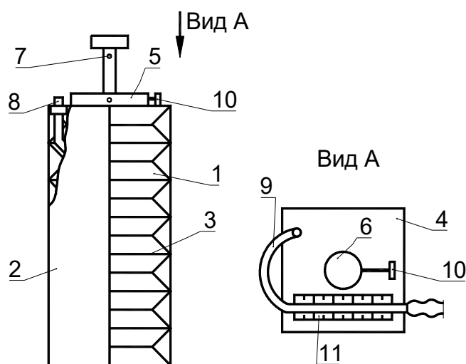
1 – сильфон; 2 – корпус; 3 – распорное кольцо; 4 – верхняя плита; 5 – неподвижная втулка; 6 – шток; 7 – углубления; 8 – штуцер; 9 – резиновая трубка; 10 – винт фиксирования; 11 – шкала Рисунок 4.1 – Газоанализатор типа УГ-2
