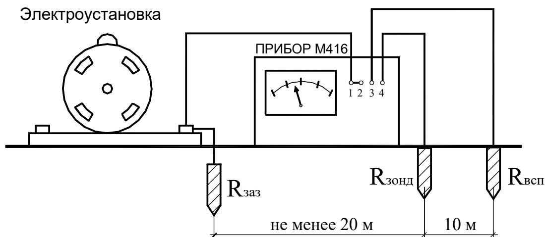
Рисунок 6.1 – Принципиальная схема соединений при измерении сопротивления заземляющего устройства
