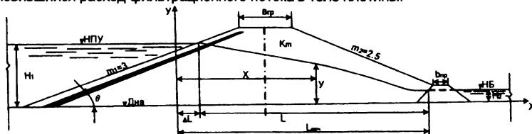
Рисунок 11. Расчетная схема к фильтрационному расчету
