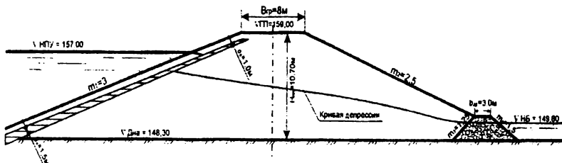
Рисунок 12. Поперечный профиль запроектированной грунтовой плотины
