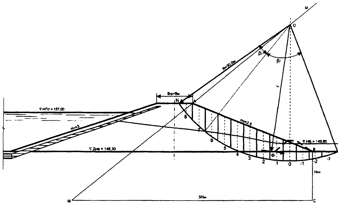
Рисунок 13. Расчетная схема к статическому расчету низового откоса плотины
