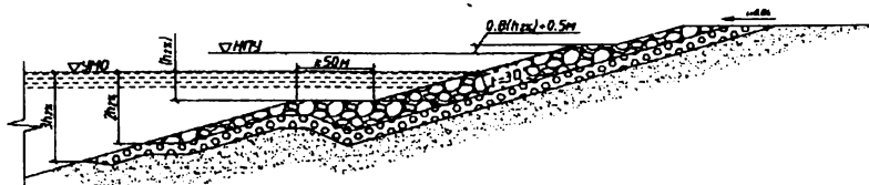
Рисунок 8. Крепление откоса каменным мощением
