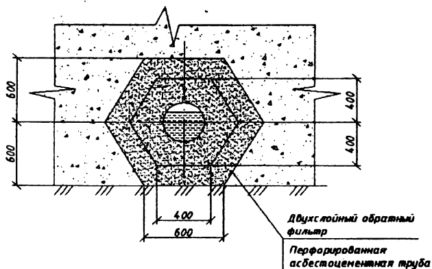
Рисунок 10. Трубчатый дренаж
