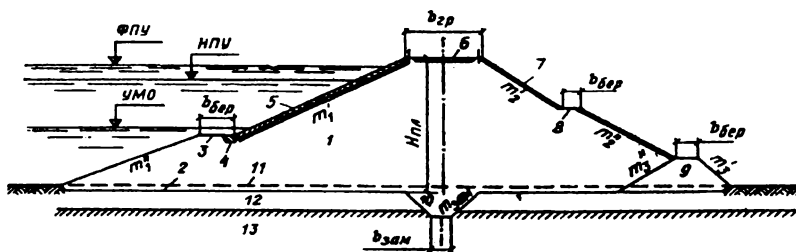
Рисунок 2. Поперечный профиль грунтовой плотины:
