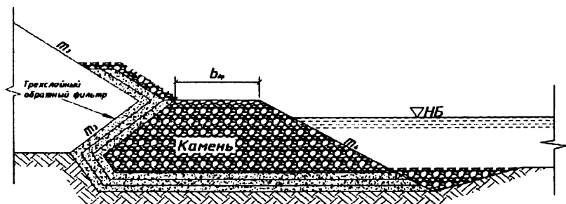
Рисунок 9. Дренажная призма
