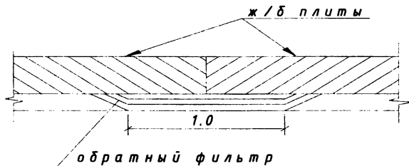
Рисунок 7. Элемент крепления откоса железобетонными плитами
