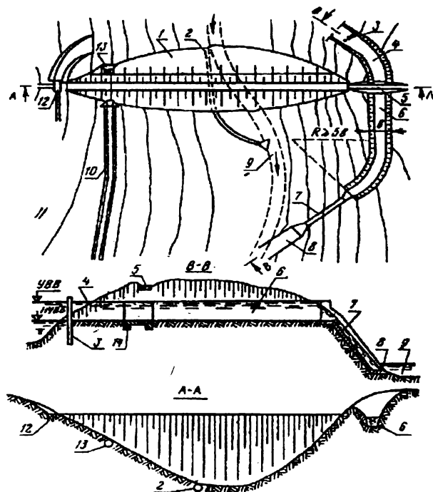
Рисунок 1. Водохранилищный гидроузел:
