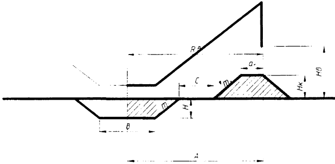
Рисунок 1 – 1) R_b \geq A ; 2) H_b \geq H_k ; 3) H_p \geq H ; 4) b \geq 1,5b_k
