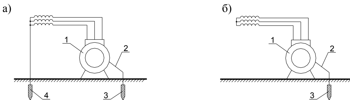
Рисунок 1 – Принципиальные схемы защитного заземления
