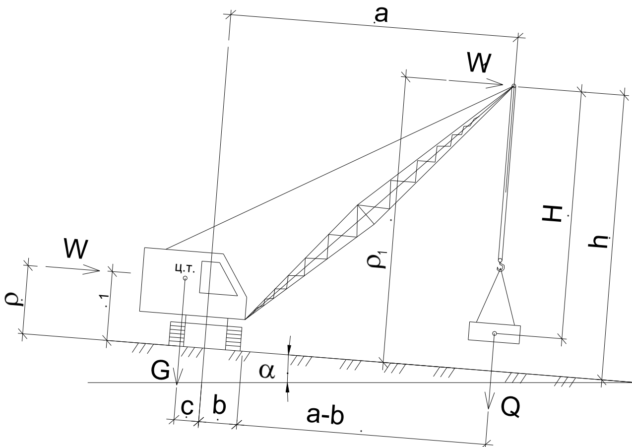
Рисунок 2 – Расчётная схема грузовой устойчивости самоходного крана
