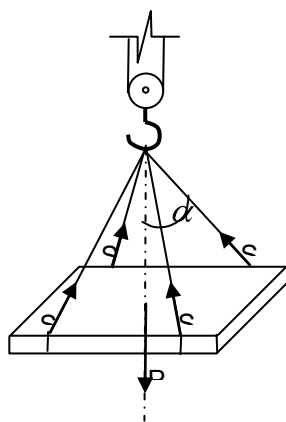
Рисунок 3 – Расчётная схема гибких строп
