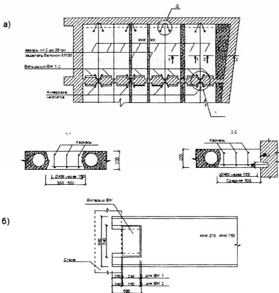
а) схема раскладки панелей, б) пример укладки вкладыша Рисунок 5.3 – Устройство междуэтажных перекрытий с укладкой панелей на выпускные ребра в пробытие в стенах гнезда и борозды (размеры гнезд для заводки выпускных ребер панелей д.б. не более 300 мм; пробытие сплошных борозд для заводки выпускных ребер панелей не допускается)
