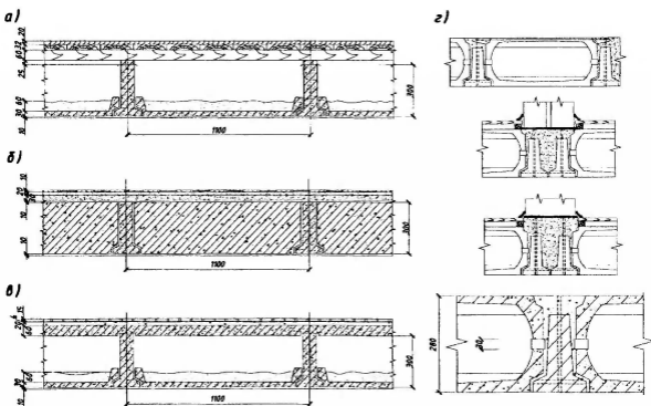
а) с нижним вкладышем; б) с вкладышем из легкого бетона; в) с двумя вкладышами; г) с вкладышами сводчатого очертания
