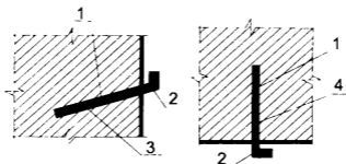
1-анкер,2-арматура,3-раствор цемента,4-бетон
