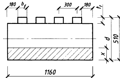
Рисунок 15.3 – К расчету усиления элементами СВА
