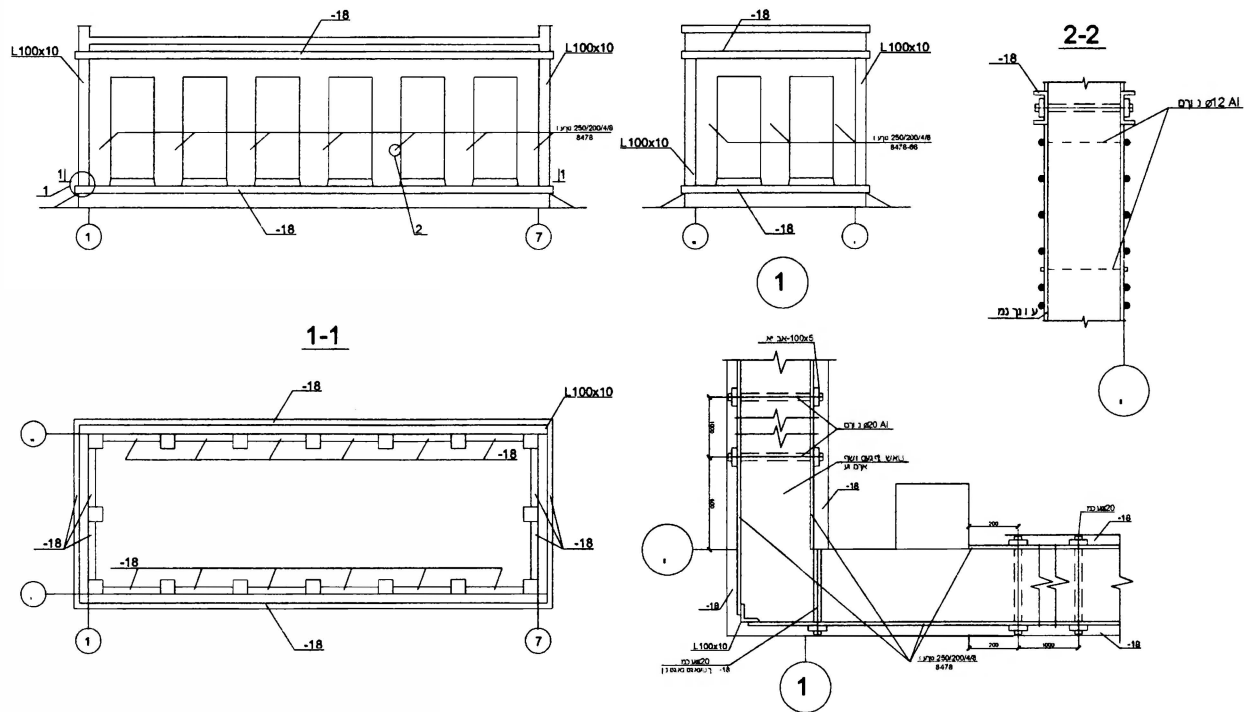
Рисунок 14.4 – Усиление стен металлическими поясами
