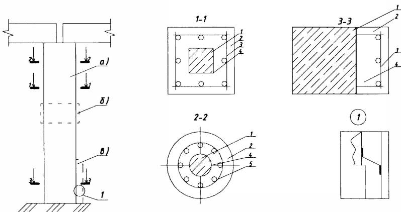
1 – усиливаемая конструкция; 2 – бетон обоймы; 3 – арматурные каркасы; 4 – подготовленная поверхность; 5 – спиральная арматура; 6 – отгиб Рисунок 7.1 – Усиление железобетонной колонны обоймой на всю высоту (а), на участке (б), при одностороннем наращивании сечения (в)
