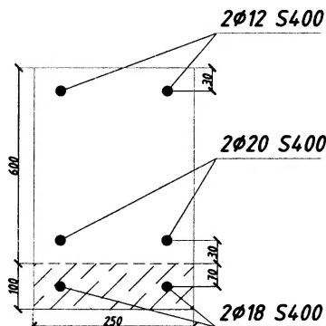
Рисунок 5.5 – К расчету усиления растянутой зоны приваркой дополнительной арматуры
