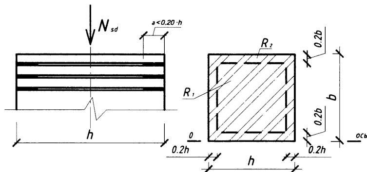
Рисунок 15.4 – К расчету усиления полимерцементным раствором
