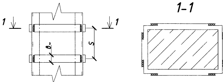
Рисунок 7.5 – К расчету усиления ободной из металла
