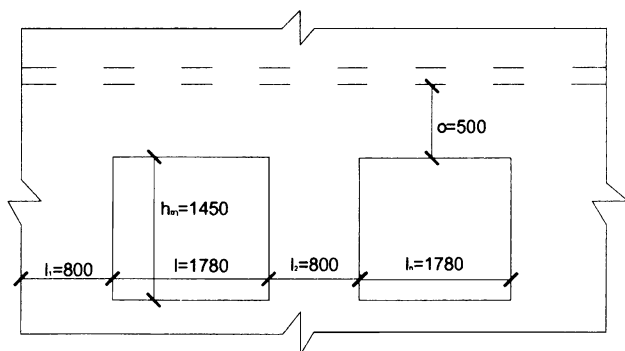
Рисунок 13.3 – К расчёту перемычек по примеру
