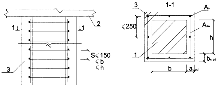
Рисунок 12.3 – Усиление кирпичного столба армированной обоймой
