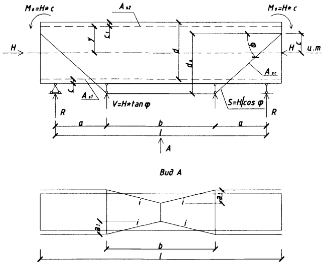
Рисунок 9.4 – К расчету шпренгельной затыжки
