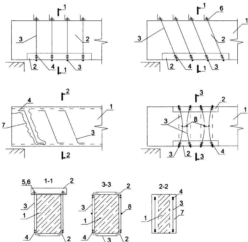
1 – усиливаемая конструкция, 2 – уголок, 3 - хомуты усиления, 4 – сварка, 5 – шайба с гайкой, 6 – косая гайка, 7 – борозда, 8 – стяжное устройство или скоба Рисунок 6.5 – Усиление наклонного сечения
