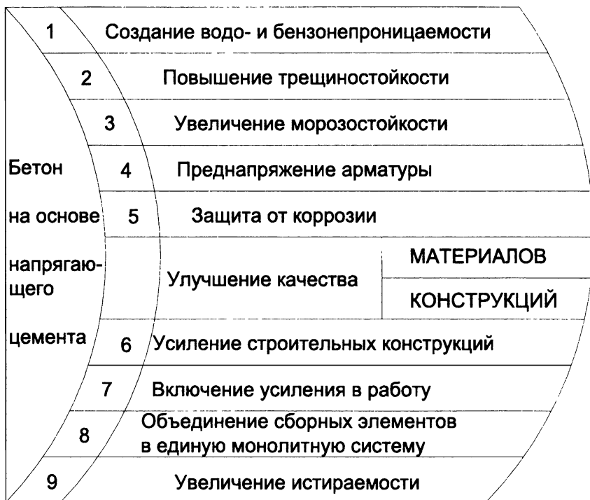
Рисунок 8.2 – Эффект применения напрягающего бетона
