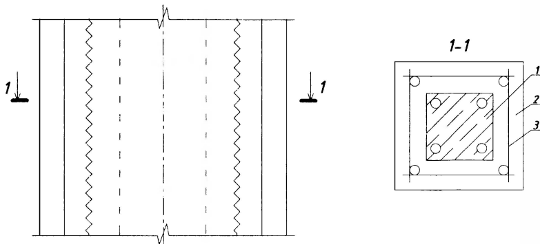
1 – усиливаемый элемент; 2 – бетон обоймы; 3 – арматура обоймы Рисунок 7.2 – К расчету усиления обоймой из железобетона
