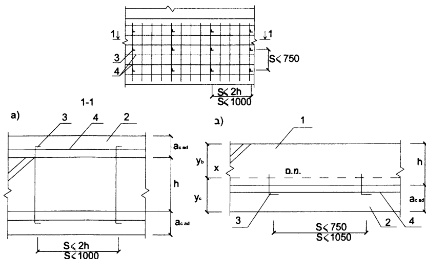
1 – усиливаемая стена; 2 – наращивание; 3 – анкера (связи); 4 – сетка Рисунок 12.4 – Усиление кирпичной стены наращиванием с двух сторон (а) и с одной стороны (б)
