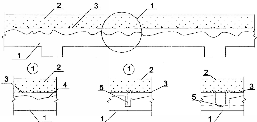
1 – усиливаемая конструкция; 2 – бетон усиления; 3 – арматура усиления; 4 – контактный шов; 5 – анкер Рисунок 6.2 – Усиление наращиванием сечения сверху
