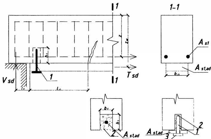
Рисунок 5.4 – К расчету прочности контактного шва
