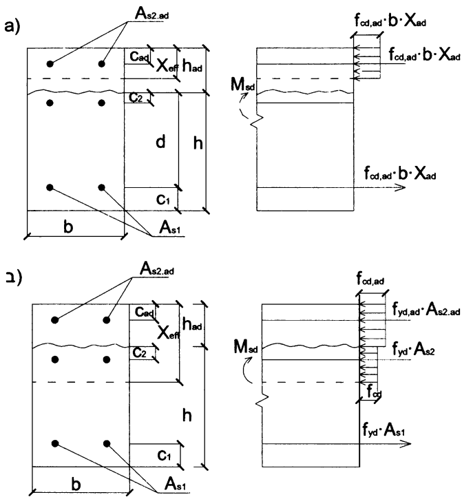
Рисунок 6.3 – Схема усилий в нормальном сечении после наращивания
