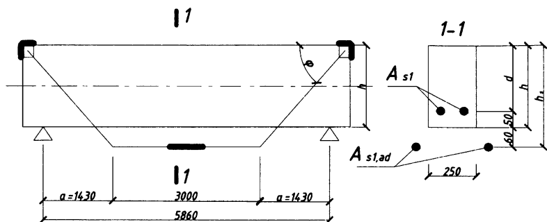
Рисунок 9.5 – К расчету шпренгельной затяжки
