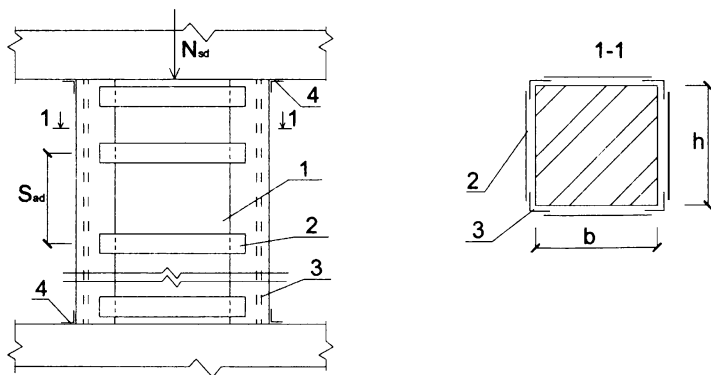
1 – столб, 2 – планки 3 – уголок, 4 – опорный уголок Рисунок 12.2 – Усиление кирпичного столба обоймой из металла
