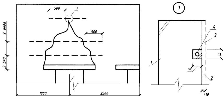
1 – кирпичная кладка; 2 – штукатурка; 3 – раствор Sure Ggrout; 4 – анкерный стержень Sure Twist
