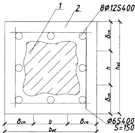
Рисунок 7.3 – К расчету усиления обоймой из железобетона
