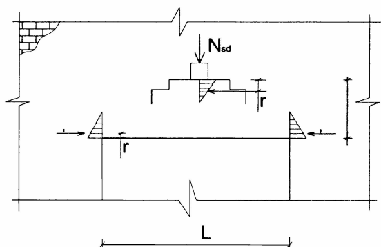
Рисунок 13.2 – К расчёту перемычек
