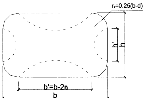
Рисунок 10.3 – Положение активных зон при усилении прямоугольных сечений колонн
