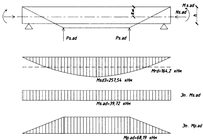
Рисунок 9.6 – К расчету шпренгельной затяжки
