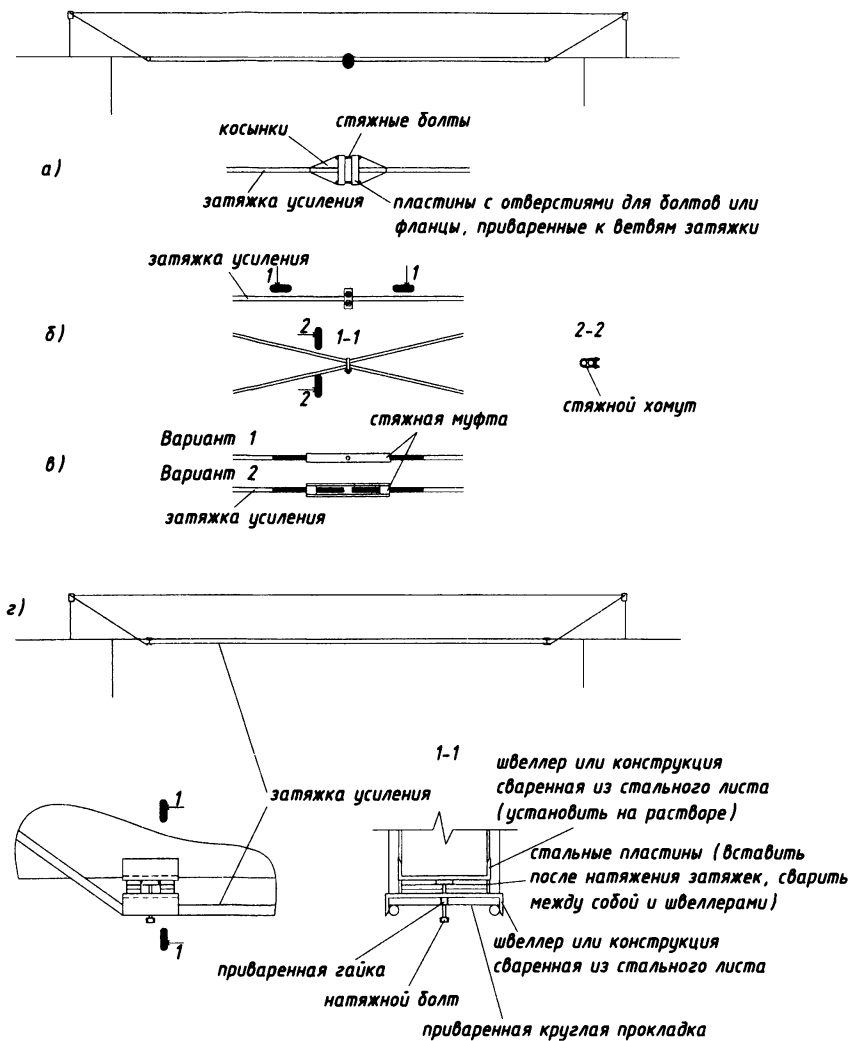
а) со стяжными болтами; б) стягиванием хомутов; в) с использованием муфт; г) с использованием болтов Рисунок 9.2 – Усиление изгибаемых элементов затяжкой
