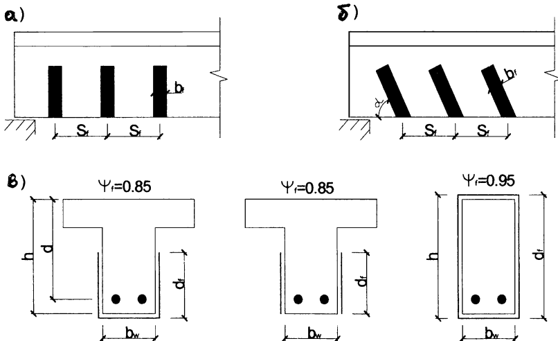
Рисунок 10.3 – Расположение ФАП хомутов при усилении наклонного сечения
