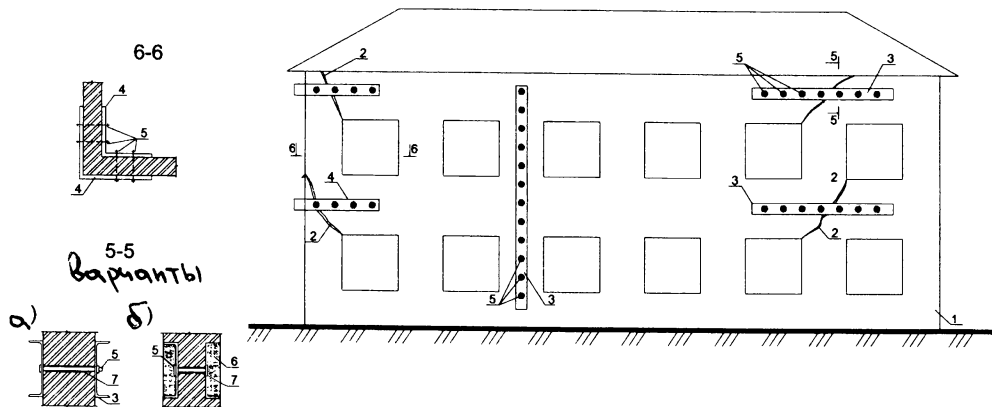
1 – деформированное здание; 2 – трещины в стенах здания; 3 – накладки из швеллеров; 4 – накладки из металлических пластин; 5 – стяжные болты; 6 – штроба для установки накладок, заделываемая раствором; 7 – отверстие в стенах для болтов (после установки болтов зачеканить раствором) Рисунок 14.3 – Установка напряженных поясов с наружной стороны здания
