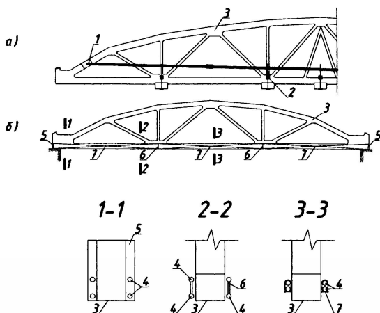
а) шарнирно-стержневая цепь; б) преднапряжённой затяжкой из арматуры 1-шарнирно-стержневая цепь; 2-натяжные подвески; 3-усиливаемая ферма; 4-затяжка из арматуры; 5-торцевой упорный лист; 6-распорка; 7-стяжной хомут Рисунок 9.3 – Усиление стропильных ферм
