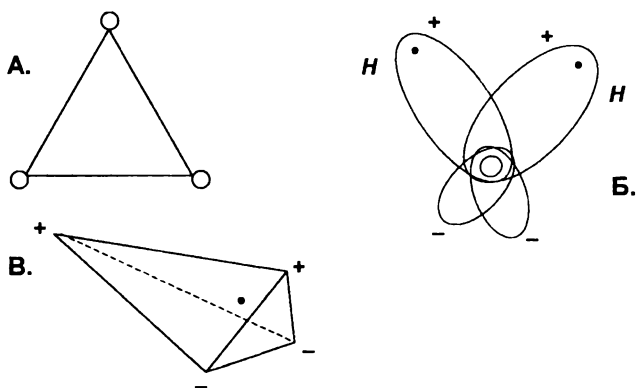
Рис. Строение молекулы воды
