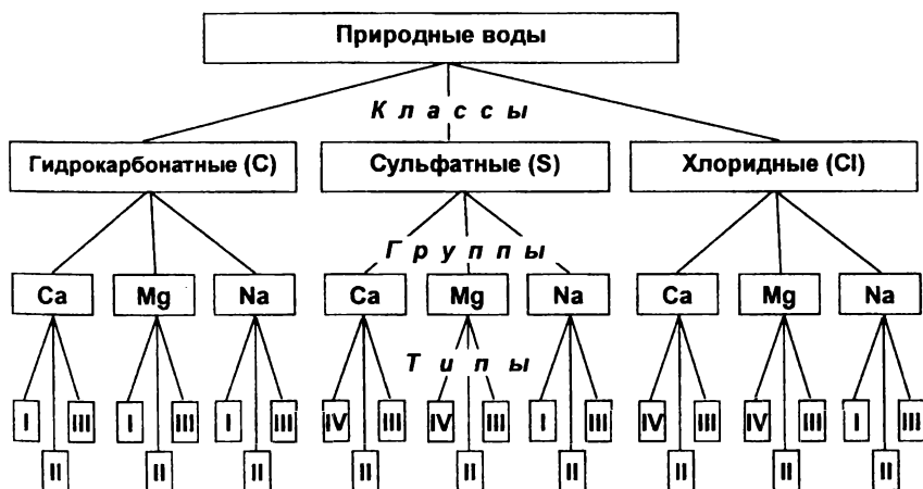
Схема классификации природных вод по преобладающему аниону и катиону и соотношению между главными ионами (по О. А. Алекину)
