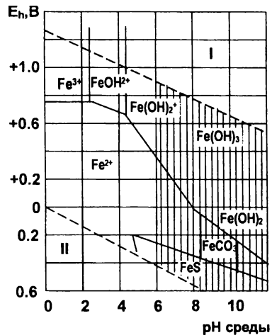
Рис. Окислительно-восстановительный потенциал системы «железо-вода» в окислительной (I) и восстановительной (II) средах
