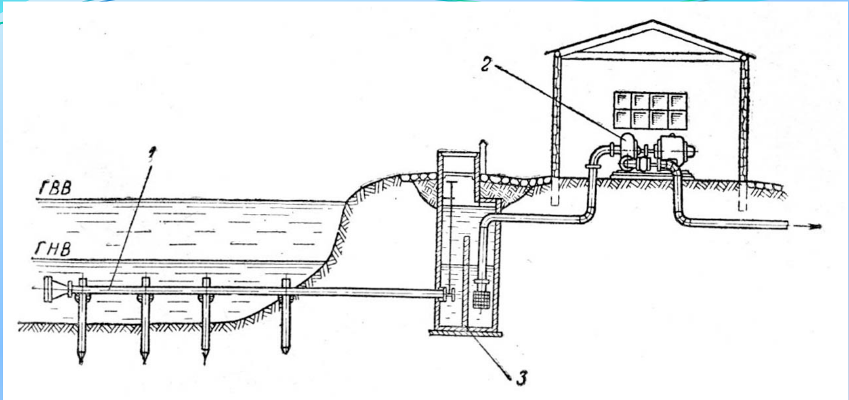
Рисунок 3 - Русловой водоприемник
