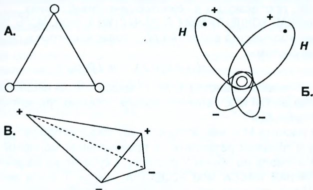
Рисунок – Строение молекулы воды
