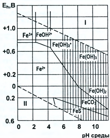
Рисунок – Окислительно-восстановительный потенциал системы «железо-вода» в окислительной (I) и восстановительной (II) средах
