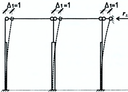
Рисунок 3.5 — Расчетная схема поперечной рамы
