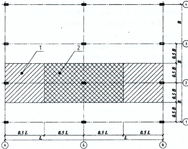
1 – грузовая площадь крайней колонны, 2 – грузовая площадь колонны среднего ряда Рисунок 3.1 – К определению нагрузок на поперечную раму
