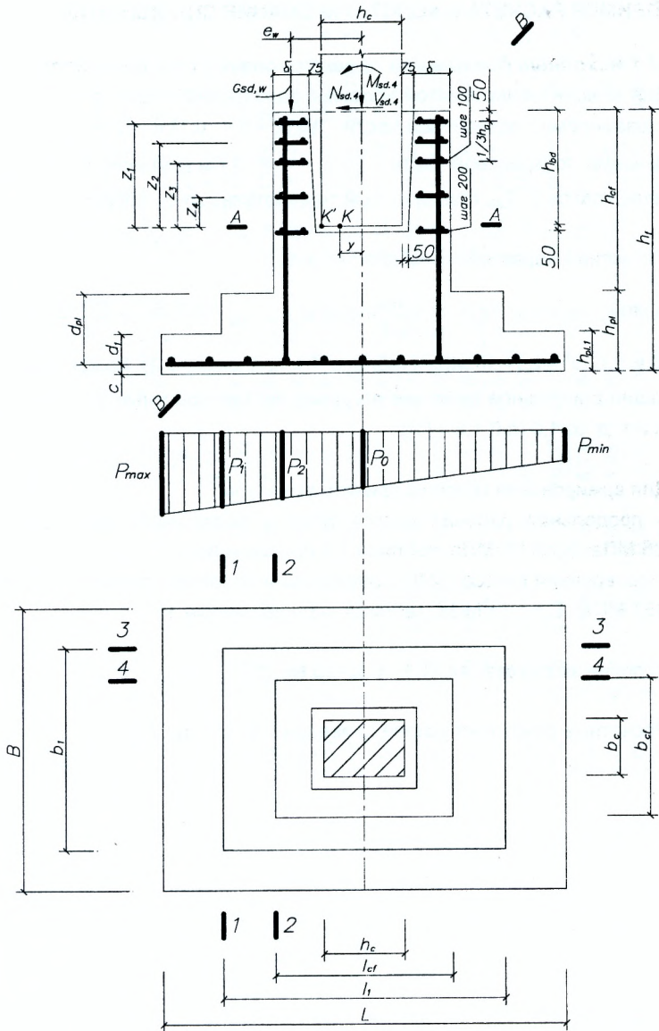
Рисунок 6.2 – К расчету и армированию фундамента
