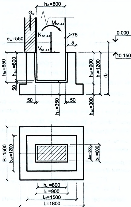
Рисунок 8.1 – Конструкция фундамента под крайнюю колонну
