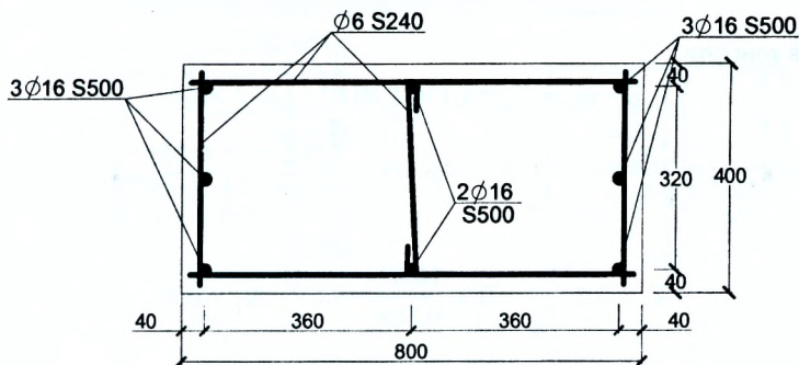
Рисунок 7.2 – Армирование сечения подкрановой части колонны
