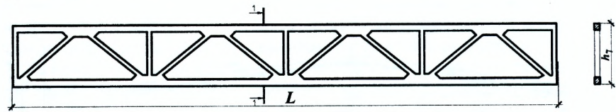
а) сегментная раскосная, б) арочная безраскосная, в) с параллельными поясами Рисунок 2.6 – Общий вид и сечение железобетонных ферм
