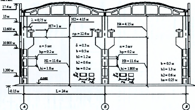
Рисунок 4.8 — Общий вид исходных данных в программе RAMAGB 2014
