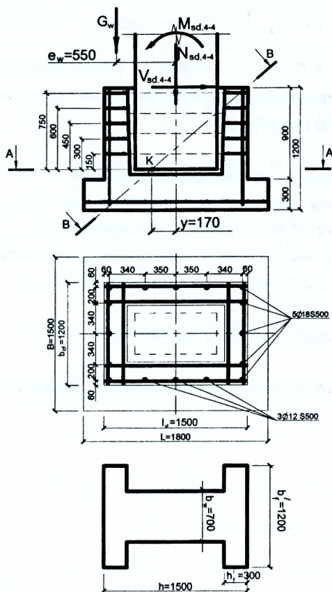
Рисунок 8.4 – К расчету подколонника фундамента
