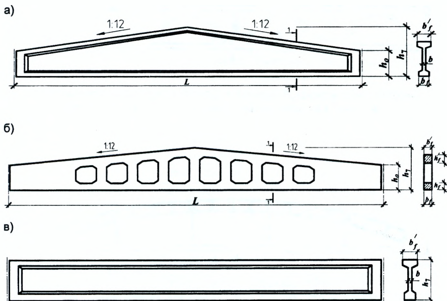
Рисунок 2.5 – Общий вид и сечение железобетонных стропильных балок
