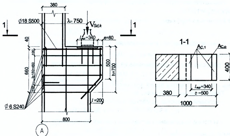
Рисунок 7.3 – Конструирование консоли колонны
