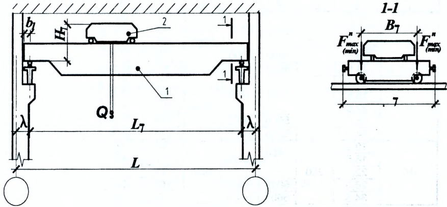
1 – мост кран, 2 – тележка
