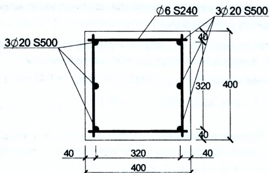
Рисунок 9.1 – Армирование сечения надкрановой части колонн
