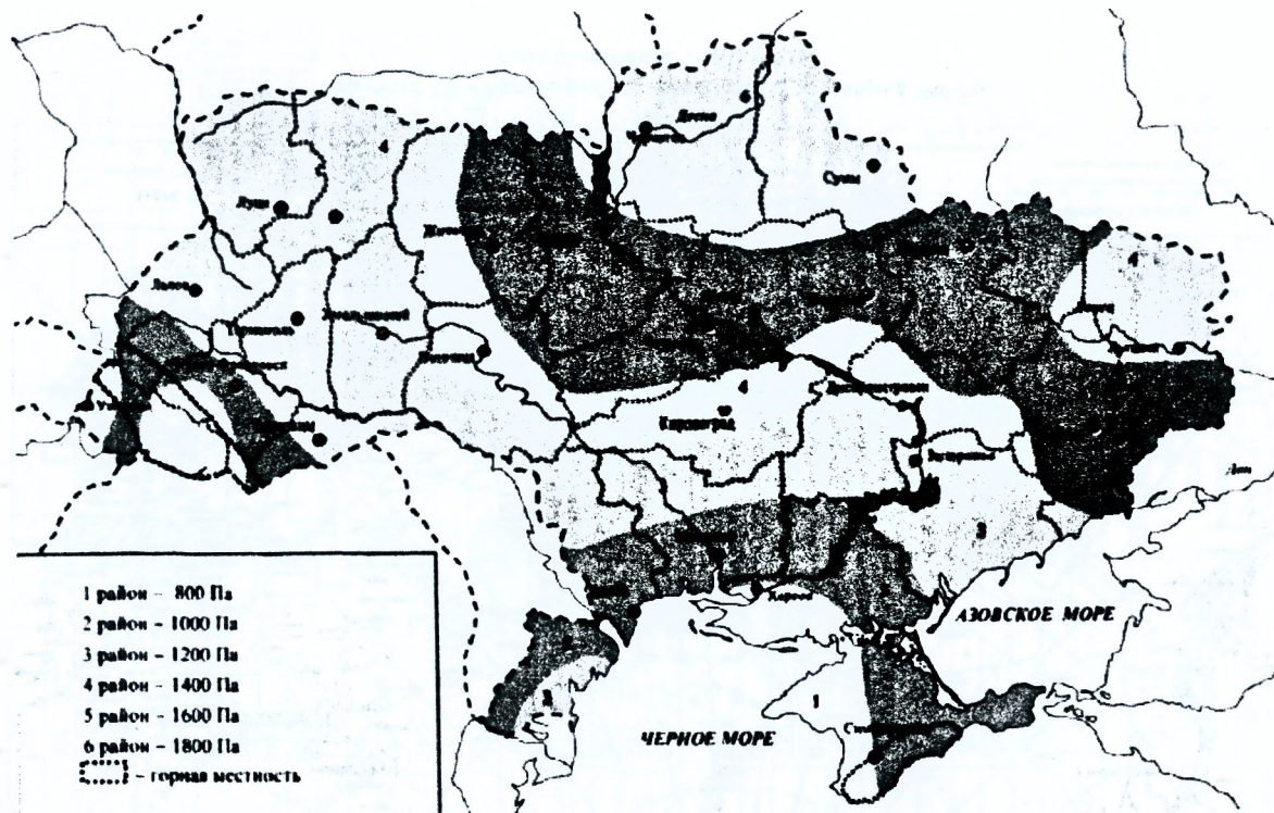
Рисунок 7.2 – Карта районирования территории Украины по характеристическим значениям веса снегового покрова [16]
