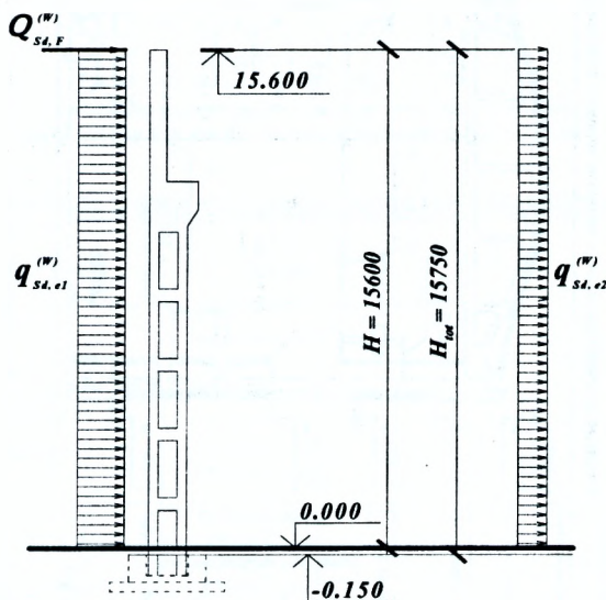
Рисунок 4.4 – К определению ветровой нагрузки на колонну
