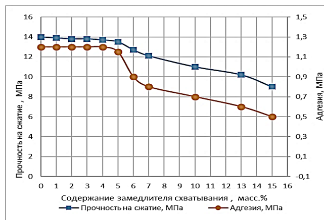
Рисунок 4 – Зависимость прочности на сжатие и адгезии композиции от количества замедлителя от количества замедлителя ( V/T = 0,37 )
