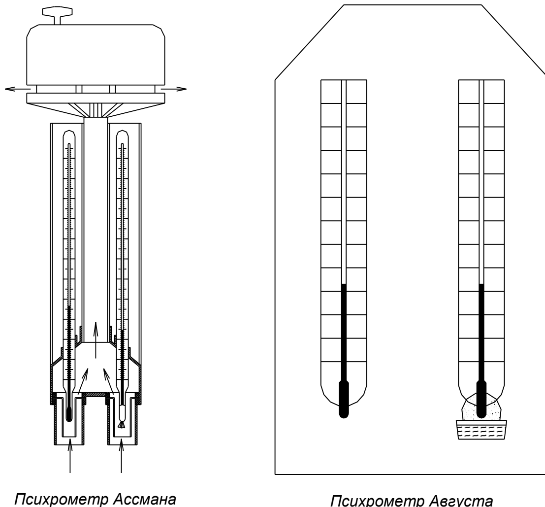
Рисунок 3.1.1 – Разновидности психрометров
