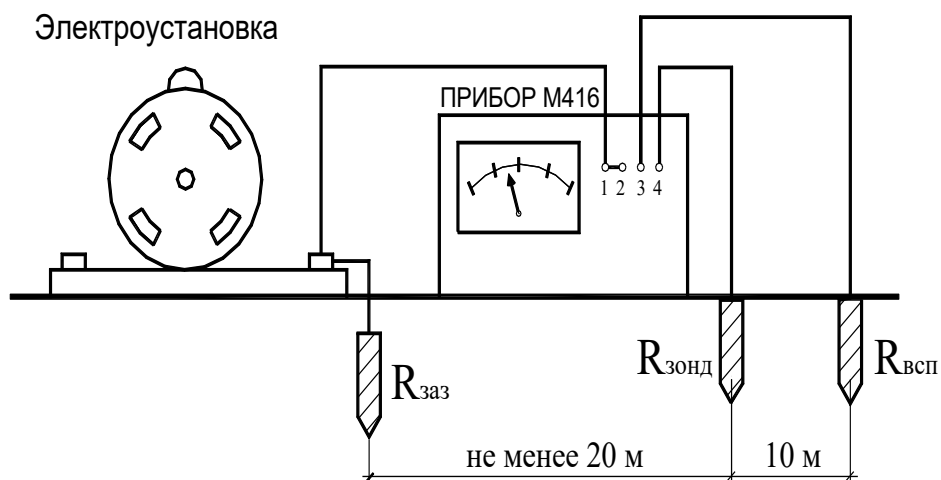
Рисунок 3.1 – Принципиальная схема соединений при измерении сопротивления заземляющего устройства
