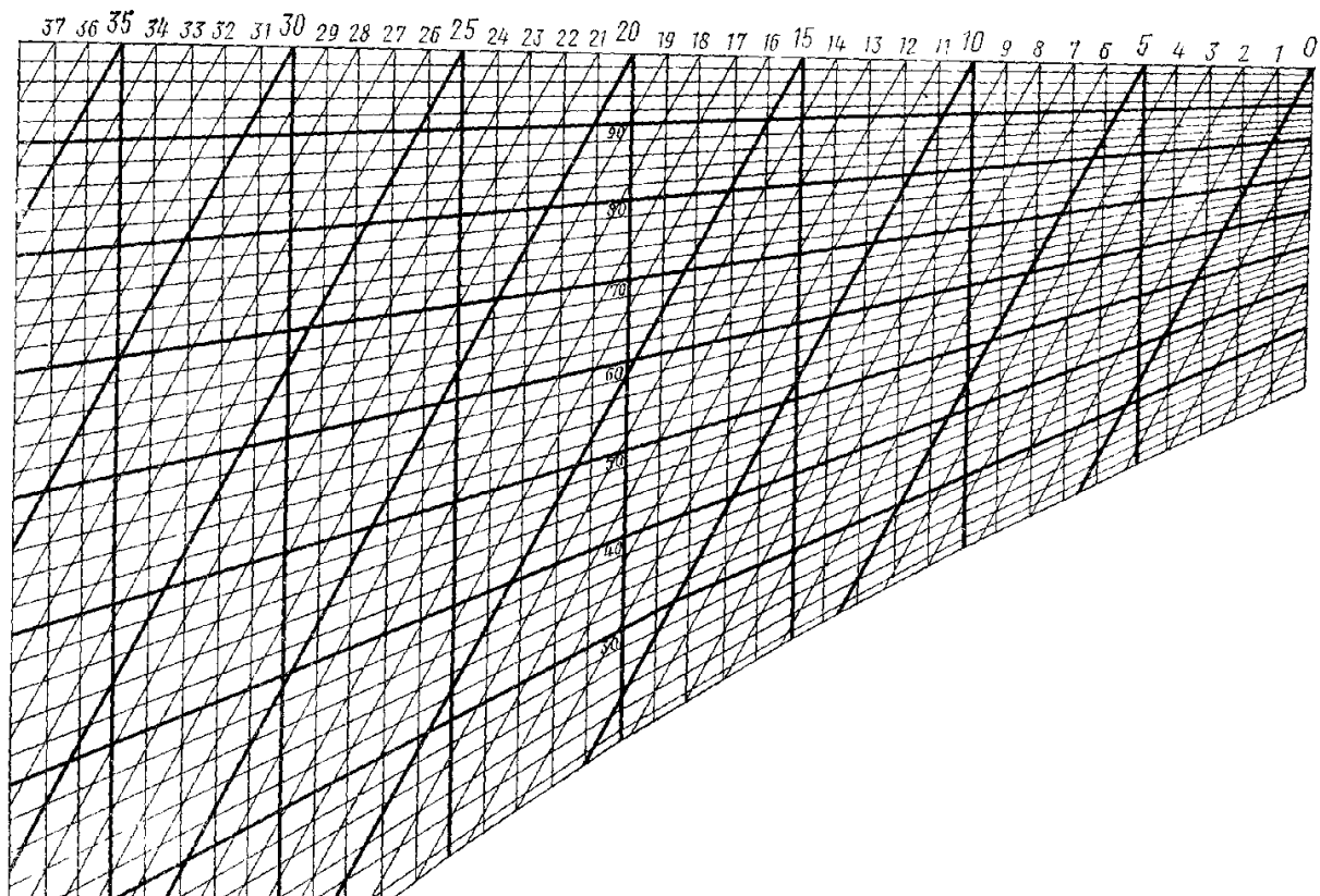
Рисунок 3.1.5 – Номограмма для определения относительной влажности
