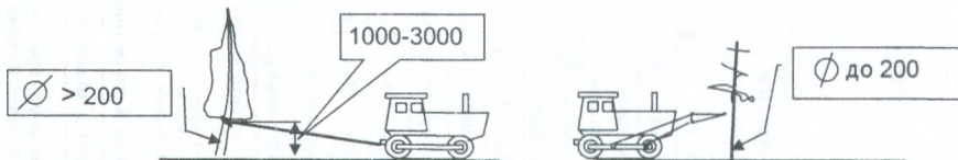
Рисунок 16.1 – Валка деревьев с использованием тракторов
