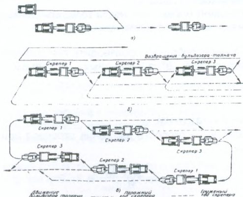
а – челночная; б – челочно-цепная; в – эллиптически – цепная Рисунок 21.16 – Схемы работы бульдозера-толкача
