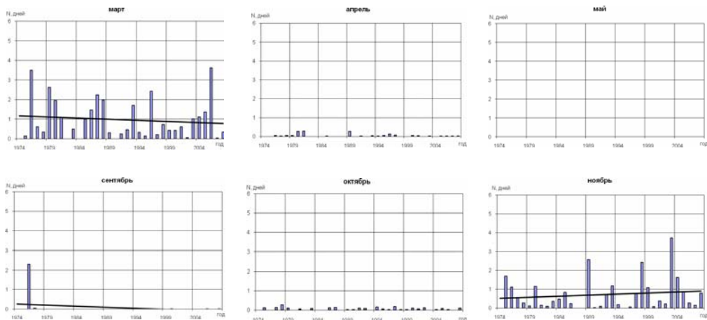
Рисунок 19 – Хронологический ход месячных значений количества дней с изморозевыми отложениями, приходящихся на одну метеостанцию на территории Беларуси
