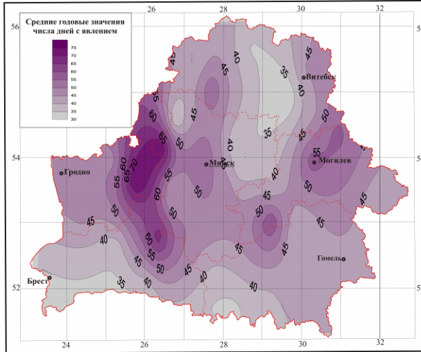
Рисунок 13 – Пространственное распределение среднего годового значения числа дней с туманами на территории Беларуси
