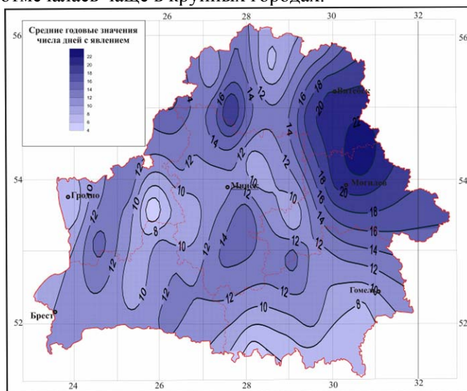
Рисунок 20 – Пространственное распределение среднего годового значения числа дней с изморозью на территории Беларуси
