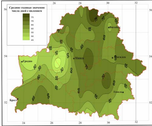
Рисунок 15 – Пространственное распределение среднего годового значения числа дней с инеем на территории Беларуси
