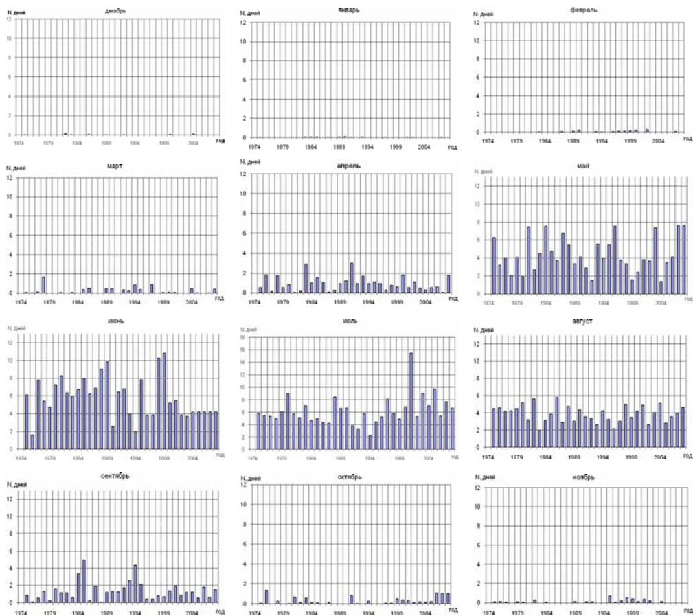
Рисунок 1– Хронологический ход месячных значений количества дней с грозами приходящихся на одну метеостанцию на территории Беларуси
