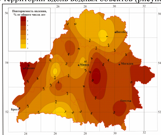
Рисунок 11 – Пространственное распределение засушливых явлений по территории Беларуси, % лет
