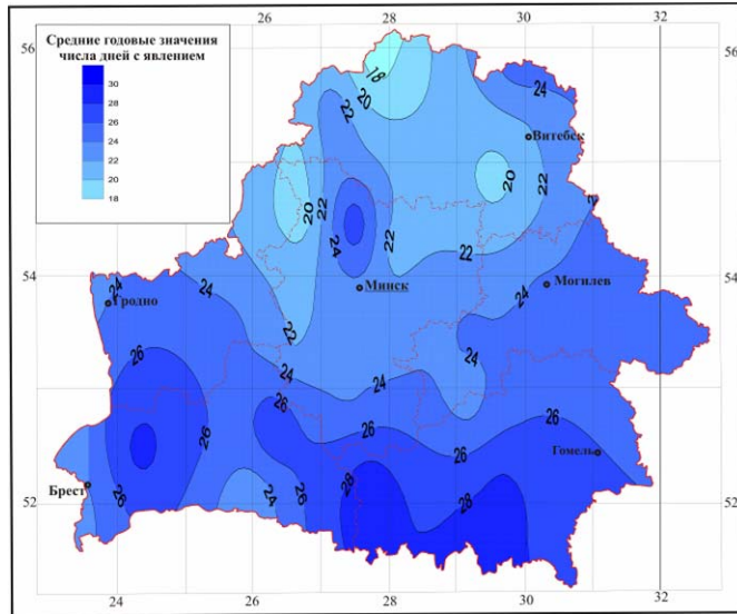
Рисунок 2 – Пространственное распределение среднего годового значения числа дней с грозами на территории Беларуси
