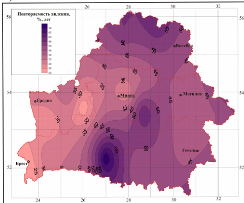
Рисунок 10 – Пространственное распределение повторяемости заморозков: весенних после 30.04 на высоте 2 м (а) и на поверхности почвы (б), и осенних до 30.09 на высоте 2 м (в) и на поверхности почвы (г) (% , лет)
