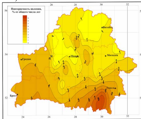
Рисунок 12 – Пространственное распределение сильной жары по территории Беларуси, % лет
