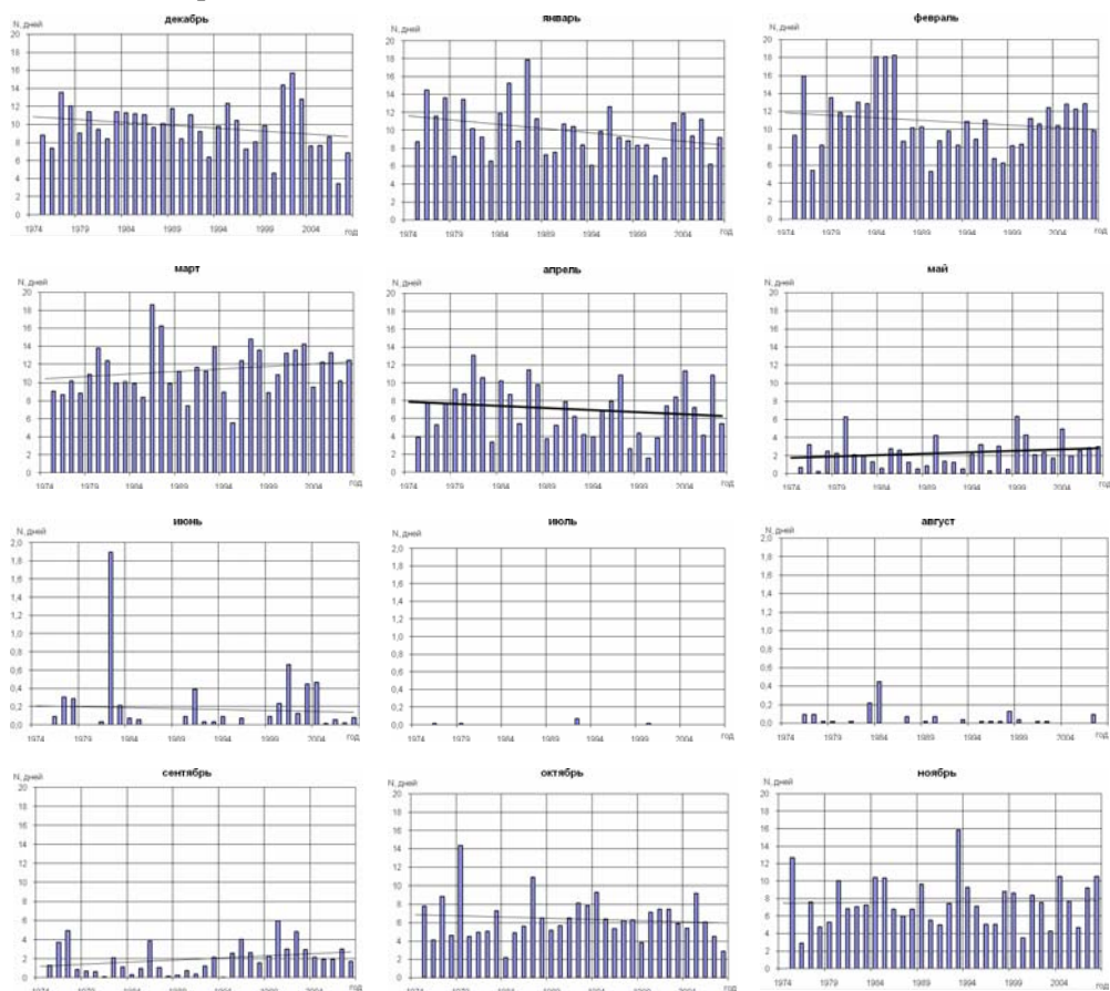
Рисунок 14 – Хронологический ход месячных значений количества дней с инеем приходящихся на одну метеостанцию на территории Беларуси
