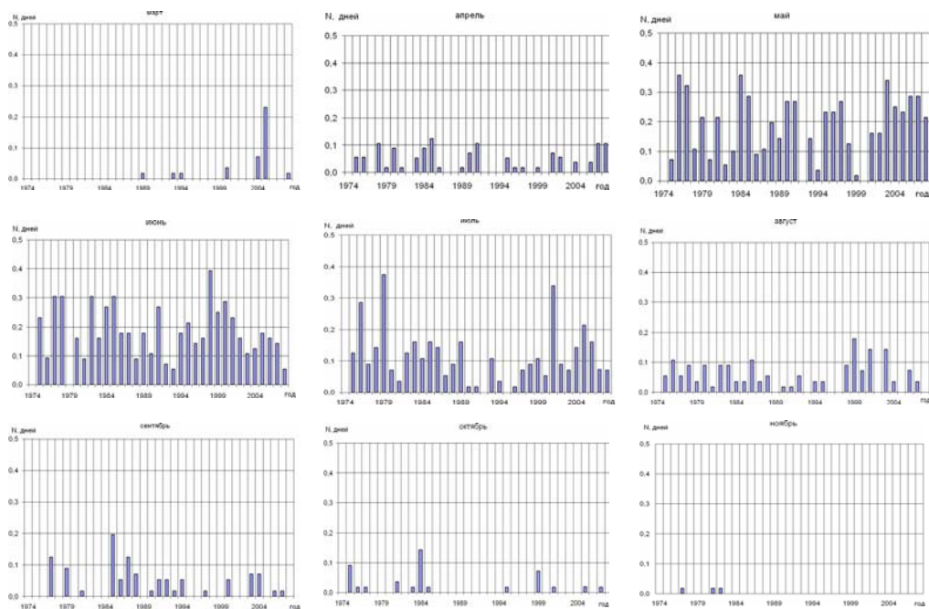
Рисунок 8 – Хронологический ход месячных значений количества дней с градом приходящихся на одну метеостанцию на территории Беларуси
