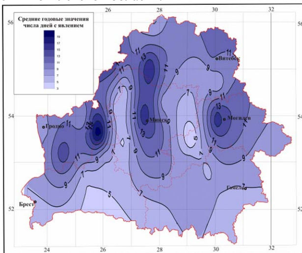
Рисунок 17 – Пространственное распределение среднего годового значения числа дней с гололедом на территории Беларуси
