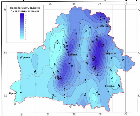
Рисунок 24 – Пространственное распределение сильного мороза на территории Беларуси, % лет
