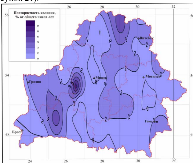
Рисунок 20 – Пространственное распределение сильного снегопада на территории Беларуси, % лет
