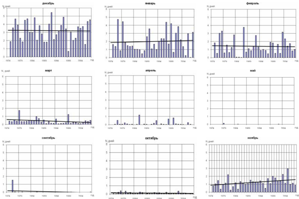
Рисунок 18 – Хронологический ход месячных значений количества дней с гололедом приходящихся на одну метеостанцию на территории Беларуси
