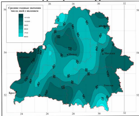
Рисунок 6 – Пространственное распределение среднего годового значения числа дней с дождями ливневыми на территории Беларуси
