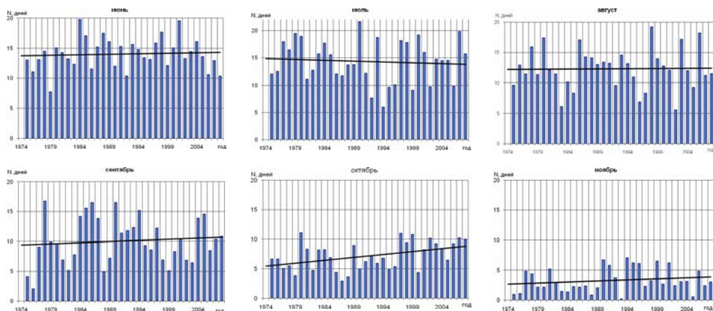
Рисунок 5 – Хронологический ход месячных значений количества дней с ливневыми дождями приходящихся на одну метеостанцию на территории Беларуси
