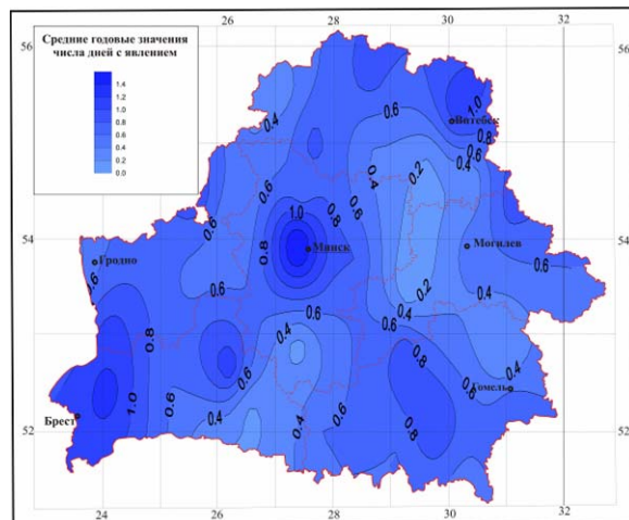
Рисунок 9 – Пространственное распределение среднего годового значения числа дней с градом на территории Беларуси
