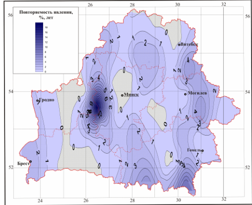
Рисунок 16 – Пространственное распределение повторяемости гололедно-изморозевых отложений по территории Беларуси, % лет
