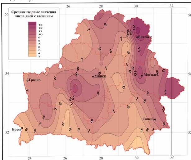
Рисунок 22 – Пространственное распределение среднего годового значения числа дней с метелями на территории Беларуси
