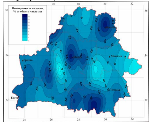
Рисунок 7 – Пространственное распределение сильных дождей по территории Беларуси, % лет
