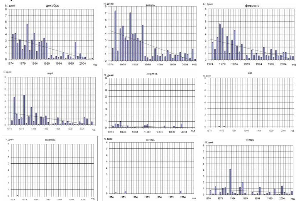
Рисунок 23 – Хронологический ход среднего количества дней с метелями, приходящихся на одну метеостанцию на территории Беларуси
