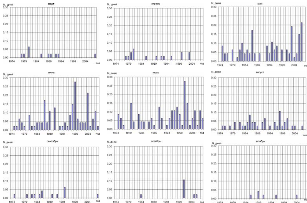
Рисунок 3 – Хронологический ход месячных значений количества дней со шквалами приходящихся одну метеостанцию на территории Беларуси
