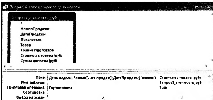
Рис. 45. Запрос14 в режиме Конструктора
