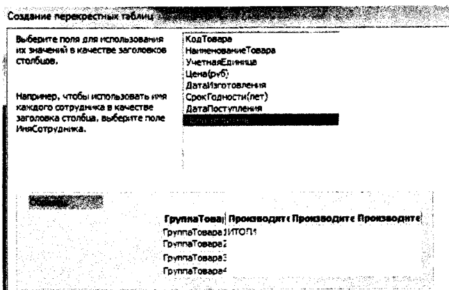
Рис. 52. Третий шаг Мастера создания перекрестного запроса
