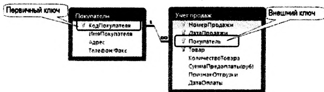
Рис. 25. Связь между таблицами, обеспеченная целостностью данных
