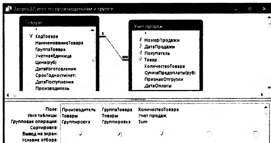
Рис. 43. Запрос12 в режиме Конструктора
