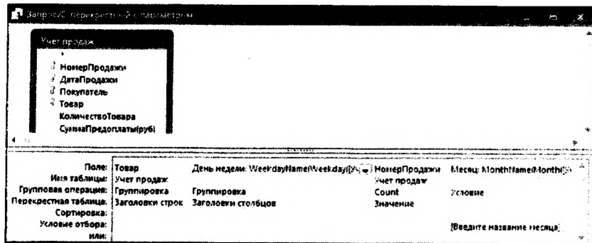
Рис. 58. Запрос20 в режиме Конструктора
