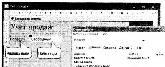
Рис. 64. Создание вычисляемого поля в форме
