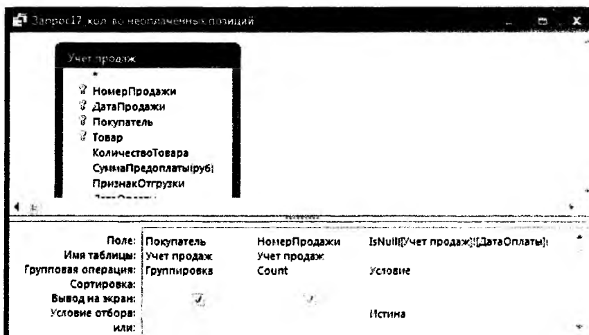
Рис. 48. Запрос17 в режиме Конструктора
