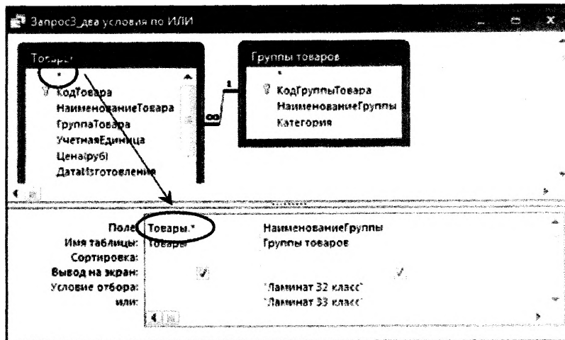
Рис. 32. Запрос3 в режиме Конструктора
