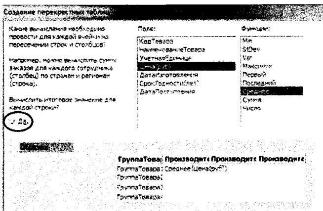
Рис. 53. Четвертый шаг Мастера создания перекрестного запроса
