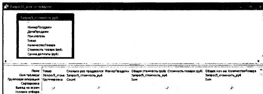
Рис. 42. Запрос11 в режиме Конструктора
