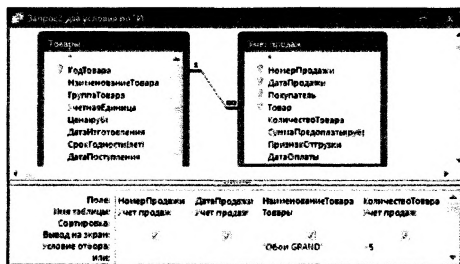
Рис. 31. Запрос2 в режиме Конструктора
