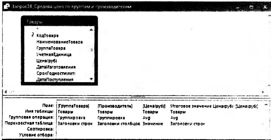
Рис. 55. Запрос18 в режиме Конструктора
