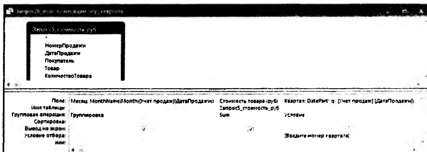
Рис. 47. Запрос16 в режиме Конструктора
