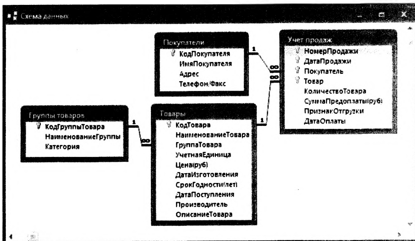
Рис. 16. Схема данных в БД Магазин "Строитель"
