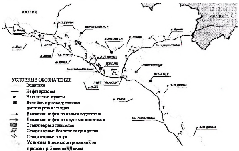
Рисунок – Схема движения нефти по водотокам
