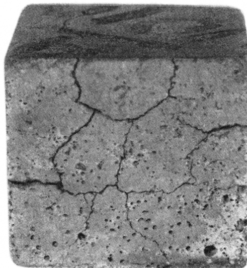
Рис.4. Образец цементного раствора, подвергшийся сульфатной коррозии.
