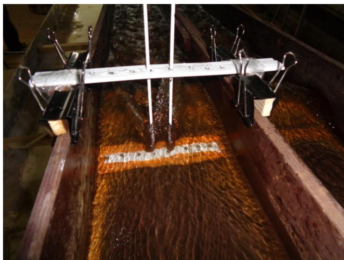
Рисунок 6 – Модель в виде бычка криволинейной вогнутой формы
