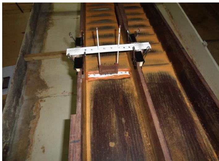
Рисунок 4 – Модель сетчатой селезадерживающей конструкции в сборе
