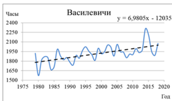
Рисунок 4 – Временная изменчивость ПСС на территории Беларуси
