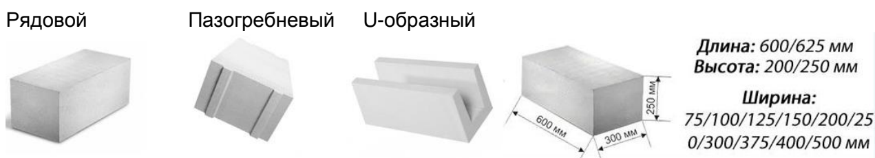
Рисунок 1 – Основные виды и размеры газосиликатных блоков
