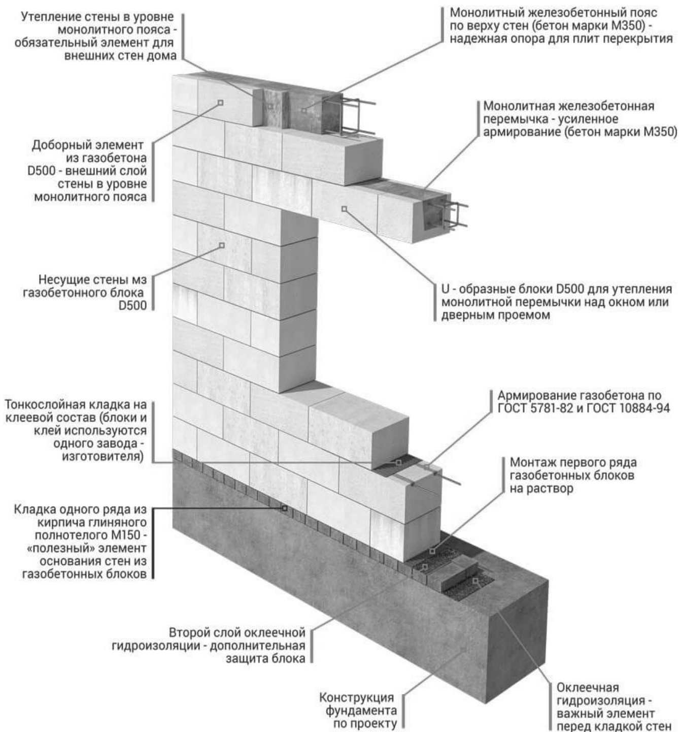
Рисунок 6 – Фрагмент стены из газобетонных блоков
