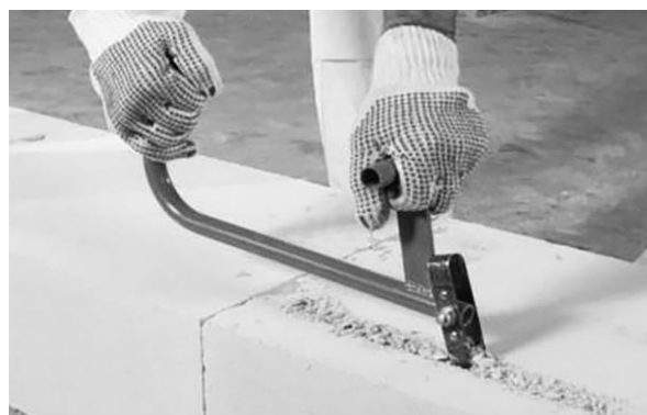
Рисунок 5 – Нарезка штроб под арматуру и уложенная арматура
