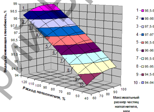
Рис. 8. Изменение водоудерживающей способности в зависимости от расхода наполнителя и максимального размера частиц наполнителя
