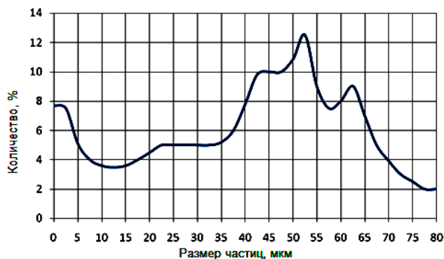
Рис. 10. Гранулометрическая кривая распределения частиц наполнителя
