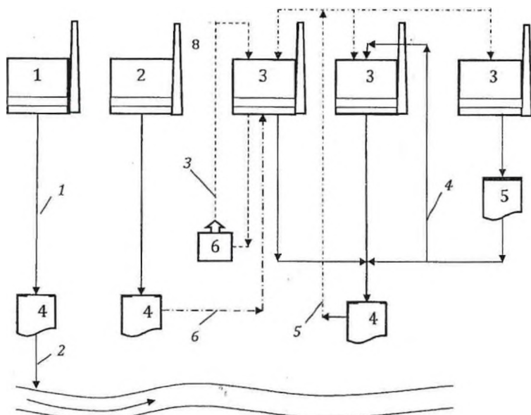
Рис. 3.1 Схемы систем водоотведения промышленных предприятий
