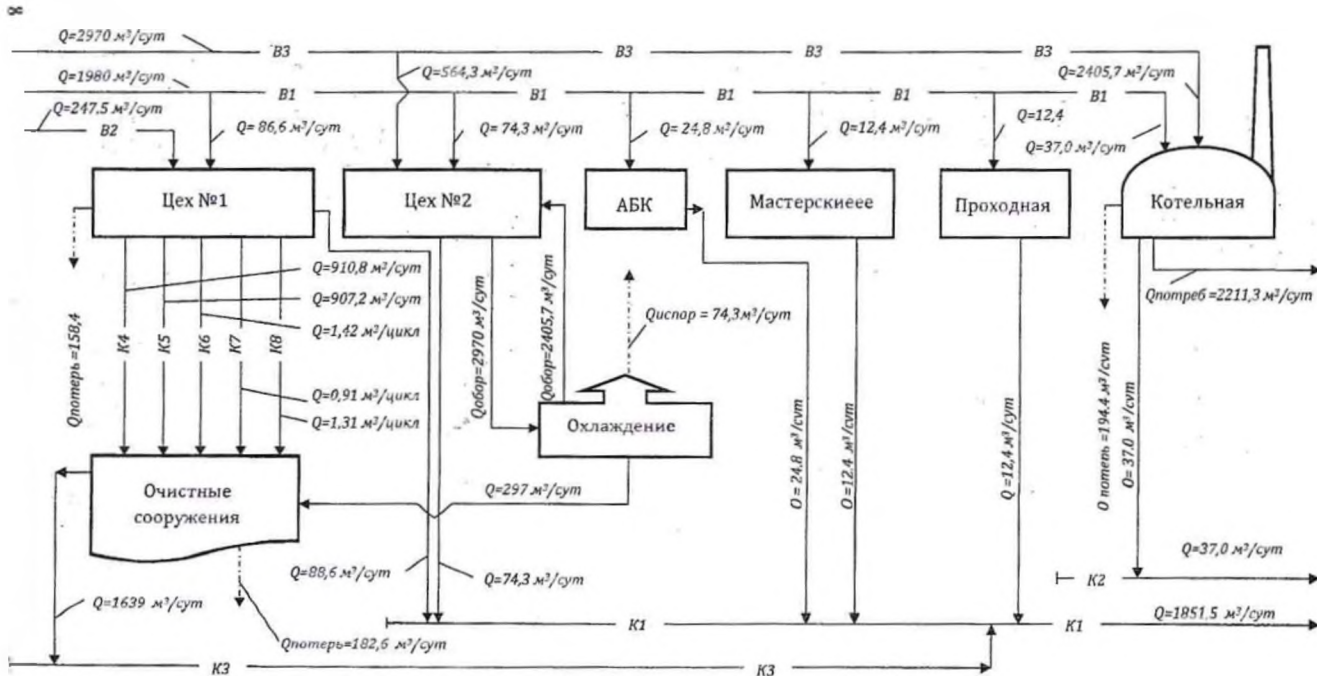
Рис. 2.1. Балансовая схема водоразъема и водоотведения промышленного предприятия
