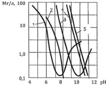
Рис. 6.1.3.1. Кривые осаждения металлов традиционно применяемыми реагентами в фильтровальной пробе без учёта эффекта соосаждения 1 - Cr 3+ ; 2 - Cu 2+ ; 3 - Zn 2+ ; 4 - Ni 2+ ; 5 - Cd 2+
