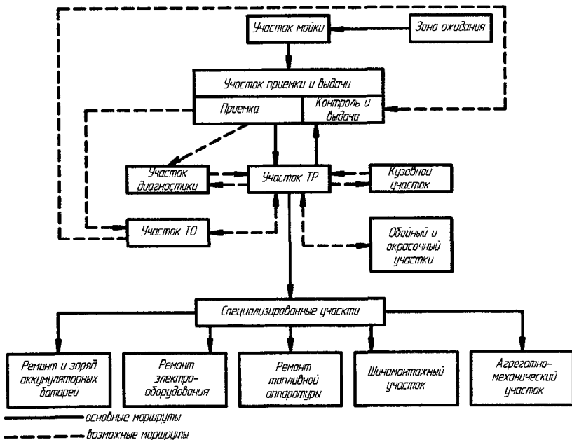
Рисунок 9 – Схема технологического процесса ТР на ПА
