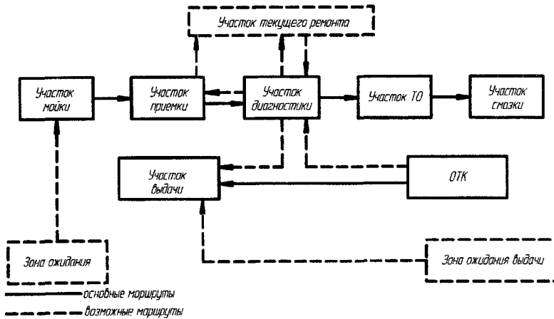
Рисунок 8 – Схема производственного процесса полного объема ТО на ПА
