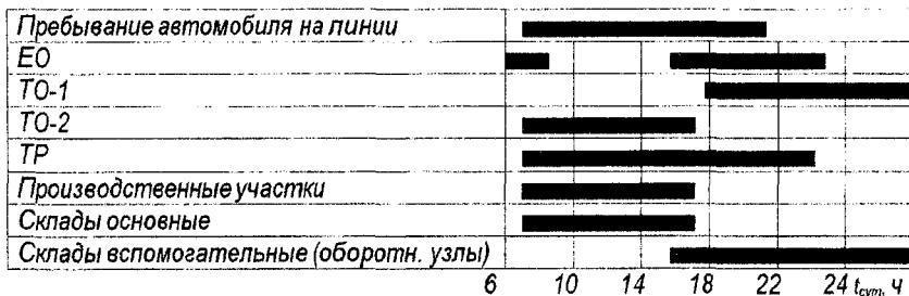
Рисунок 4 – Линейный график производственного процесса
