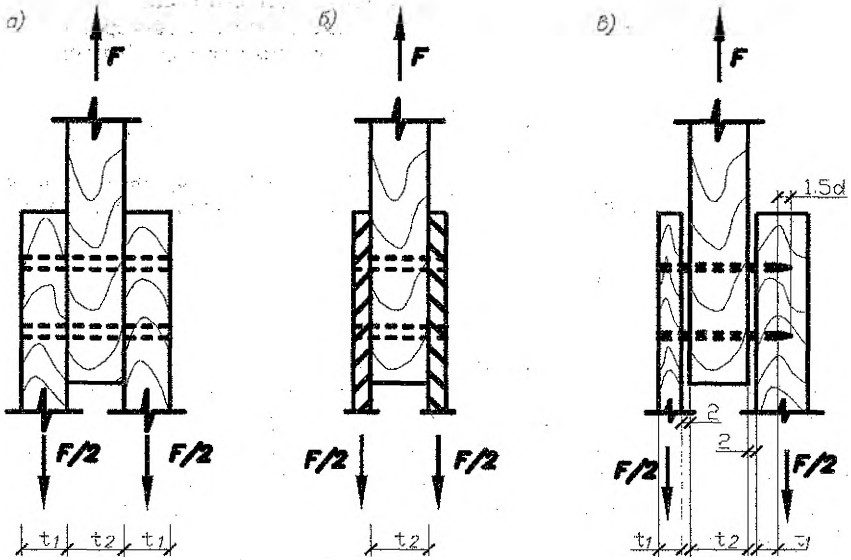
а) — нагельные древесины с древесиной б) — нагельные металлических пластин с древесиной в) — гвоздевые древесины с древесиной
