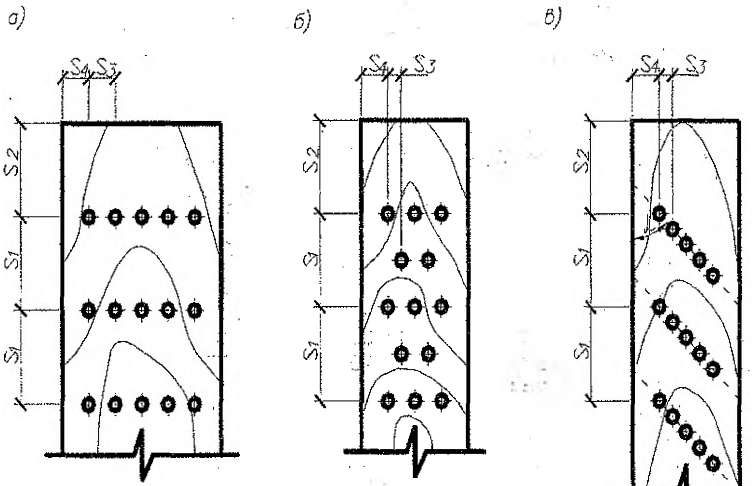
а) — нормальная б) — в шахматном порядке в) — косыми рядами (только гвоздей при \alpha \leq 45^\circ )
