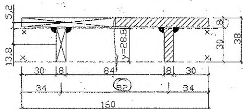
Рисунок 2.8. Упорная плита башмака с рёбрами жёсткости
