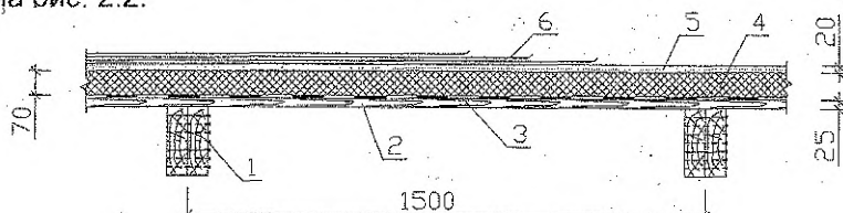
Рисунок 2.2. Конструктивная схема крыши
