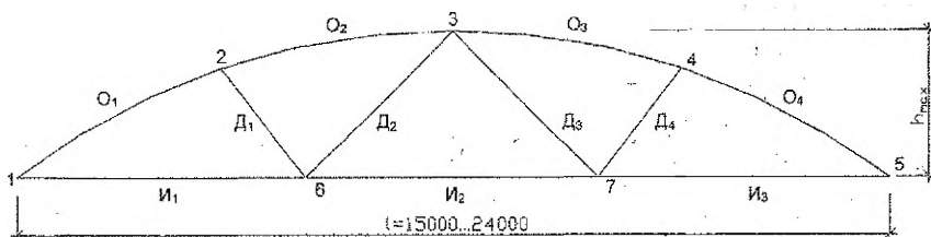
Рисунок А.2. Схема сегментной фермы с числом панелей верхнего пояса равным 4
