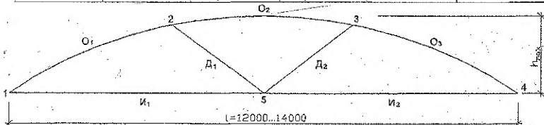
Рисунок А.1. Схема сегментной фермы с числом панелей верхнего пояса равным 3
