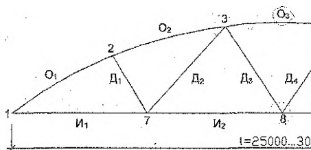
Рисунок А.3. Схема сегментной фермы с числом панелей верхнего пояса равным 5
