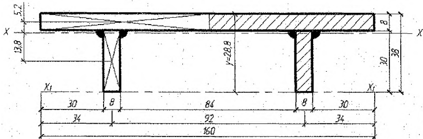
Рисунок 3.5 – Упорная плита башмака с рёбрами жёсткости
