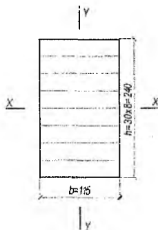
Рисунок 3.2 – Сечение верхнего пояса фермы
