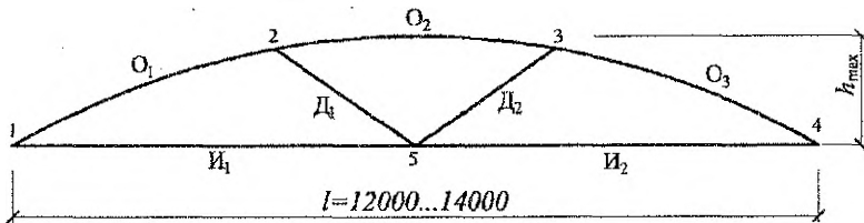
Рисунок У1 – Схема фермы
