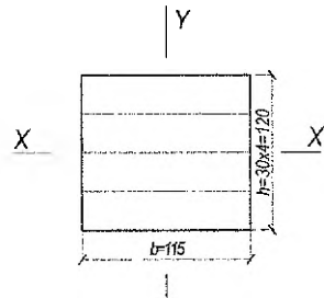
Рисунок 3.3 – Сечение раскосов
