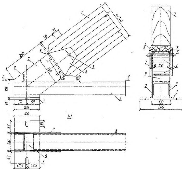
1 – опорная плита; 2 – вертикальные фанонки сварного башмака; 3 – упорная плита; 4 – ребра жесткости упорной плиты; 5 – болт \varnothing 14 мм, l=160 мм; 6 – накладки для соединения башмака с верхним поясом; 7 – верхний пояс фермы; 8 – нижний пояс фермы ( 2\angle 75 \times 50 \times 5 ); 9 – соединительная прокладка \angle 75 \times 50 \times 5 , l=100 мм
