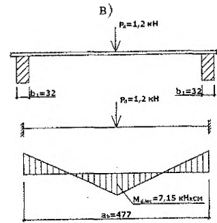
а – план плиты; б – поперечный разрез плиты; в – расчётная схема верхней обшивки на монтажную нагрузку; 1 – вкладыш, 2 – стык фанерной обшивки «на ус»; 3 – верхняя фанерная обшивка; 4 – нижняя фанерная обшивка; 5 – продольное ребро; 6 – стыковочный брусок; 7 – пароизоляция; 8 – утеплитель
