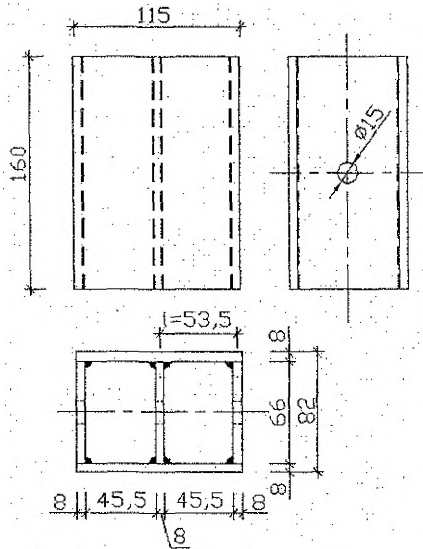
Рисунок 3.7 – Сварной вкладыш конькового узла
