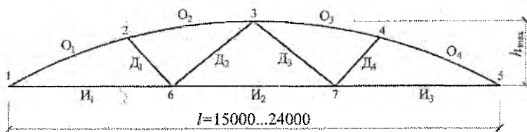
Рисунок У2 – Схема фермы
