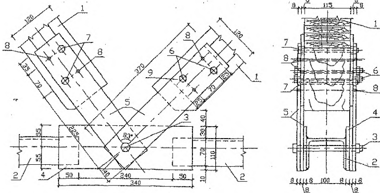
1 – раскос, 2 – нижний пояс фермы (2 \angle 75 \times 50 \times 5); 3 – узловой болт \varnothing 14 мм, l=170мм; 4 – передаточная пластина 340 \times 110 \times 8 мм; 5 – пластинки-наконечники 370 \times 80 \times 8 мм; 6 – болт \varnothing 10 мм, l=170 мм; 7 – болт \varnothing 10 мм, l=160 мм, 8 – гвоздь \varnothing 5 мм; 9 – подкладка 120 \times 80 \times 8 мм Рисунок 3.8 – Нижний промежуточный узел фермы
