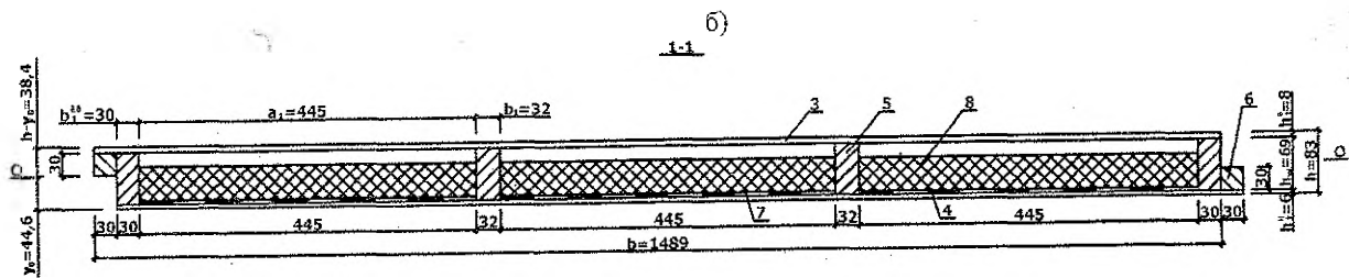
а – план плиты; б – поперечный разрез плиты; в – расчётная схема верхней обшивки на монтажную нагрузку; 1 – вкладыш, 2 – стык фанерной обшивки «на ус»; 3 – верхняя фанерная обшивка; 4 – нижняя фанерная обшивка; 5 – продольное ребро; 6 – стыковочный брусок; 7 – пароизоляция; 8 – утеплитель
