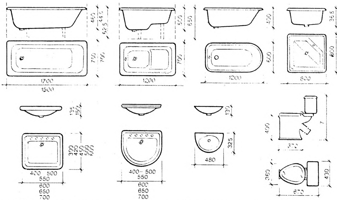
Рис.5 Габаритные размеры предметов оборудования санитарных узлов
