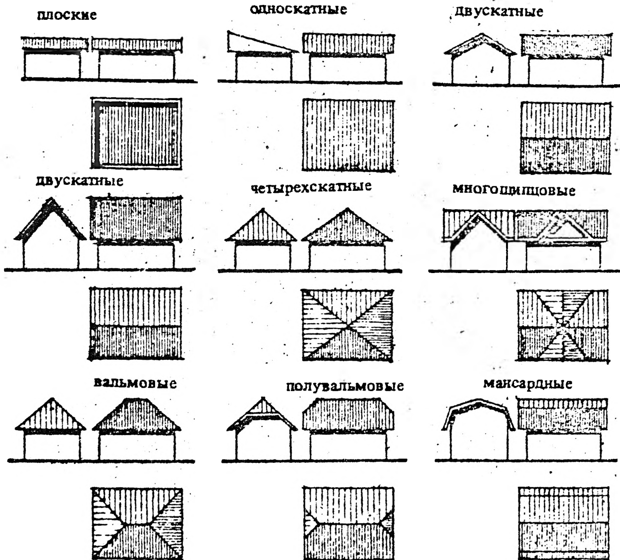
Рис.8 Типы крыш малоэтажного жилого дома
