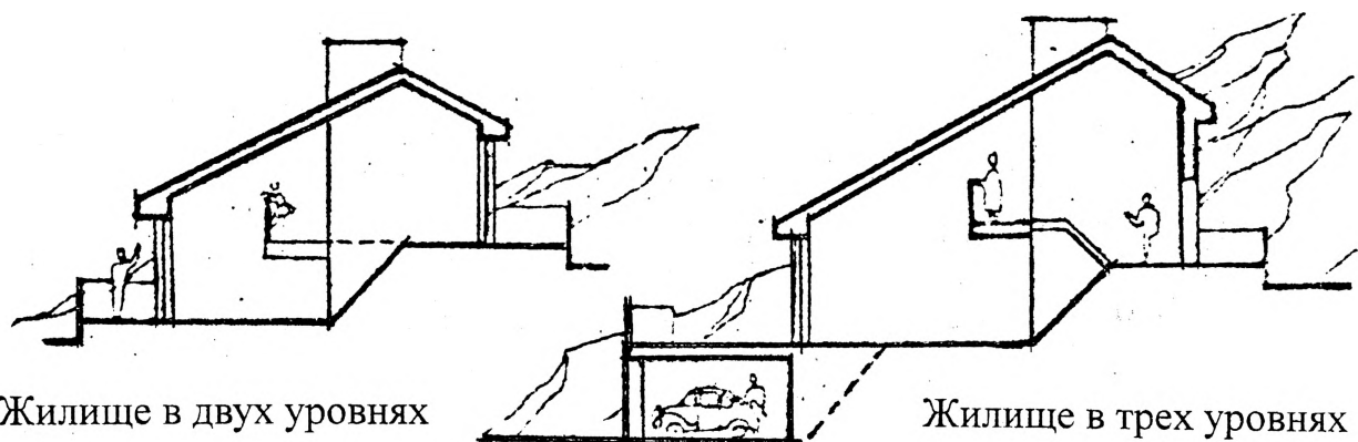
Рис.7 Примеры организации внутреннего пространства малоэтажного жилого дома.
