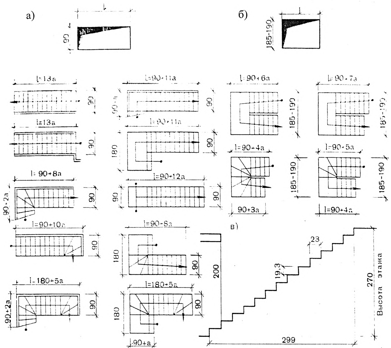
Рис.6 Типы внутриквартирных лестниц:
