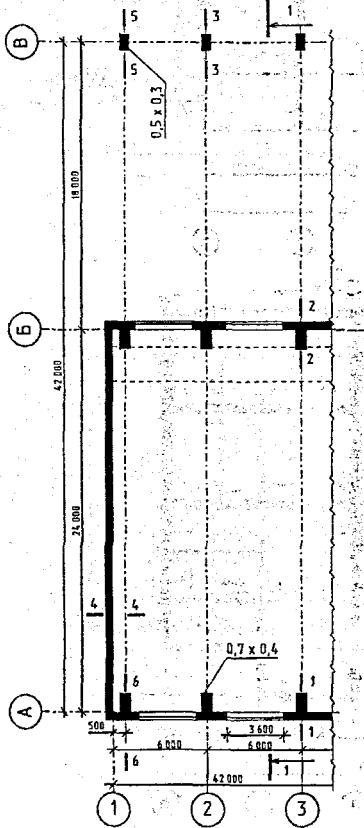
План цеха
