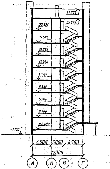
Разрез I-I
