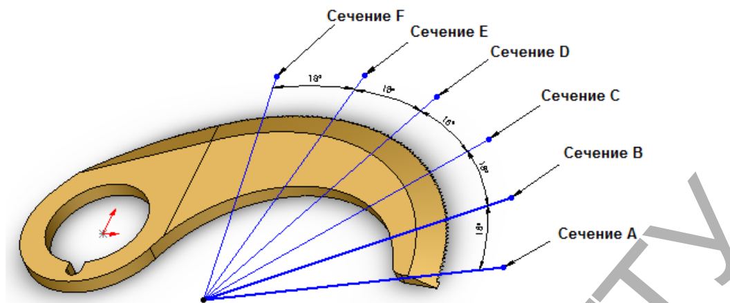
Рисунок 1 – Расположение сечений на рабочей зоне ножа
