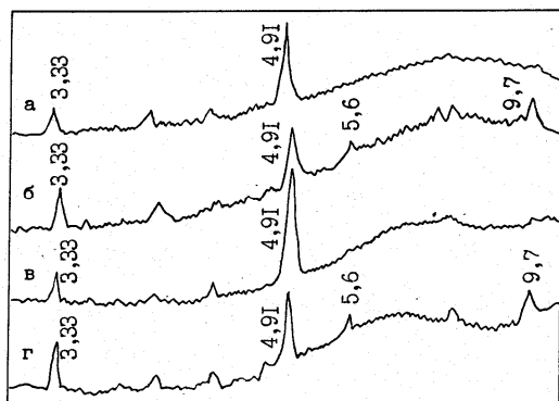
Рисунок 3 - Рентгенограммы гидратированных цементов: контрольный цемент через 3 суток (а), через 28 суток (в); цемент с САД через 3 суток (б), через 28 суток (г).
