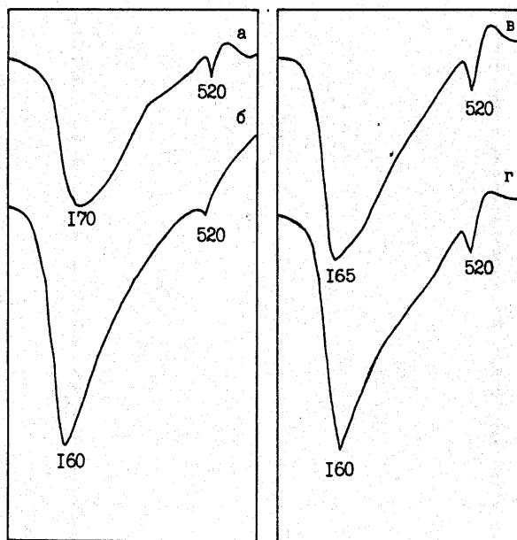
Рисунок 4 - Фрагменты термограмм образцов цемента: после 3 суток гидратации (а) - контрольный цемент, (б) - цемент с САД; после 28 суток гидратации: (в) - контрольный цемент, (г) - цемент с САД.
