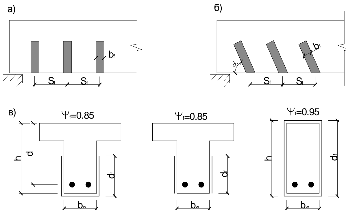
Рисунок 10.3 – Расположение ФАП хомутов при усилении наклонного сечения
