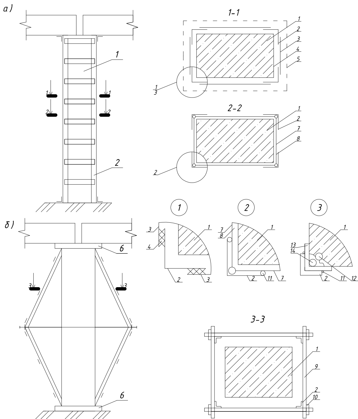
а) с напряженными планками; б) с напряженными распорками (1-1 и 2-2 – варианты конструктивного решения)
