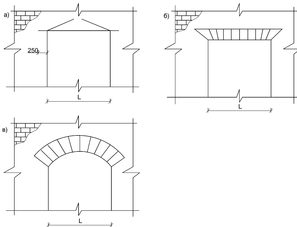
а – рядовая; б – клинчатая; в - арочная Рисунок 13.1 – Тип перемычек из кирпича
