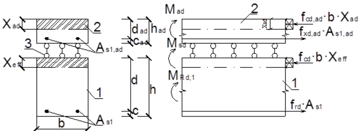
Рисунок 6.1 – Расчетная схема усиления наращиванием без сцепления существующего и нового бетона
