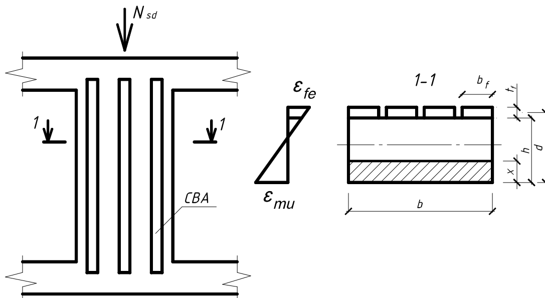
Рисунок 15.2 – К расчету усиления внецентренно сжатого простенка
