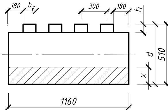
Рисунок 15.3 – К расчету усиления элементами СВА
