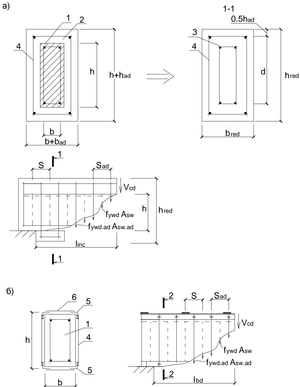
а) при усилении обоймой; б) при усилении внешней арматурой Рисунок 6.6 – Схема действующих усилий при усилении наклонного сечения
