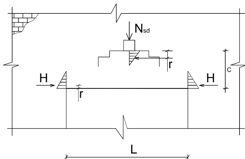
Рисунок 13.2 – К расчёту перемычек
