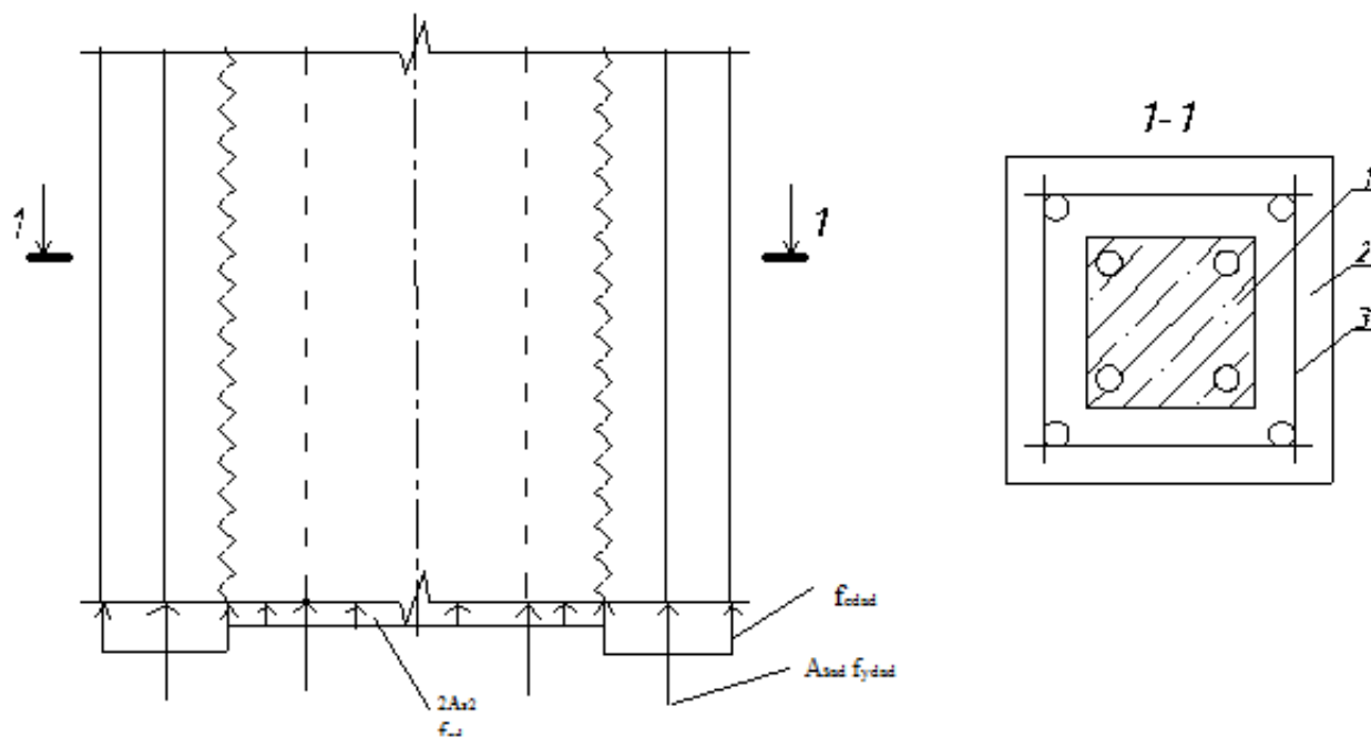
1 – усиливаемый элемент; 2 – бетон обоймы; 3 – арматура обоймы Рисунок 7.2 – К расчету усиления обоймой из железобетона
