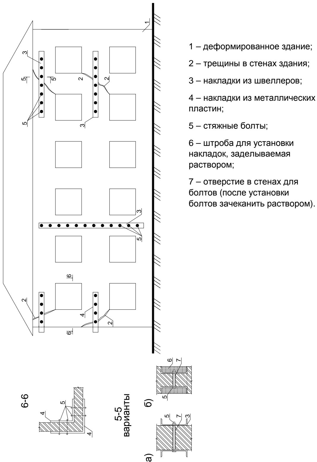
Рисунок 14.3 – Установка напряженных поясов с наружной стороны здания
