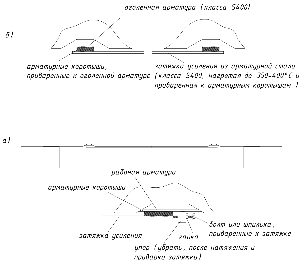
а) с натяжением гайками; б) с нагревом; в) с нагревом на упоры Рисунок 9.1 – Усиление изгибаемых элементов затяжкой
