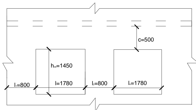
Рисунок 13.3 – К расчёту перемычек по примеру
