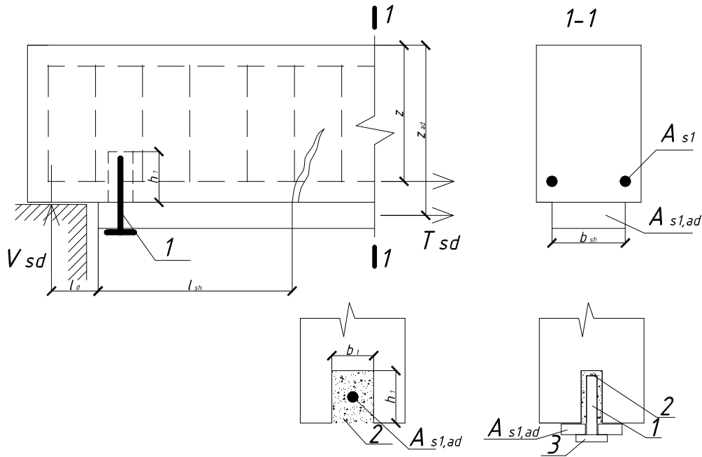
1 - анкер; 2 - полимерраствор; 3 - сварка Рисунок 5.4 – К расчету прочности контактного шва
