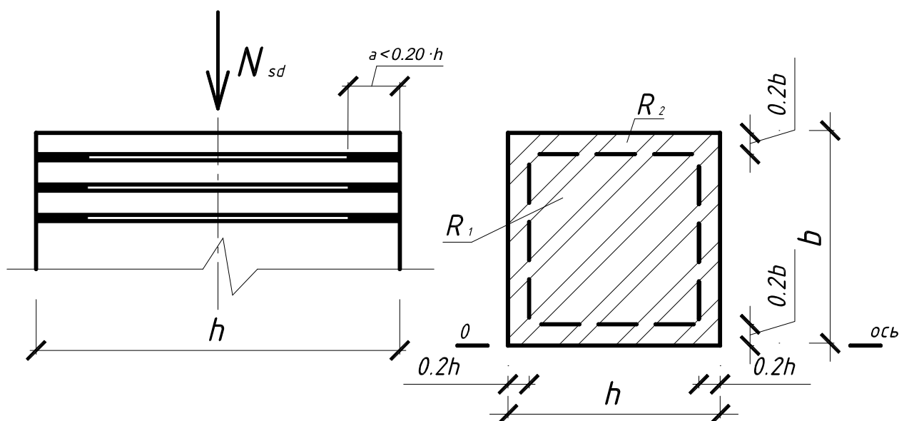
Рисунок 15.4 – К расчету усиления полимерцементным раствором
