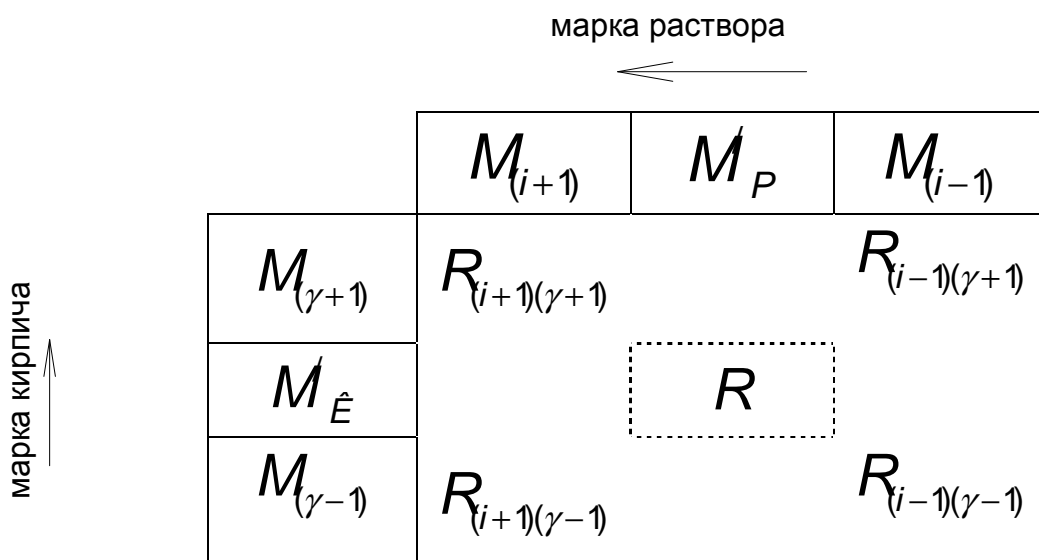
Рисунок 11.1 – Схема определения расчетного сопротивления кирпичной кладки по результатам испытания образцов.
