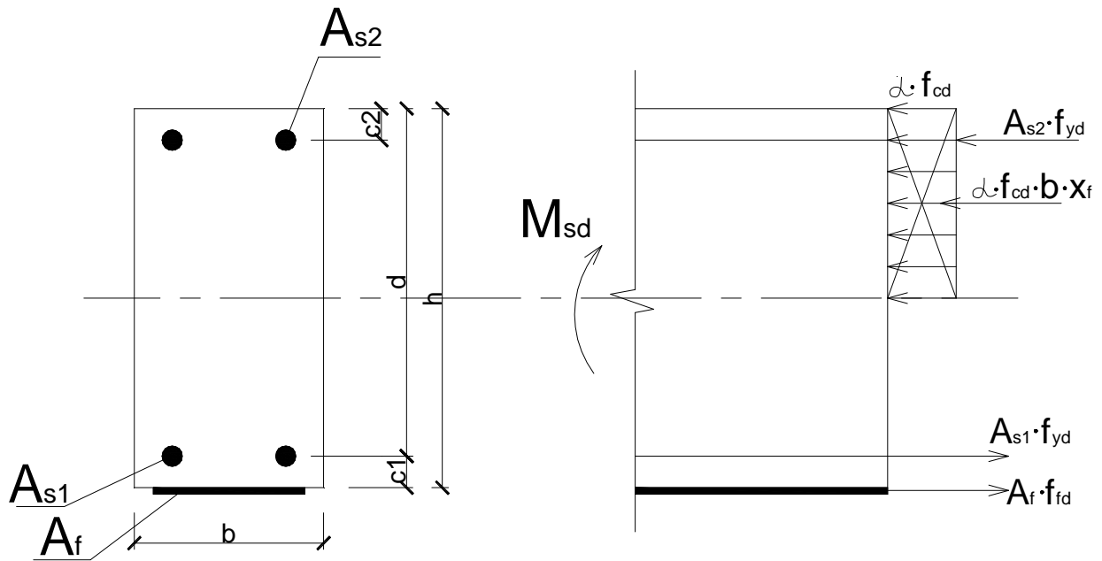
Рисунок 10.2 – Схема усилий и эпюра напряжений в сжатой зоне нормального сечения усиленного изгибаемого элемента.
