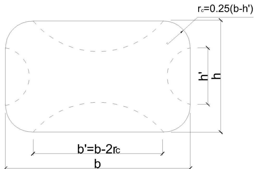
Рисунок 10.3 – Положение активных зон при усилении прямоугольных сечений колонн.
