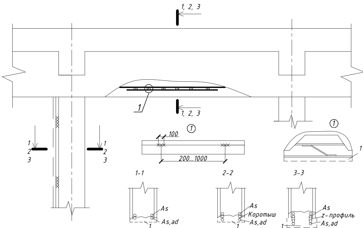
Рисунок 5.1 – Усиление растянутой зоны конструкций приваркой дополнительной арматуры: 1 - ремонтный состав
