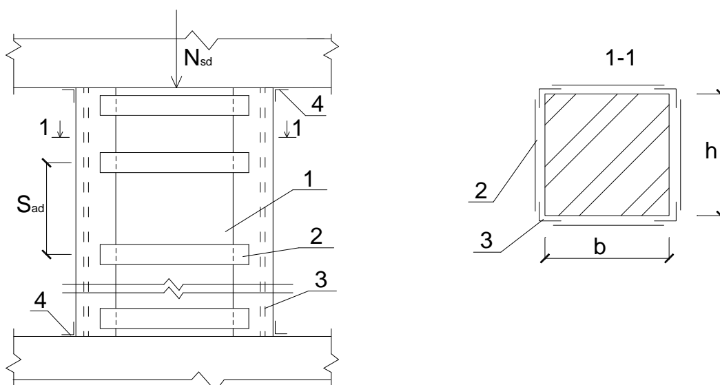
Рисунок 12.2 – Усиление кирпичного столба обоймой из металла
