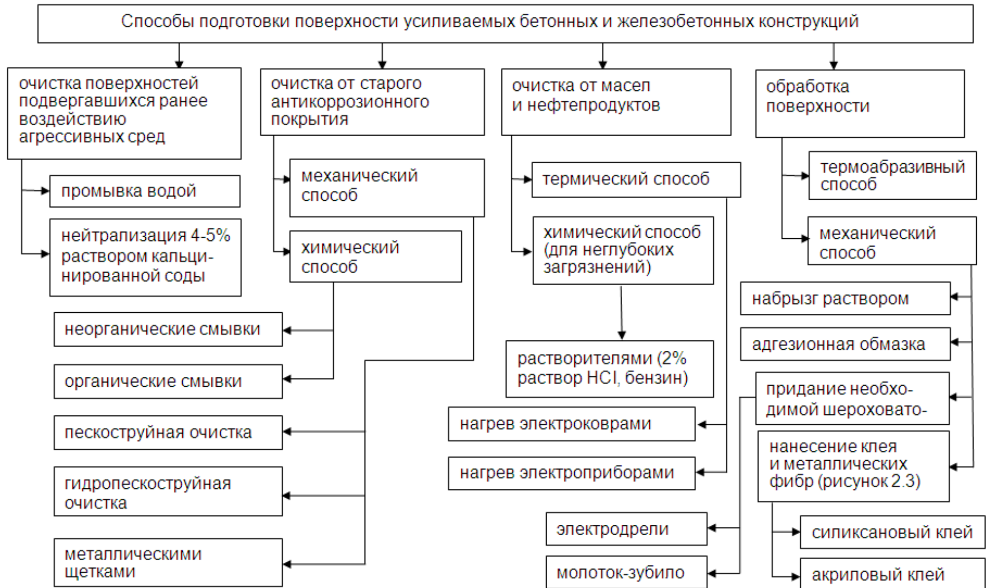
Рисунок 2.1 – Классификация способов подготовки поверхности бетона к ремонту
