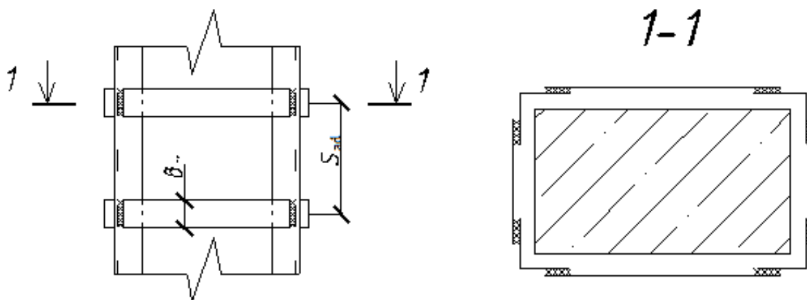
Рисунок 7.5 – К расчету усиления обоймой из металла
