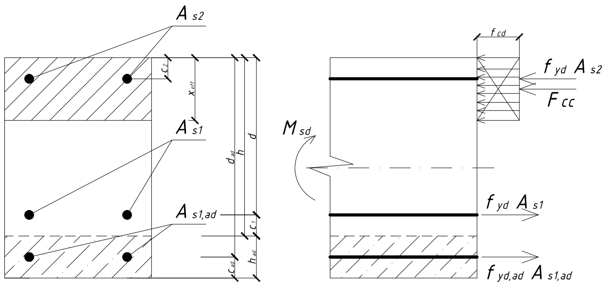
Рисунок 5.3 – Расчетная схема нормального сечения изгибаемого элемента с усиленной растянутой зоной
