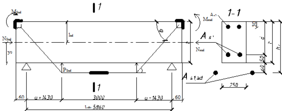
Рисунок 9.5 – К расчету шпренгельной затяжки
