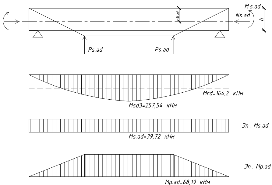
Рисунок 9.6 – К расчету шпренгельной затяжки
