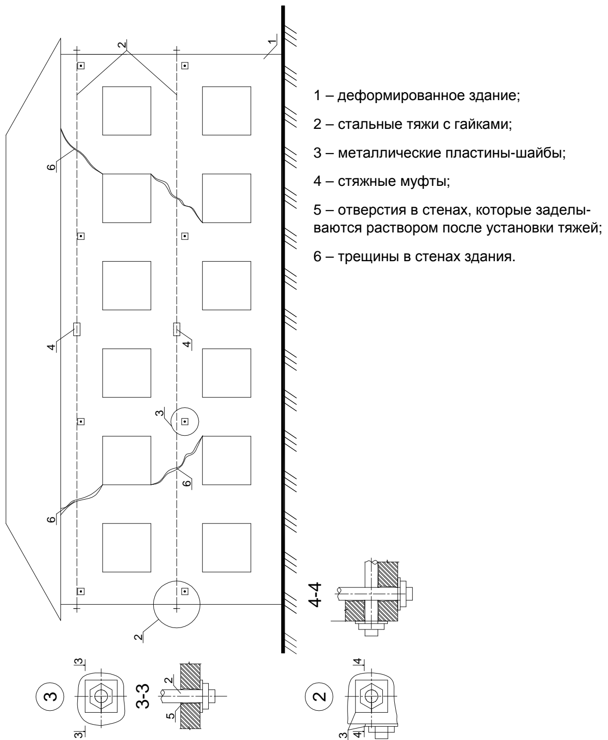
Рисунок 14.2 – Установка напряженных поясов внутри здания.
