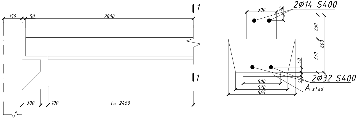
Рисунок 5.6 – К расчету усиления растянутой зоны наклейкой дополнительной арматуры
