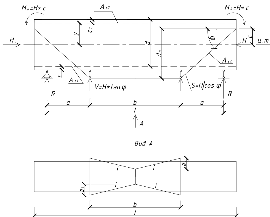
Рисунок 9.4 – К расчету шпренгельной затяжки
