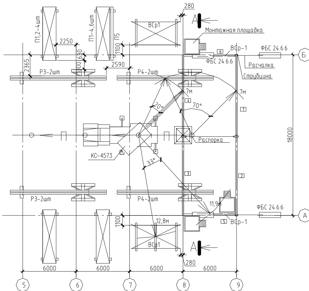
Рисунок 4.4.15 – Схема монтажа полурам и связей способом поворота со смещением стоянки относительно поперечной оси вперед по ходу крана
