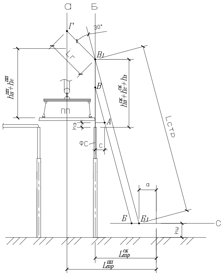
Рисунок 4.4.7 – Схема графического определения L_{стр} , L_г и L_{мп} при монтаже стропильной конструкции и плиты покрытия, располагаемой напротив стоянки крана, гуськом
