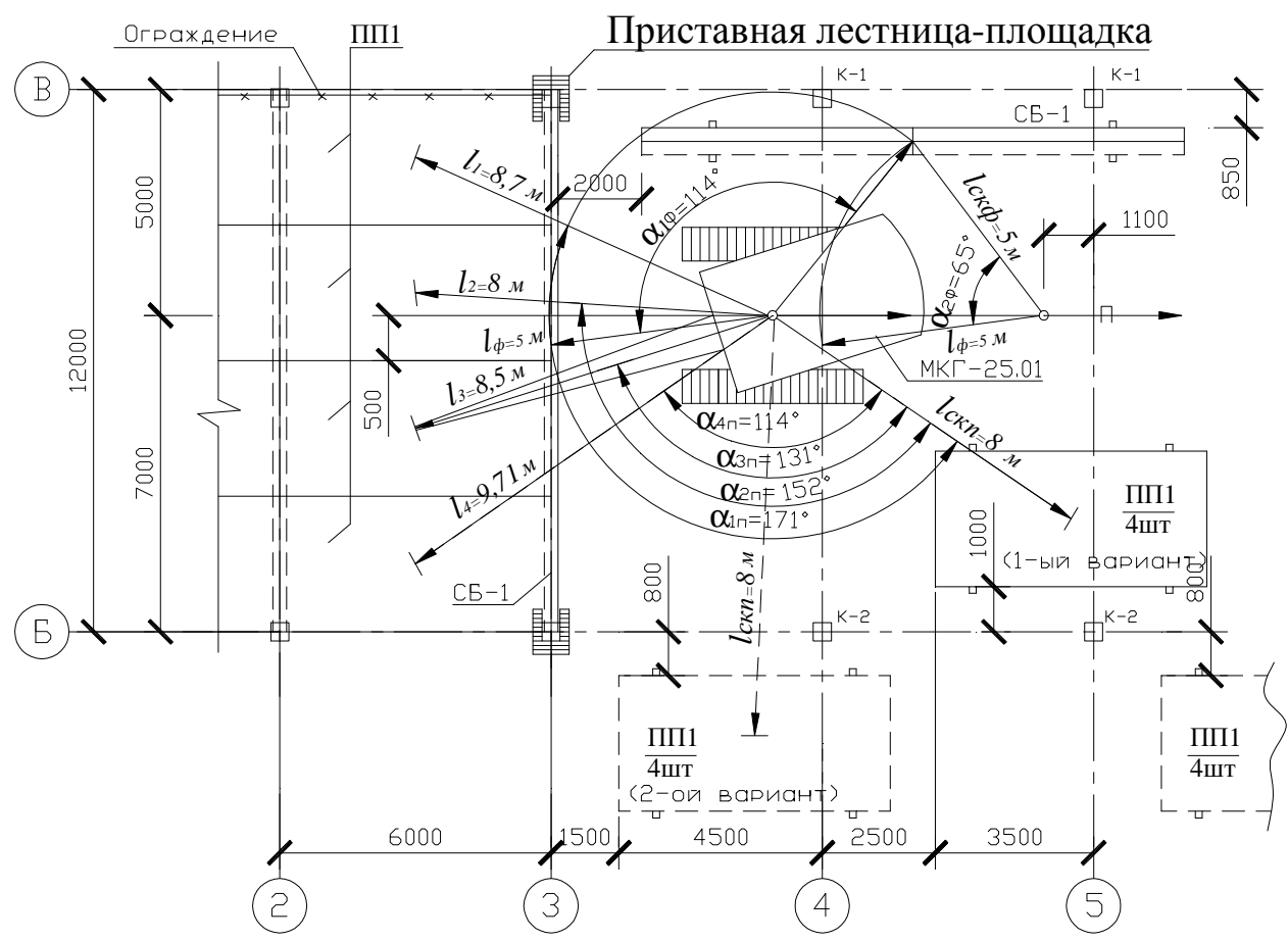
Рисунок 4.4.19 – Схема монтажа конструкций покрытия при пролете 12 м
