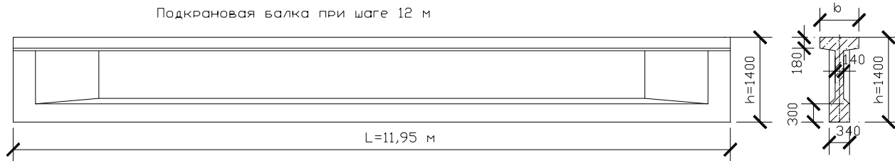
Подкрановая балка при шаге 12 м
