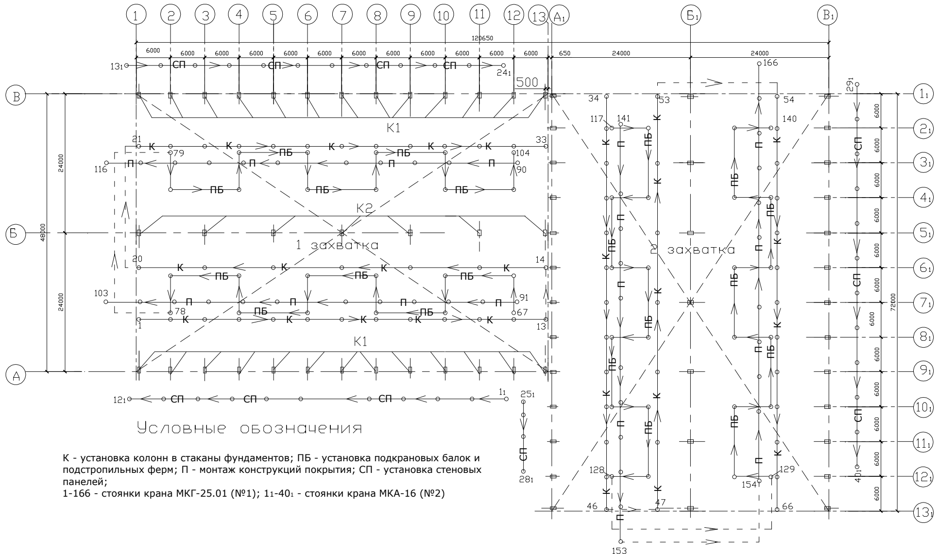
Рисунок 4.5.2 – Схема движения кранов при монтаже конструкций здания
