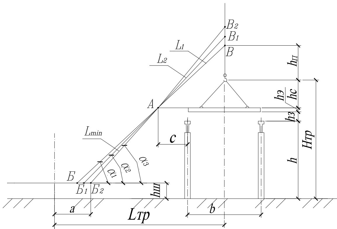
Рисунок 4.4.6 – Схема графического определения H_{тр} , L_{стр} , L_{тр} при монтаже плиты покрытия, располагаемой напротив стоянки крана
