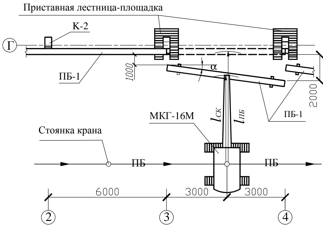
Рисунок 4.4.18 – Схема монтажа подкрановых балок изменением вылета стрелы
