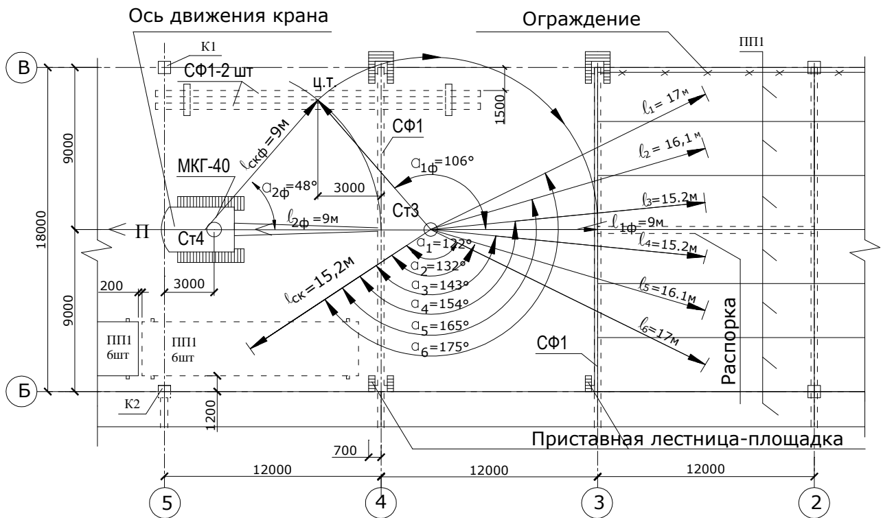
Рисунок 4.4.20 – Схема монтажа конструкций покрытия при пролете 18 м
