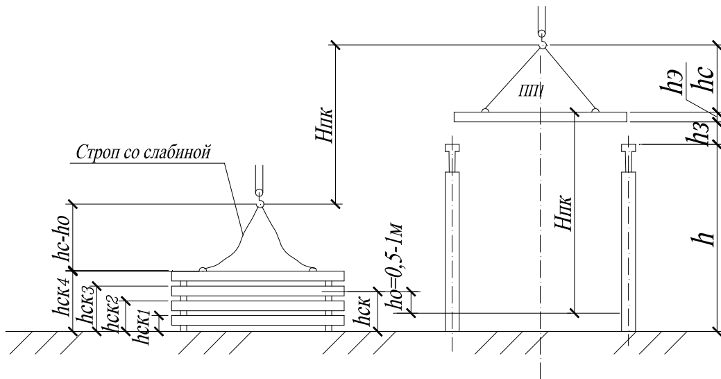
Рисунок 4.4.31 – Схема к определению H_{пк} при складировании элементов в штабеле
