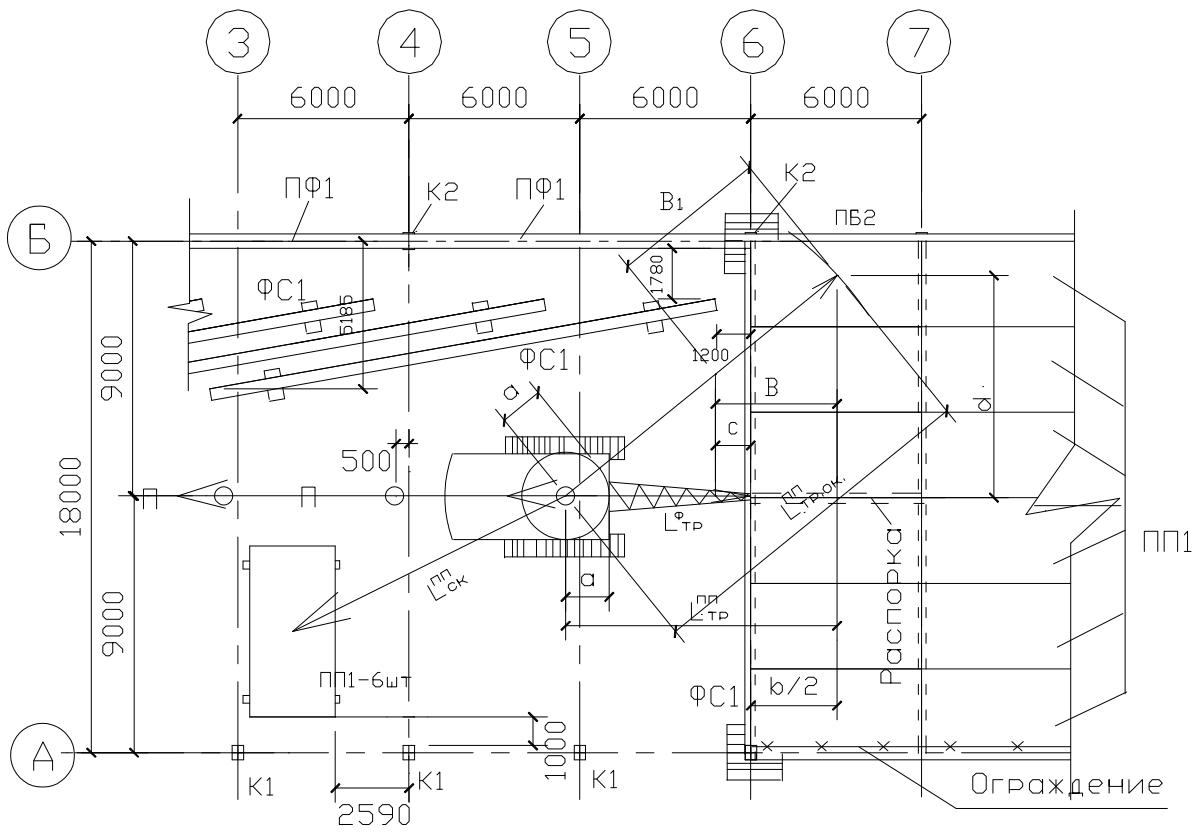
Рисунок 4.4.3 – Схема определения L_{стр} , L_{тр} при монтаже краном всех плит покрытия ячейки с одной стоянки
