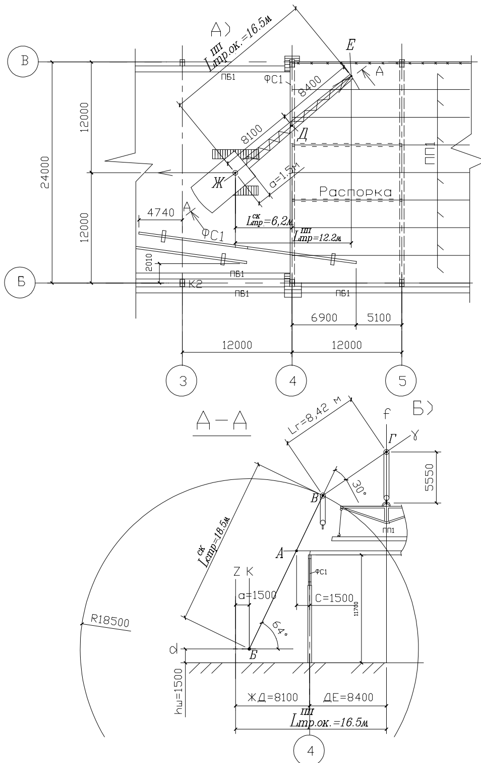
Рисунок 4.4.8 – Схема определения L_{тр.ок}^{nn} , L_z при монтаже гуськом крана всех плит покрытия ячейки с одной стоянки: а – в плане; б – в разрезе «А-А»
