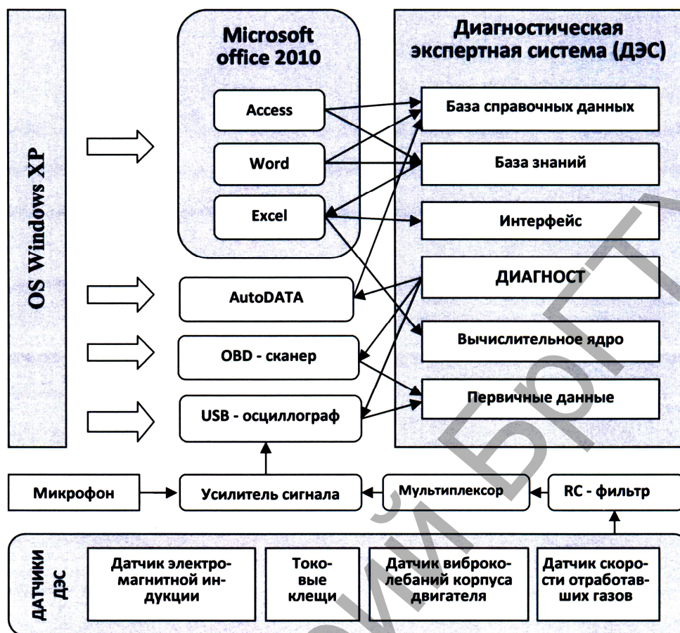
Рис. 1. Состав диагностической системы
