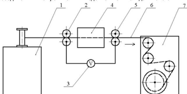
Рис. 5. Устройство для контроля качества протяженных TiNi изделий
