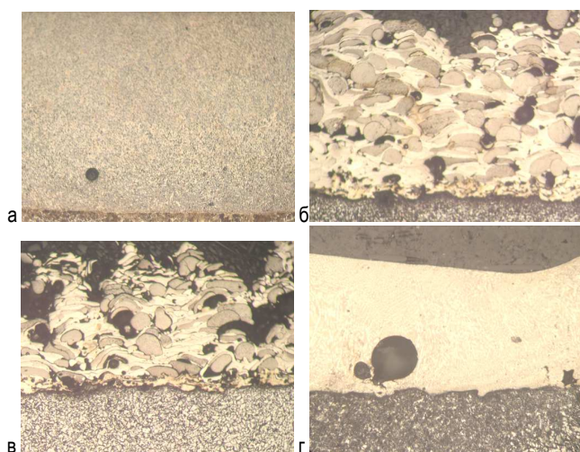
а – без нанougлерода; б – 2%; в – 5%; г – 10% Рисунок 6 – Микроструктура образца ПР-Х4ГСП
