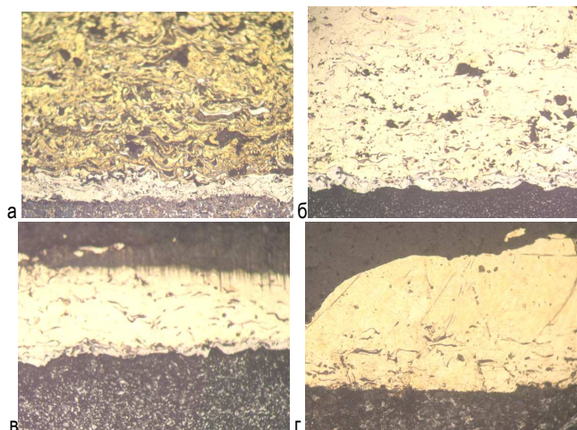
а – без нанougлерода; б – 2%; в – 5%; г – 10% Рисунок 7 – Микроструктура образца ПГ-19М-01
