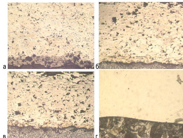
а – без нанougлерода; б – 2%; в – 5%; г – 10% Рисунок 8 – Микроструктура образца ПТ-ЮНХ16СР3
