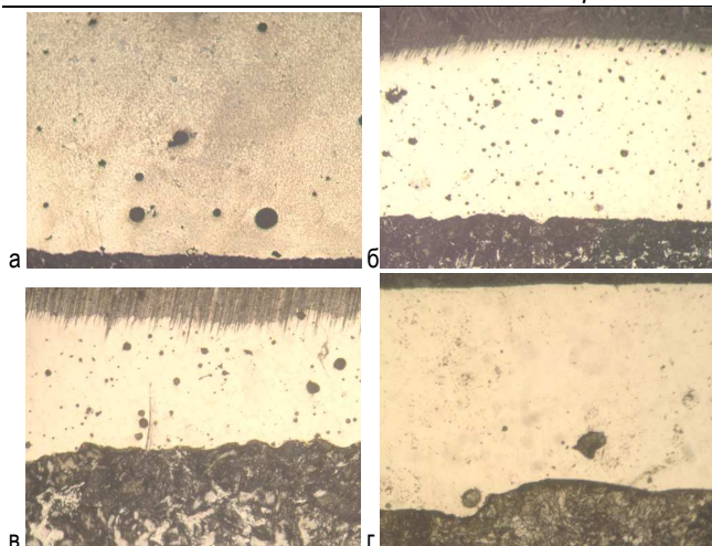
а – без нанougлерода; б – 2%; в – 5%; г – 10% Рисунок 5 – Микроструктура образца ПН-НД-42
