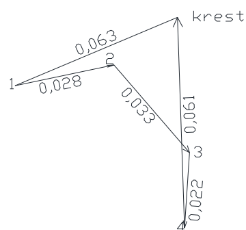
Рисунок 4 – Смещение центров сечения по каждому ярусу колокольни.
