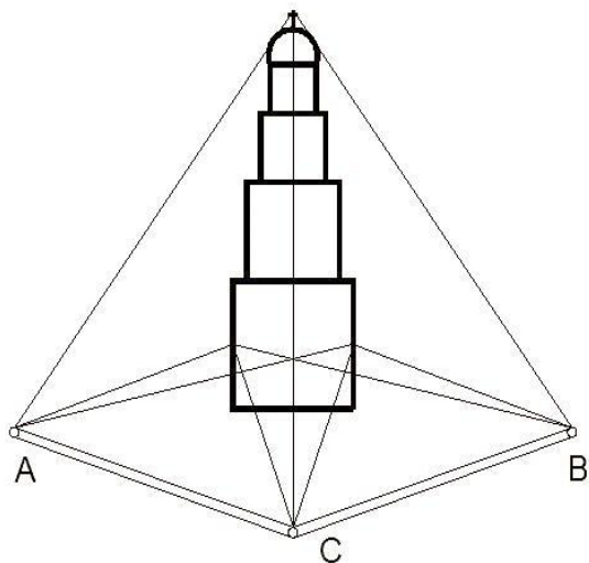
Рисунок 1 – Схема измерений прямой угловой засечкой
