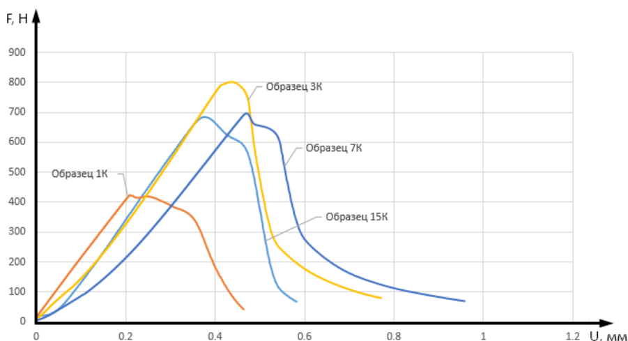
Рисунок 1 – Диаграммы деформирования некоторых образцов ГВЛ при кратковременном действии нагрузки при растяжении в плоскости листа
