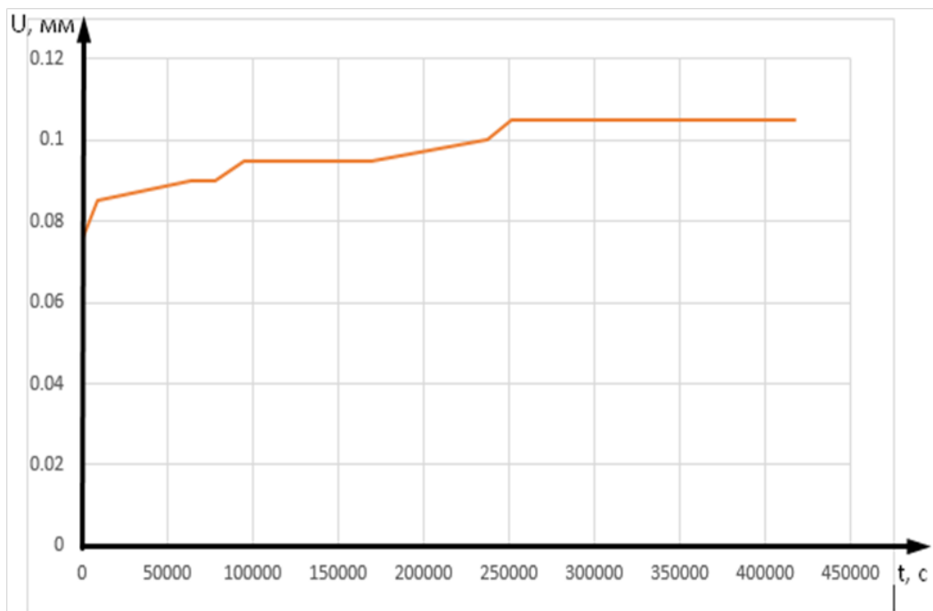
Рисунок 2 - График зависимости деформации от времени для образца № 3 ( \sigma_1=0,9 \cdot f_{t,mean} МПа) (разрушился через 5 дн. 17 ч 55 мин)
