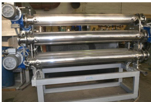
Рисунок5 – Кристаллизатор-охладитель жира перед фасовкой (вотатор)
