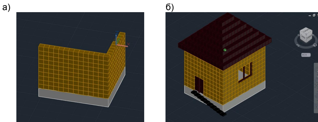
Рисунок 3 – Пример 3D параметрической модели в AutoCAD
