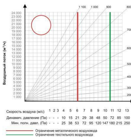
Рисунок 3 – Диаграмма для подбора диаметра воздуховода круглого сечения
