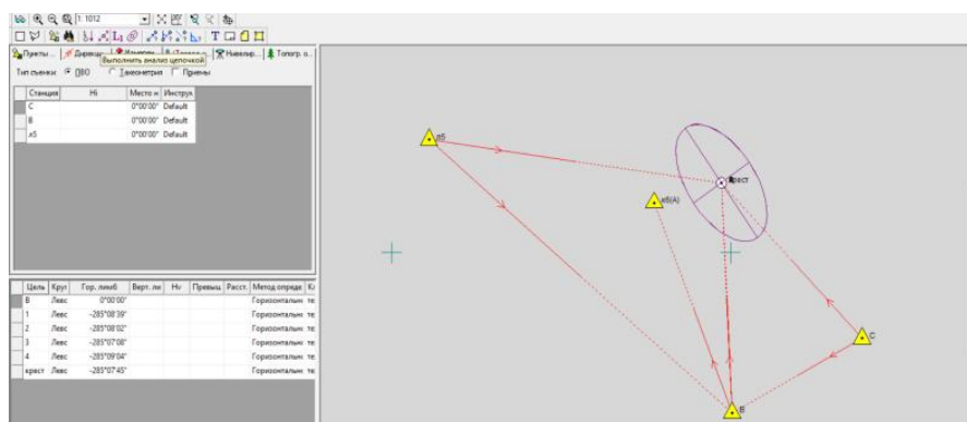
Рисунок 2 – Обработка результатов измерений в программном комплексе CREDO_DAT
