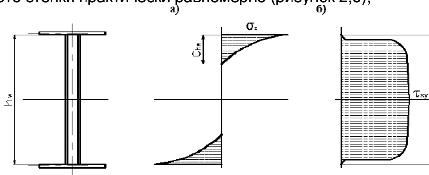
Рисунок 2 – Характер распределения напряжений в сечениях стержней
