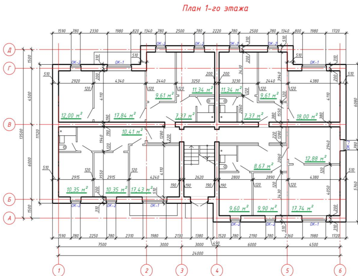
Рисунок 1 – Чертеж плана здания с использованием параметрических объектов
