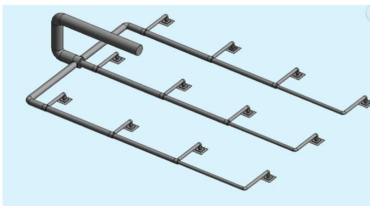
Рисунок 1 – 3D-план системы вентиляции зала заседаний
