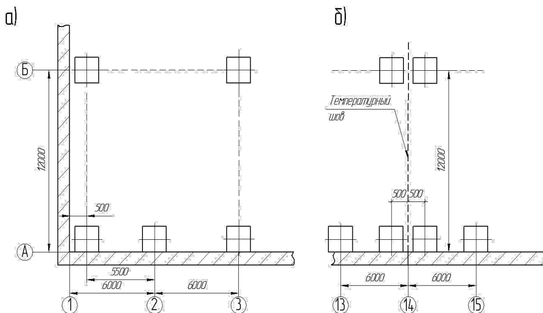
а) привязка колонн в торце здания;
