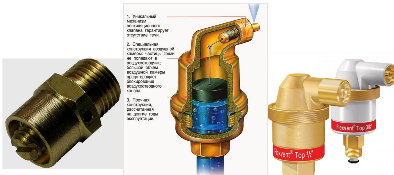
Кран Маевского
