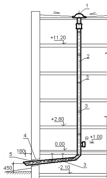
Схема внутреннего водостока:
