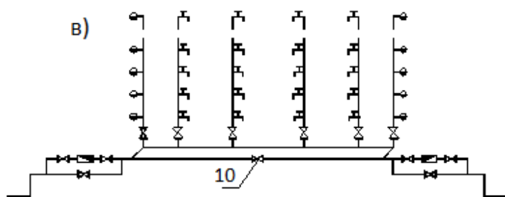
в) схема, закольцованная вводами: 10 – трубопровод, кольцующий вводы.
