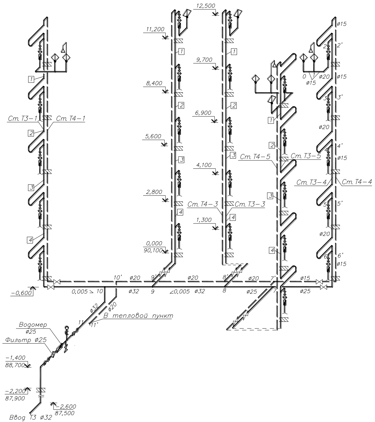
Аксонметрическая схема внутреннего горячего водопровода
