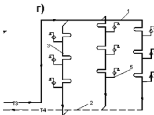
г) схема сетей горячего водопровода с верхней разводкой.
