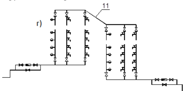
г) схема хозяйственно-противопожарного водопровода с кольцующими перемычками: 11 – кольцующие перемычки.
