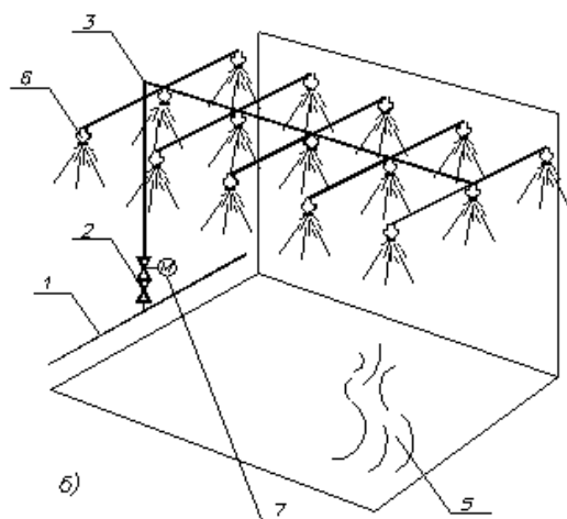
Трубопроводы со спринклерами
