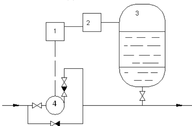
Установка переменного давления
