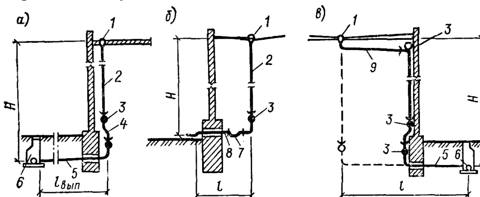
Схемы внутренних водостоков перпендикулярные (а, б, в)
