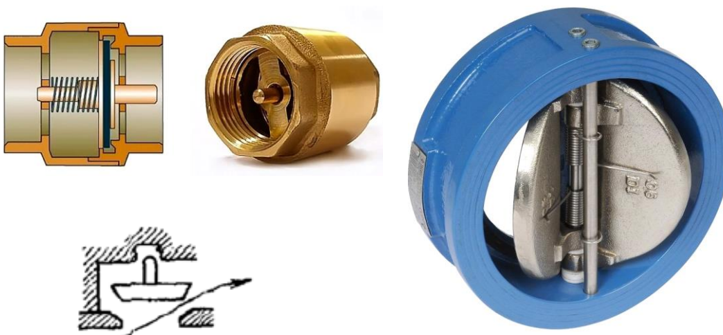
Принципиальная схема действия обратного клапана
