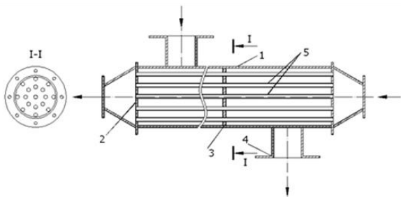
Трубчатый противоточный водонагреватель
