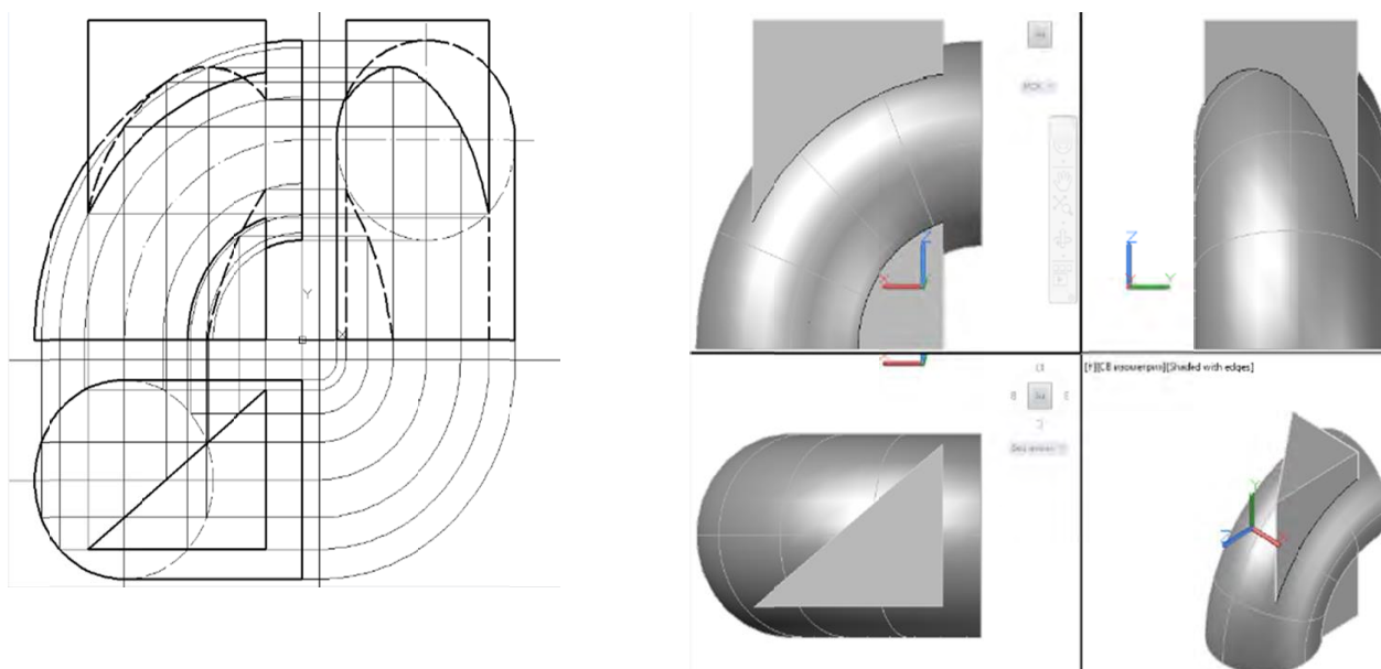
Рис. 9. Построение трех проекций и аксонометрии комбинированного тела (тора, треугольной призмы) средствами 3D-моделирования и создания реалистичных изображений
