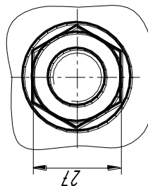
Болтовое соединение
