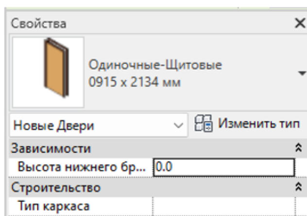
Рис. 3.29. Типоразмер двери
