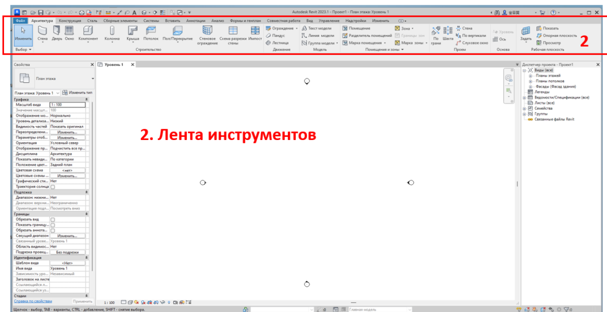
Рис. 2.13 Лента инструментов
