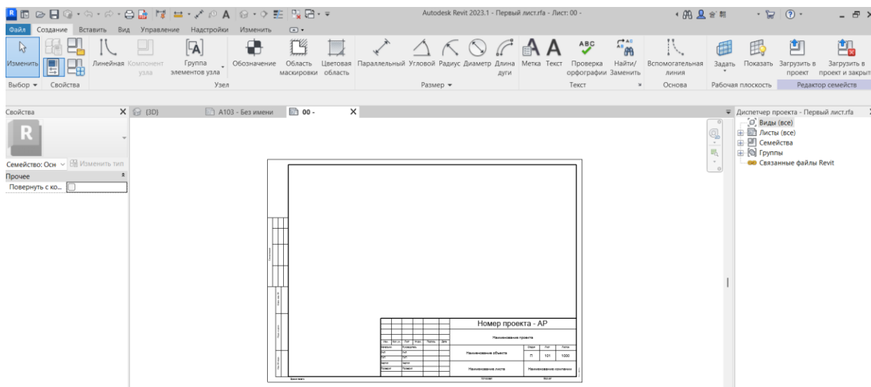
Рис. 5.3 Редактор семейств
