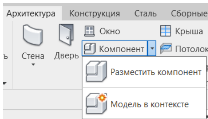
Рис. 4.19 Вкладка «Компонент»
