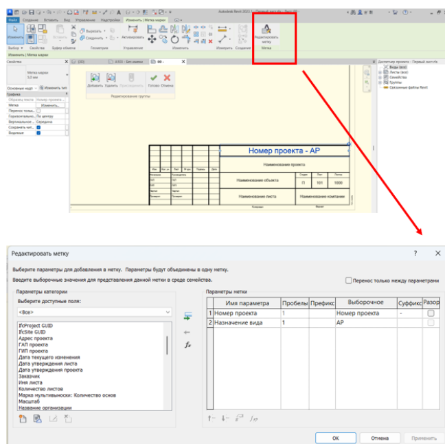
Рис.5.4 Редактирование метки
