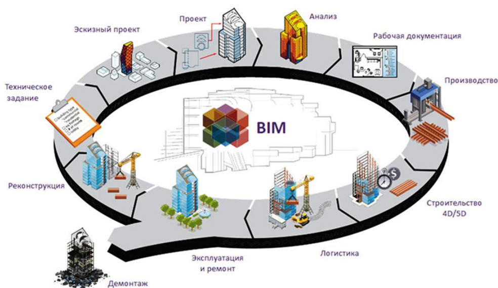
Рис. 1.1 Информационная модель
