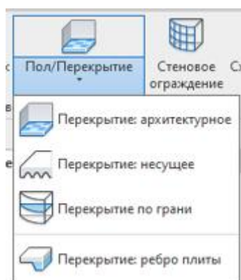
Рис. 3.23. Инструмент «Перекрытие»
