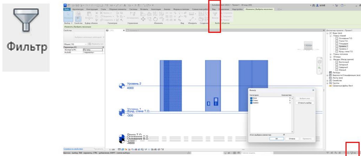
Рис. 2.32 Инструмент Фильтр
