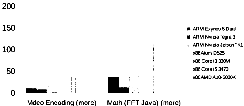
Мал. 2. Параўнанне архітэктур на рэальных задачах (сямейства x86 адзначана штыроўкай; найбольш высокія значэнні адпавядаюць большай прадукцыйнасці)
