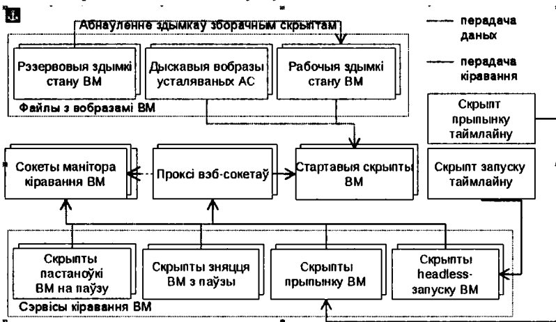
Малюнак 2. Архітэктара сістэмы
