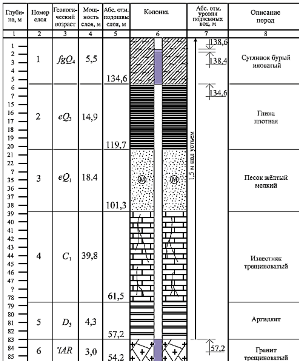
Рисунок 2 – Пример геологической колонки буровой скважины
