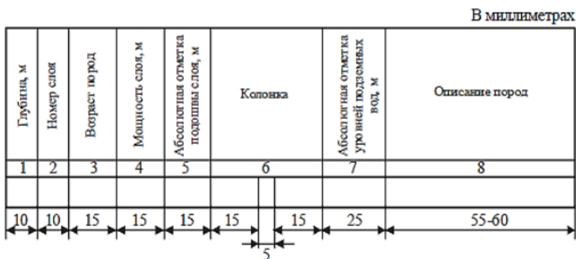
Рисунок 1 – Габаритные размеры геологической колонки буровой скважины
